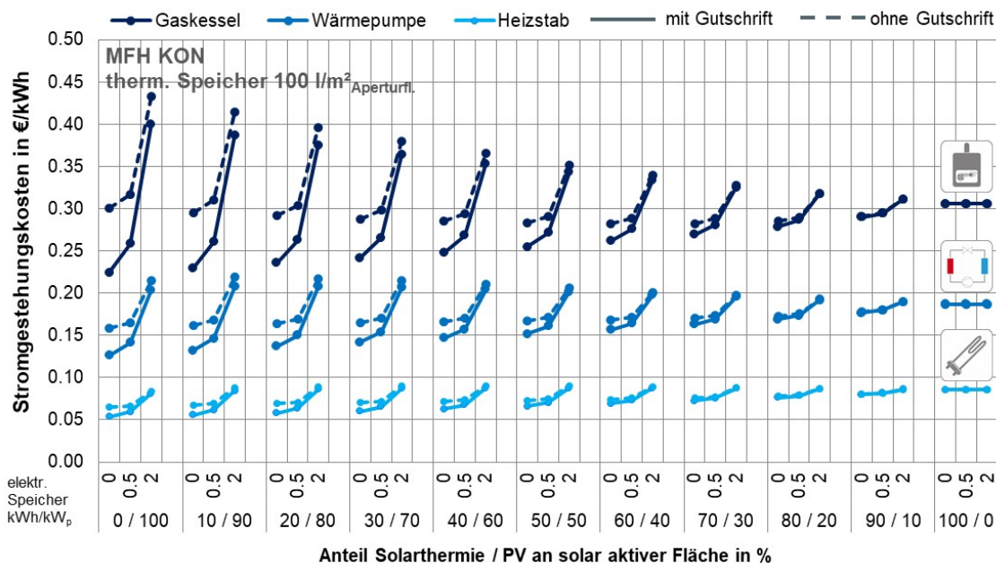
Abbildung 7-37: MFH KON: Gestehungskosten Strom in Abhängigkeit der Konzeptvariante
