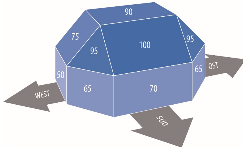
Abbildung A. 22: Prozentual maximal zu erzielende PV-Erträge in abhängig der Modulausrichtung
