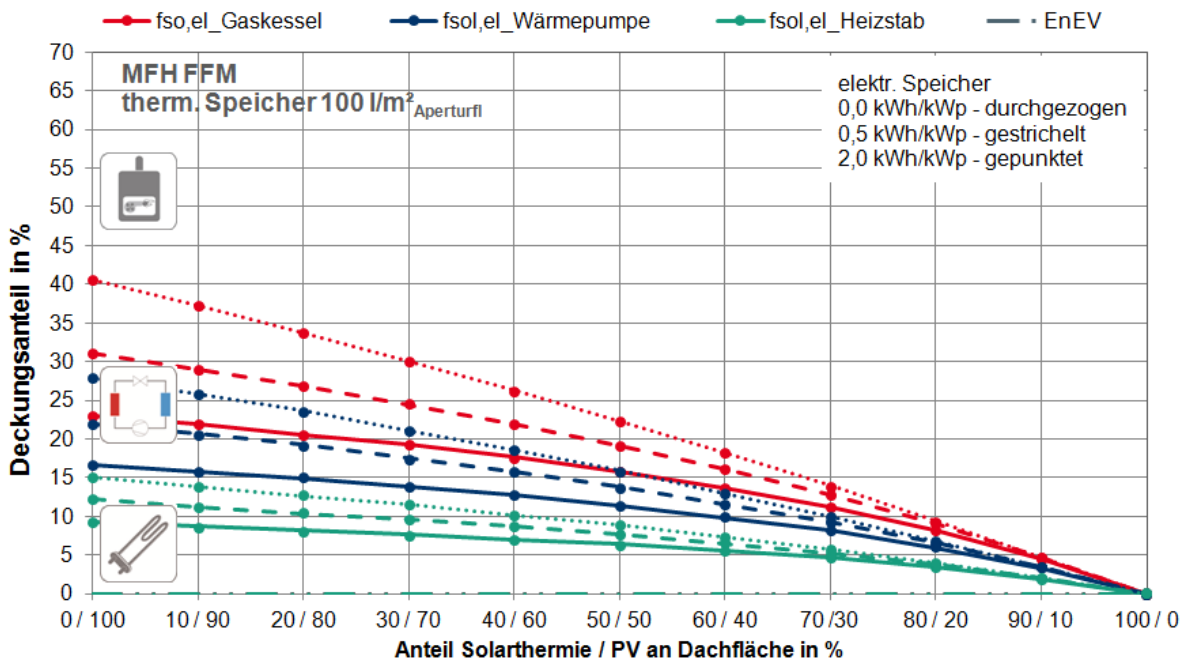
Abbildung G. 11: MFH FFM: Solar elektrische Deckungsanteile f_{sol,el} am jährlichen Stromverbrauch in Abhängigkeit der Konzeptvariante
