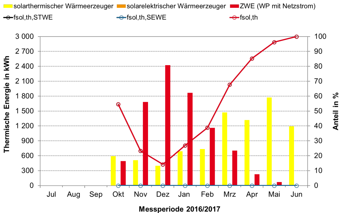
Abbildung 6-28: Monatliche Wärmeerzeugung nach Wärmequellen sowie die solarthermischen Deckungsanteile für den Messzeitraum 2016/2017 des Gebäudes in Döhlau
