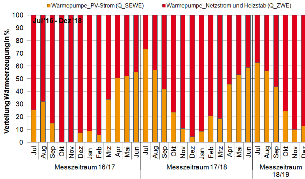
Abbildung 6-19: MFH FFM: Monatliche Deckungsanteile der Wärmeerzeugung
