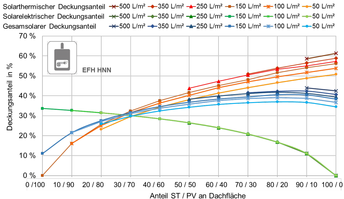
Abbildung 5-5: Solare Deckungsanteile für das EFH in HNN in Abhängigkeit der thermischen Speichergröße, Variante mit Gasbrennwertgerät
