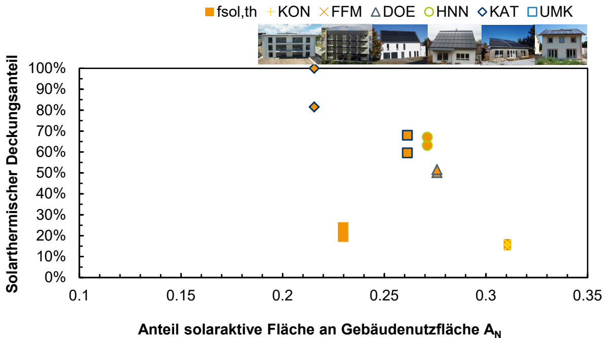
Abbildung 7-5: Solarthermischer Deckungsanteil f_{sol,th} in den messtechnisch untersuchten Gebäuden, Messzeitraum 16/17 und 17/18
