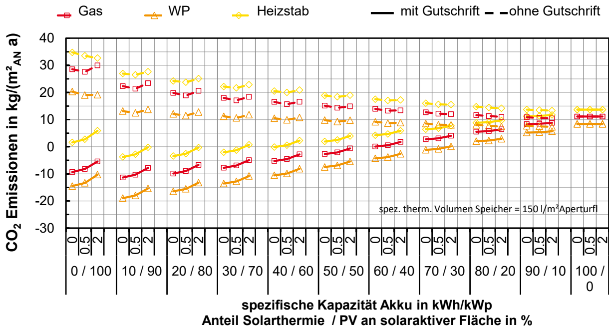
Abbildung G. 30: EFHKAT: spez. CO 2 -Emissionen in Abhängigkeit der Konzeptvariante bezogen auf den Lebenszyklus
