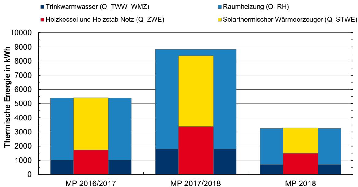
Abbildung 6-59: Jährliche Messdaten für die Wärmeversorgung aus messtechnisch untersuchten Zeiträumen
