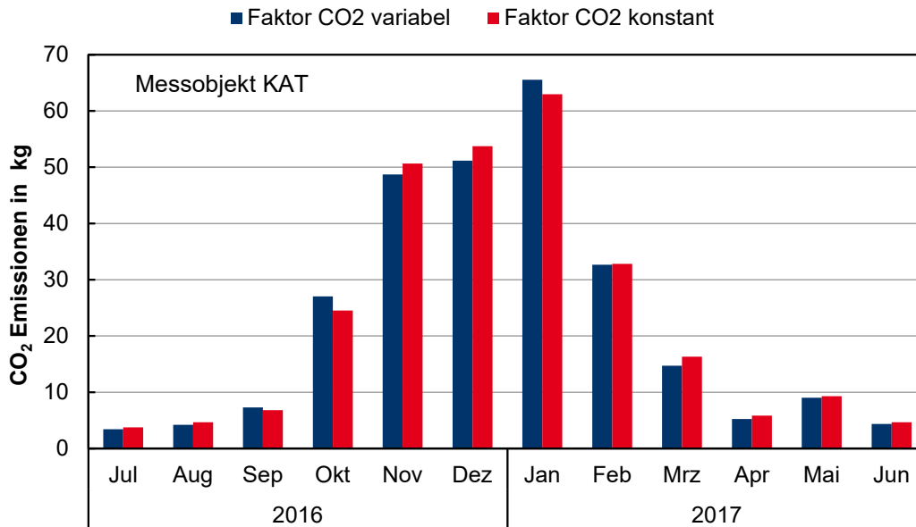
Abbildung 7-22: An den Bezug von elektrischer Energie gebundene CO 2 Emissionen für das EFH KAT in dem Zeitraum 01.07.2016 – 30.06.2017 basierend auf stündlich aufgelösten Daten
