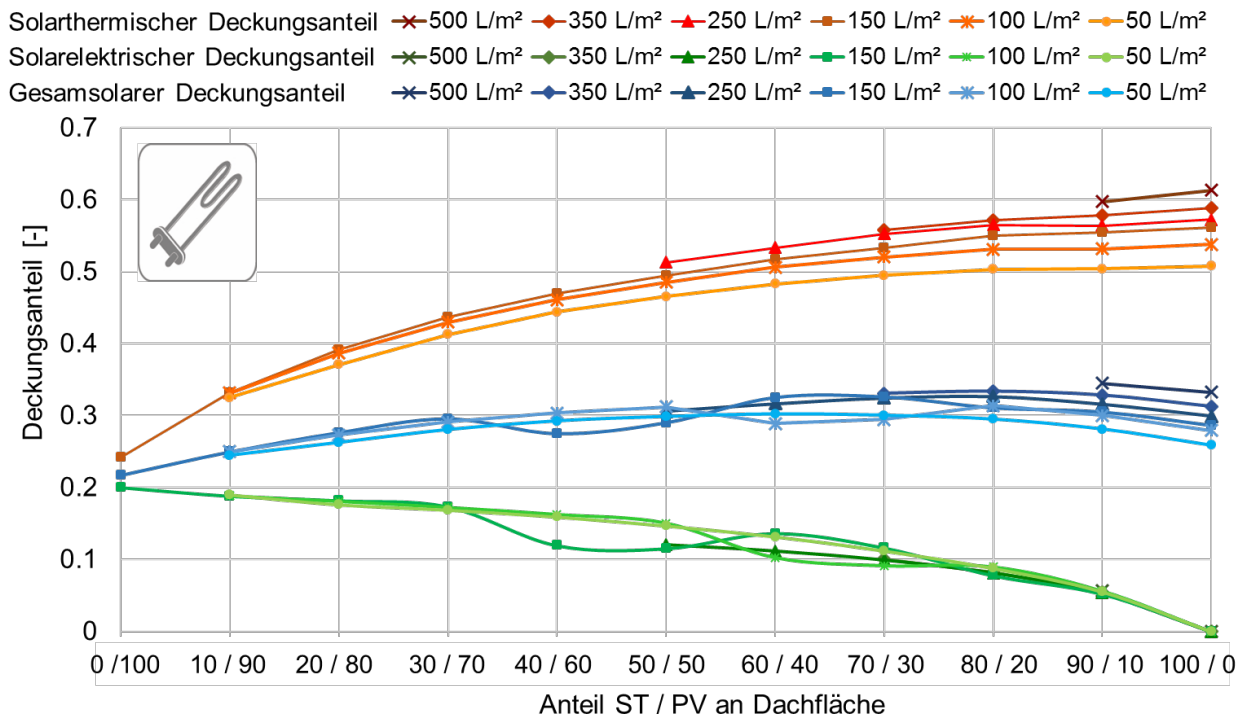
Abbildung G. 5: Solare Deckungsanteile für das EFH in HNN in Abhängigkeit der thermischen Speichergröße, Variante mit Heizstab
