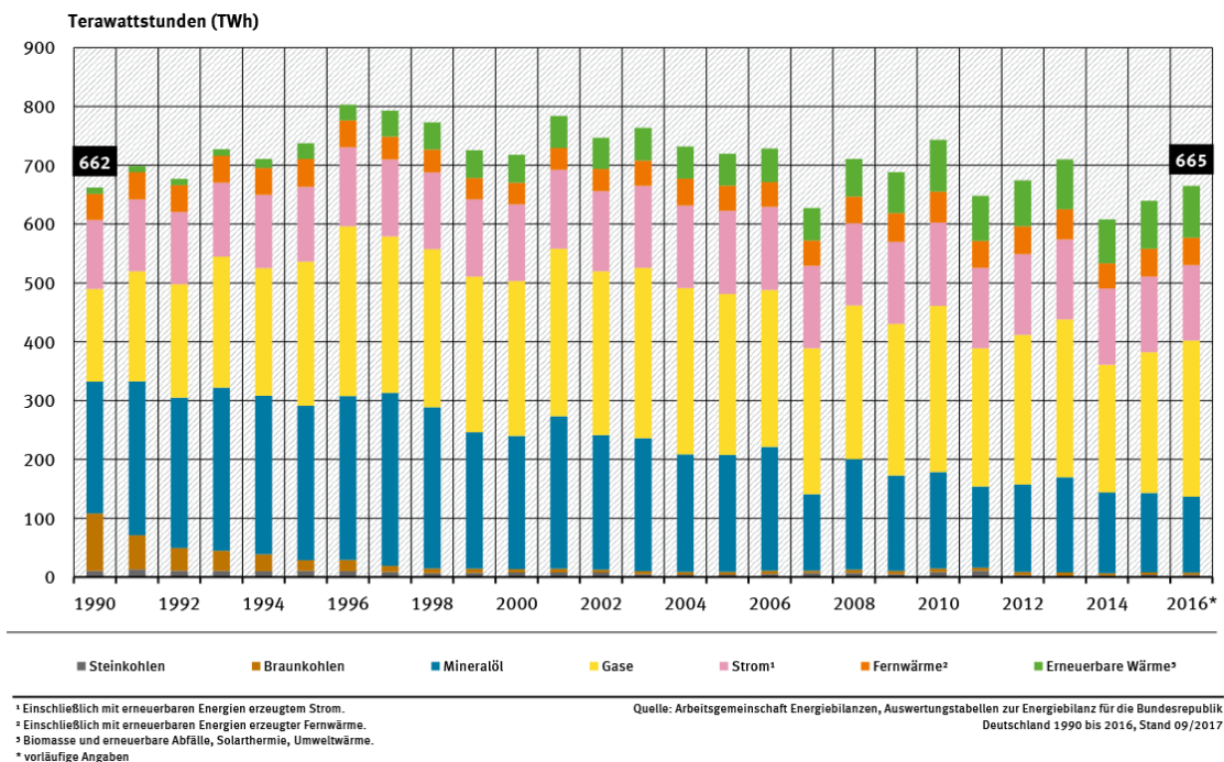
Abbildung 3-2: Entwicklung des Endenergieverbrauchs der privaten Haushalte in Deutschland in den Jahren 1990 bis 2016 [UBA]
