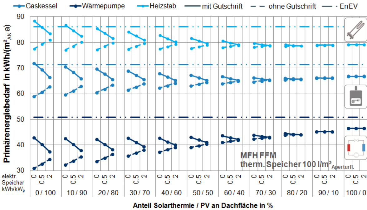
Abbildung G. 34: MFH FFM: spez. Primärenergiebedarf in Abhängigkeit der Konzeptvariante während des Betriebes
