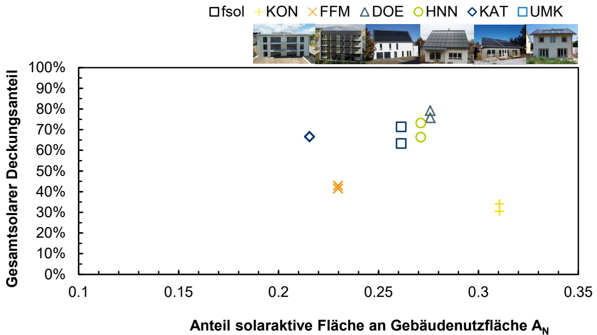
Abbildung 7-7: Gesamtsolarer Deckungsanteil in den messtechnisch untersuchten Gebäuden, Messzeitraum 16/17 und 17/18
