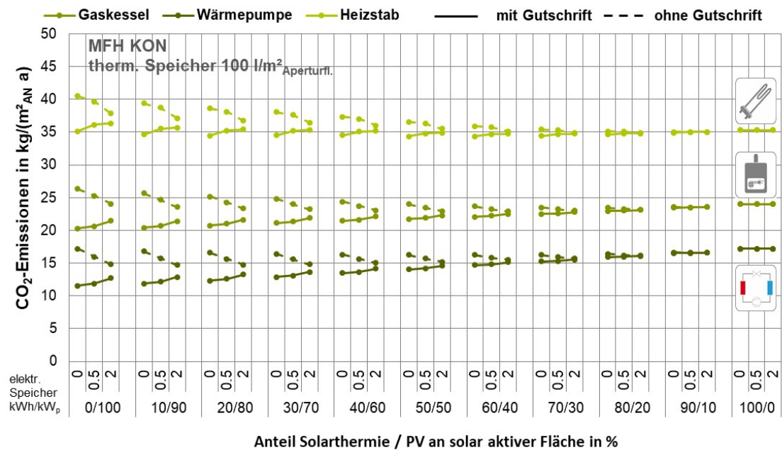
Abbildung 7-31: Vergleich der CO 2 -Emissionen des EFH UMK und des MFH KON ohne und mit Gutschrift für eingespeisten Strom
