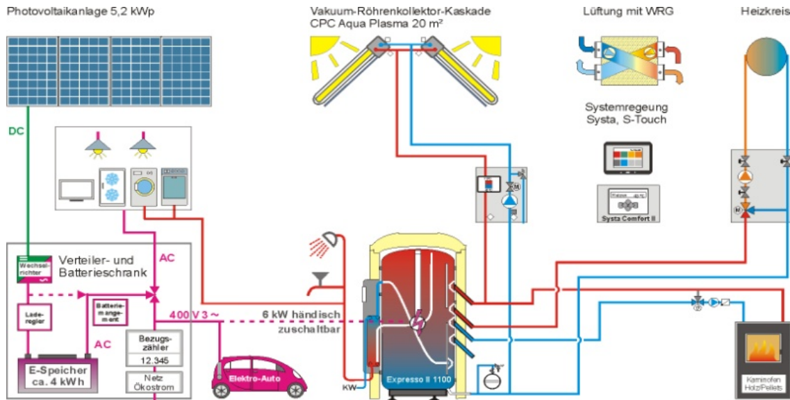
Abbildung 6-54: Energiekonzept des Gebäudes UMK
