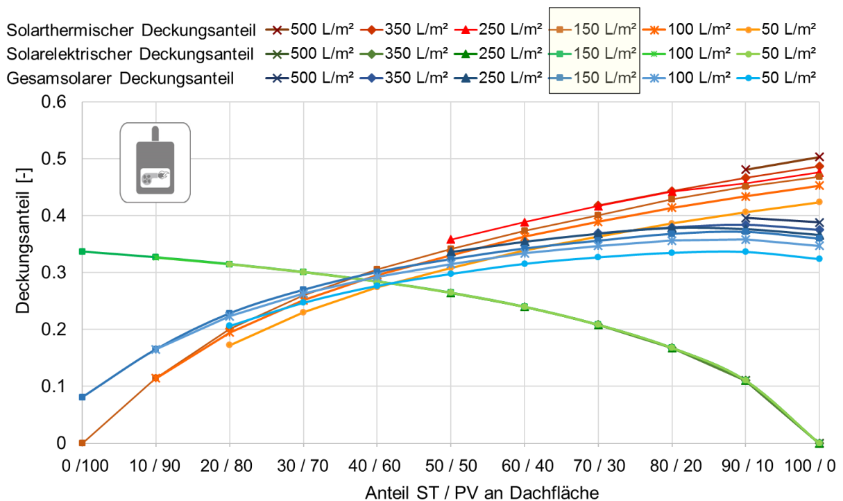
Abbildung 4-2: Einfluss des Verhältnisses von thermischer Speichergöße zur Aperturfläche auf den solaren Deckungsanteil beim EFH
