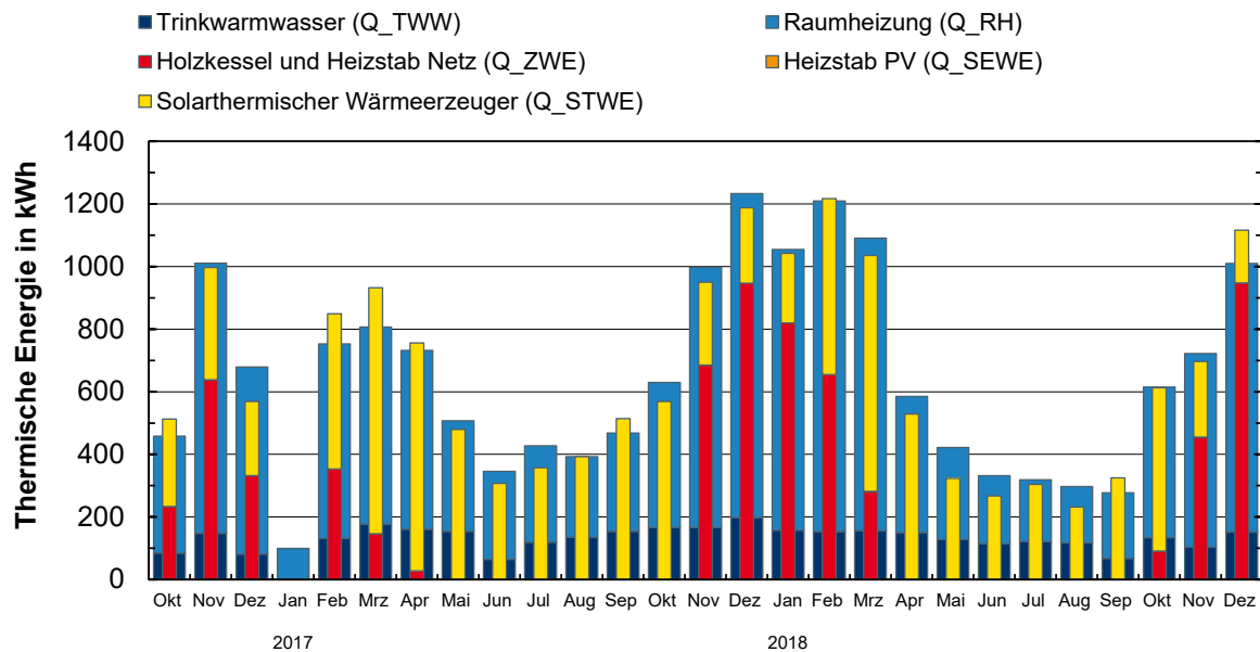
Abbildung 6-58: Monatliche Messdaten für die Wärmeversorgung aus dem gesamten messtechnisch untersuchten Zeitraum
