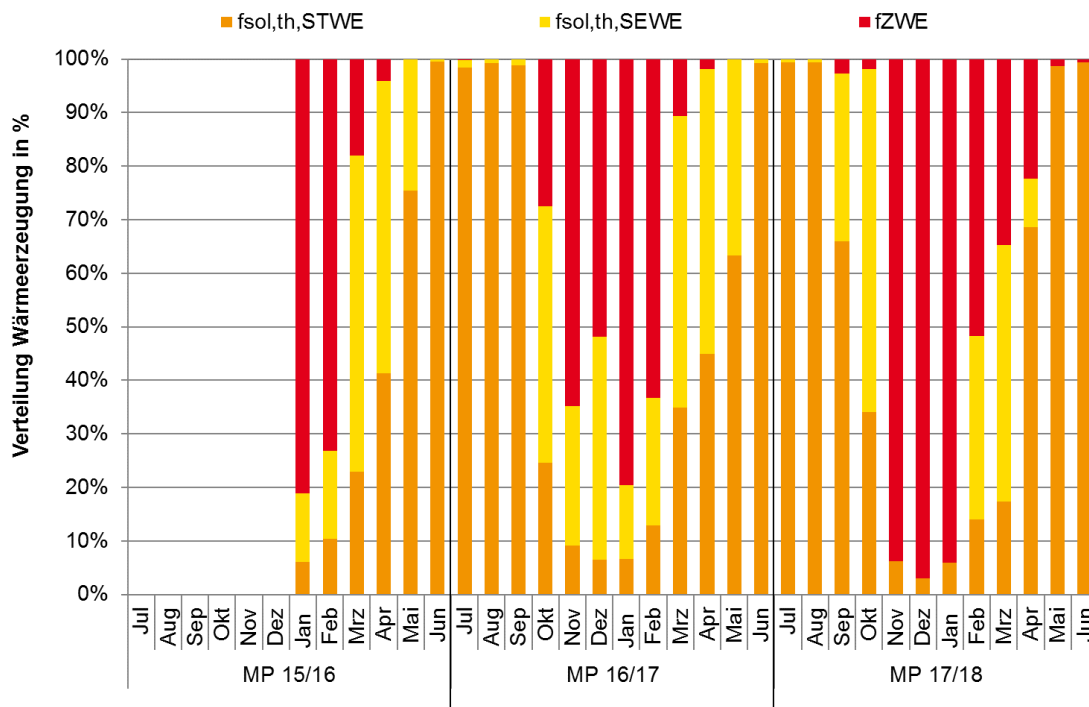
Abbildung 6-39: Anteile der monatlichen Wärmeerzeugung nach Wärmequellen für den Messzeitraum 2016/2017 und 2017/2018 des Gebäudes in Heilbronn-Neckargartach
