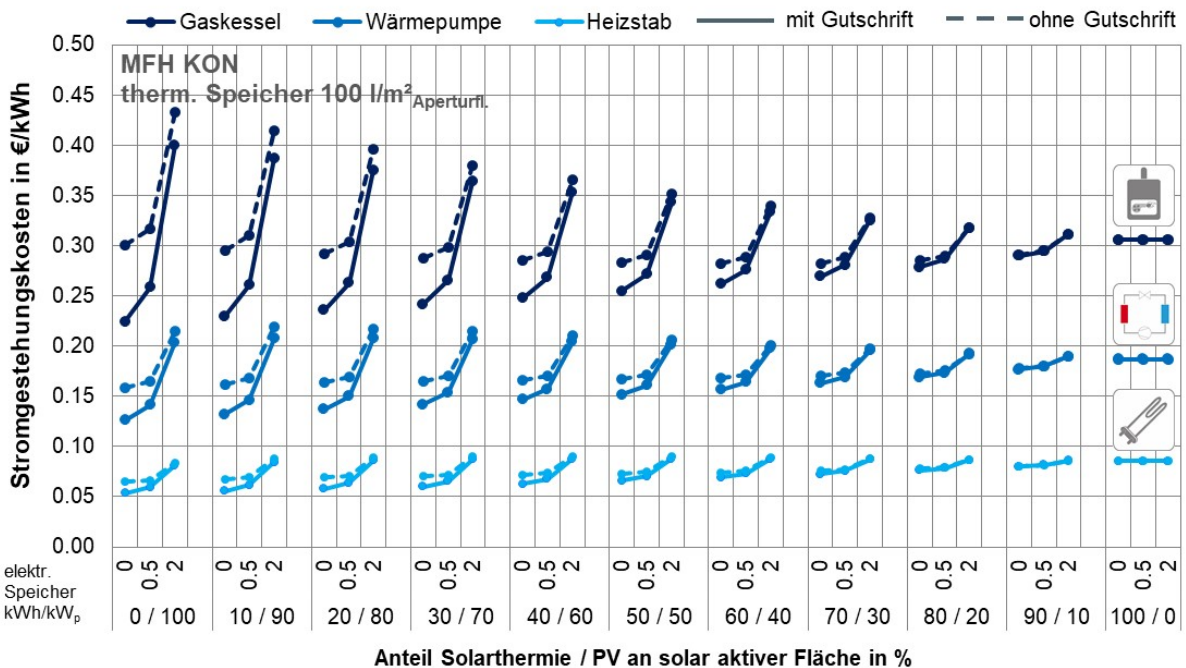
Abbildung G. 50: MFH KON: Gestehungskosten Strom in Abhängigkeit der Konzeptvariante
