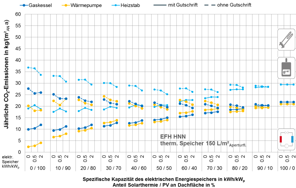
Abbildung G. 28: EFH HNN: spez. CO 2 -Emissionen in Abhängigkeit der Konzeptvariante bezogen auf ein Jahr über den gesamten Lebenszyklus von 20 Jahren
