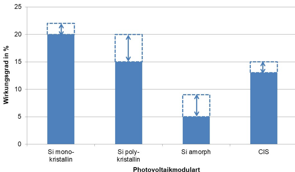
Abbildung A. 2: Modulwirkungsgrade bei Verwendung unterschiedlicher Solarzellen (Wafer)
