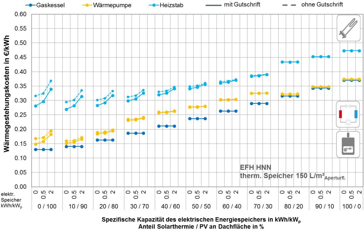
Abbildung G. 55: EFH HNN: Gestehungskosten Wärme in Abhängigkeit der Konzeptvariante
