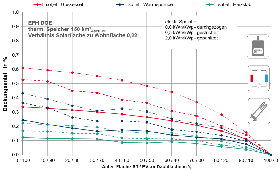
Abbildung G. 17: EFH DOE: Solar elektrische Deckungsanteile f_{sol,el} am jährlichen Stromverbrauch in Abhängigkeit der Konzeptvariante
