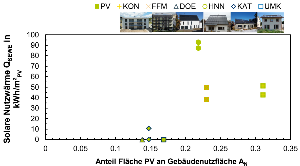
Abbildung 7-11: Spezifische Erträge der solarelektrischen Wärmeerzeuger Q_{SEWE} über dem Anteil der Bruttomodulfläche an der Gebäudenutzfläche A_N , Messzeitraum 16/17 und 17/18
