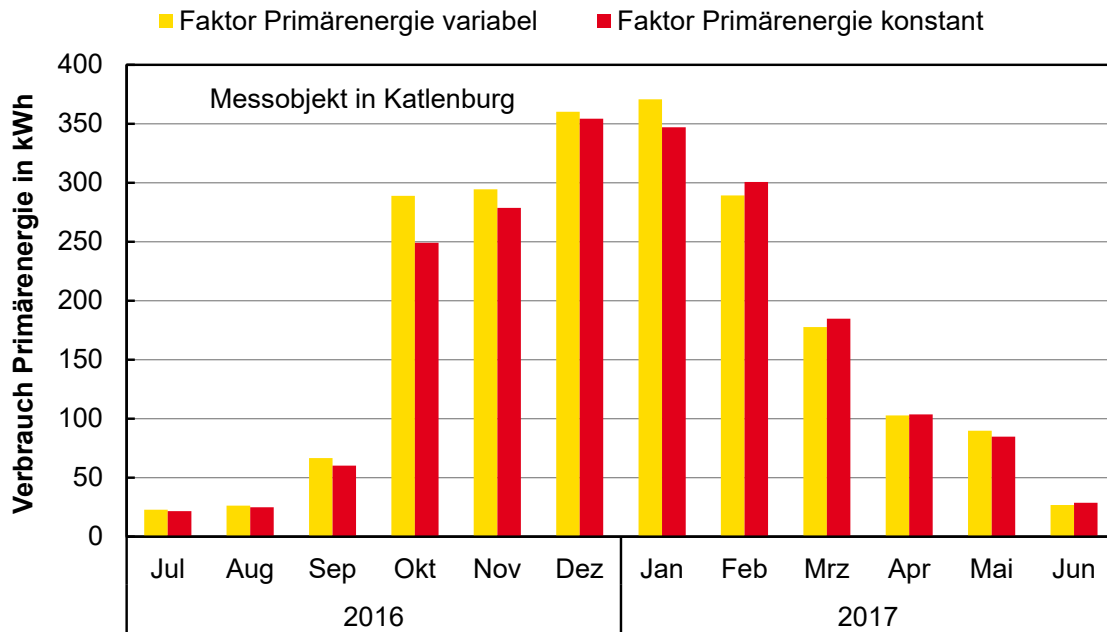
Abbildung 7-18: Verbrauch an Primärenergie für die elektrische Energieversorgung für das EFH KAT in dem Zeitraum 01.07.2016 – 30.06.2017 basierend auf stündlich aufgelösten Daten
