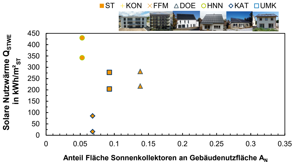
Abbildung 7-10: Spezifische Erträge der solarthermischen Wärmeerzeuger Q_{STWE} über dem Anteil der Bruttokollektorfläche an der Gebäudenutzfläche A_N , Messzeitraum 16/17 und 17/18
