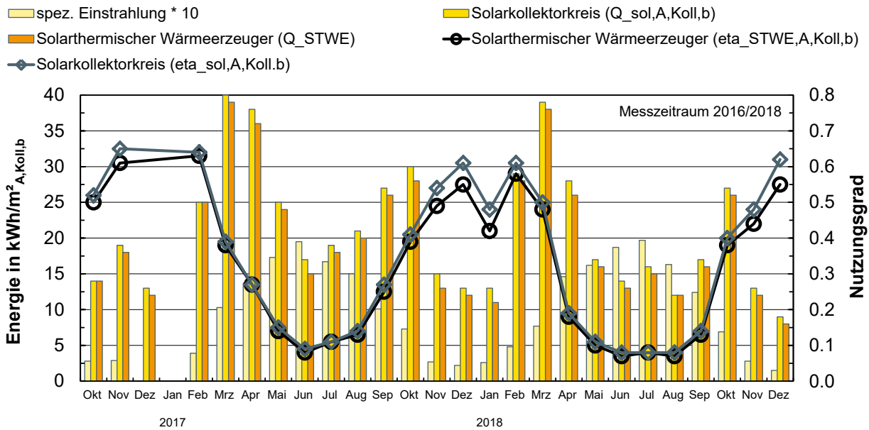
Abbildung 6-55: Aperturflächenspezifische Einstrahlung sowie die im Kollektorkreis erzeugte Wärme bezüglich dem tatsächlich nutzbaren solarthermischen Ertrag und den daraus resultierenden Nutzungsgraden für den Kollektorkreis und den solarthermischen Wärmeerzeuger.
