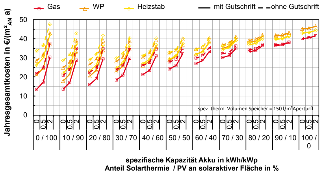
Abbildung 7-34: EFH UMK: spez. Jahresgesamtkosten in Abhängigkeit der Konzeptvariante
