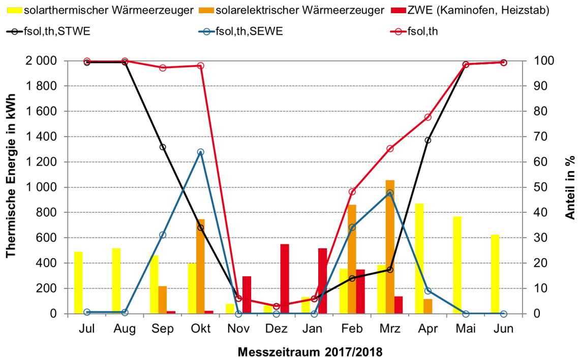
Abbildung 6-38: Monatliche Wärmeerzeugung nach Wärmequellen sowie die solarthermischen Deckungsanteile für den Messzeitraum 2017/2018 des Gebäudes in Heilbronn-Neckargartach
