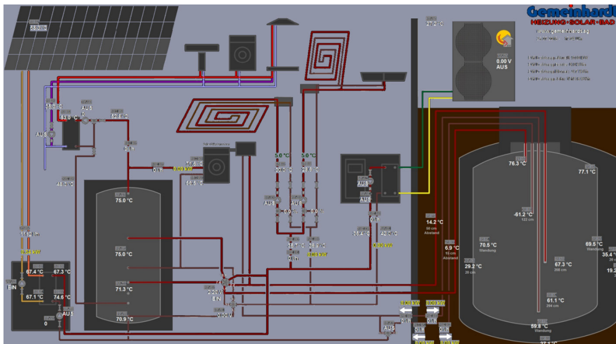
Abbildung 6-25: Energiekonzept des Gebäudes in Döhlau
