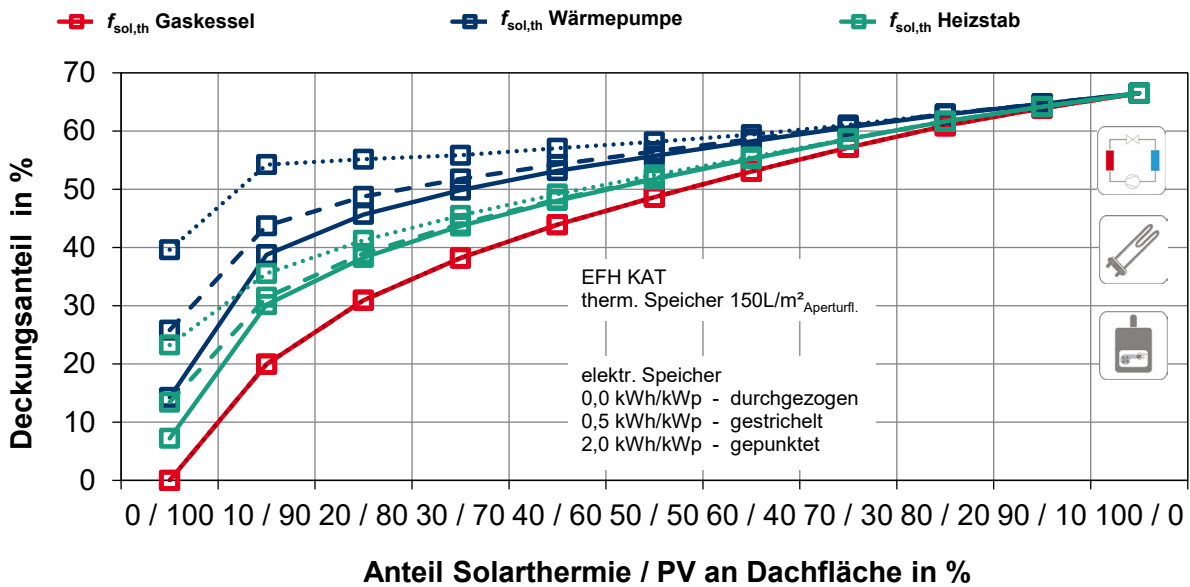
Abbildung G. 19: EFH KAT: Solar thermische Deckungsanteile f_{sol,th} an der Wärmebereitstellung in Abhängigkeit der Konzeptvariante
