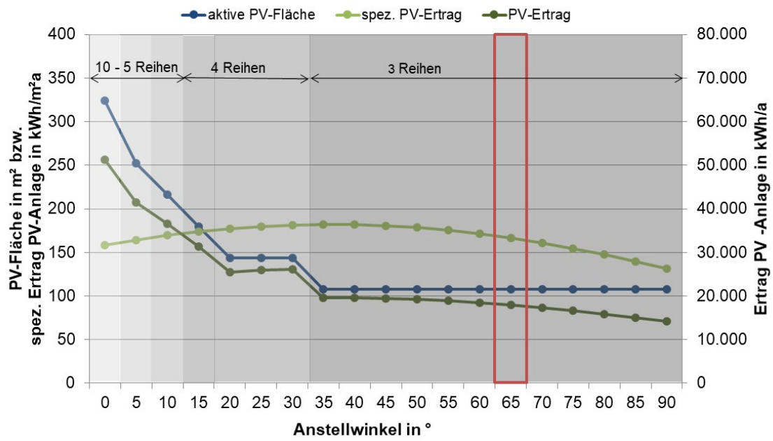
Abbildung 5-8: Mögliche PV-Fläche, spez. und absoluter Ertrag der PV-Anlage in Abhängigkeit des Anstellwinkels der PV-Module
