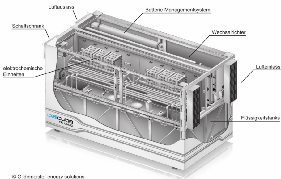
Abbildung A. 21: Schematische Darstellung des Aufbaus einer Vanadium-Redox-Flow-Batterie mit Nebenaggregaten [Gildemeister]
