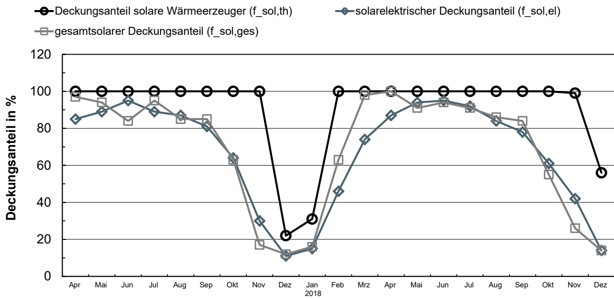
Abbildung 6-51: EFH KAT: Monatliche solare Deckungsanteile
