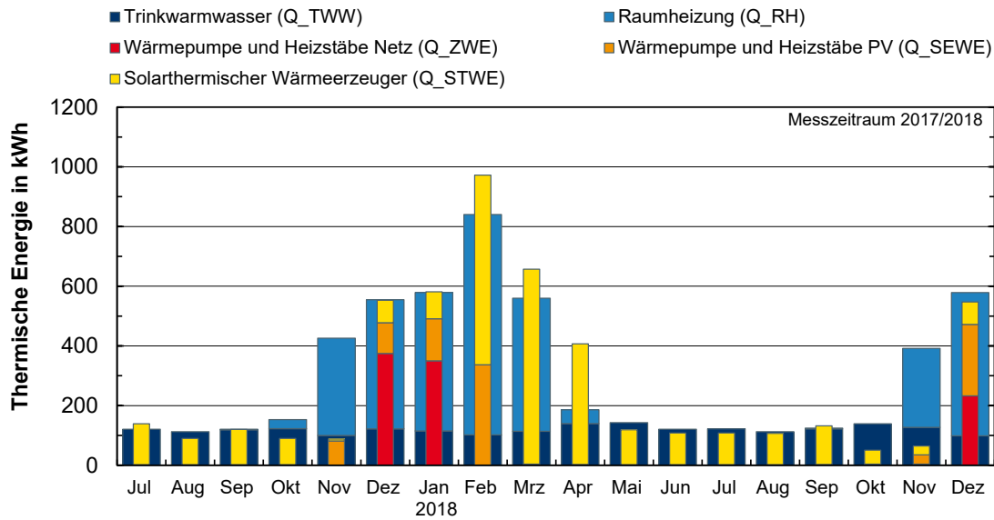
Abbildung 6-47: Monatliche Messdaten für die Wärmeversorgung aus dem gesamten messtechnisch untersuchten Zeitraum
