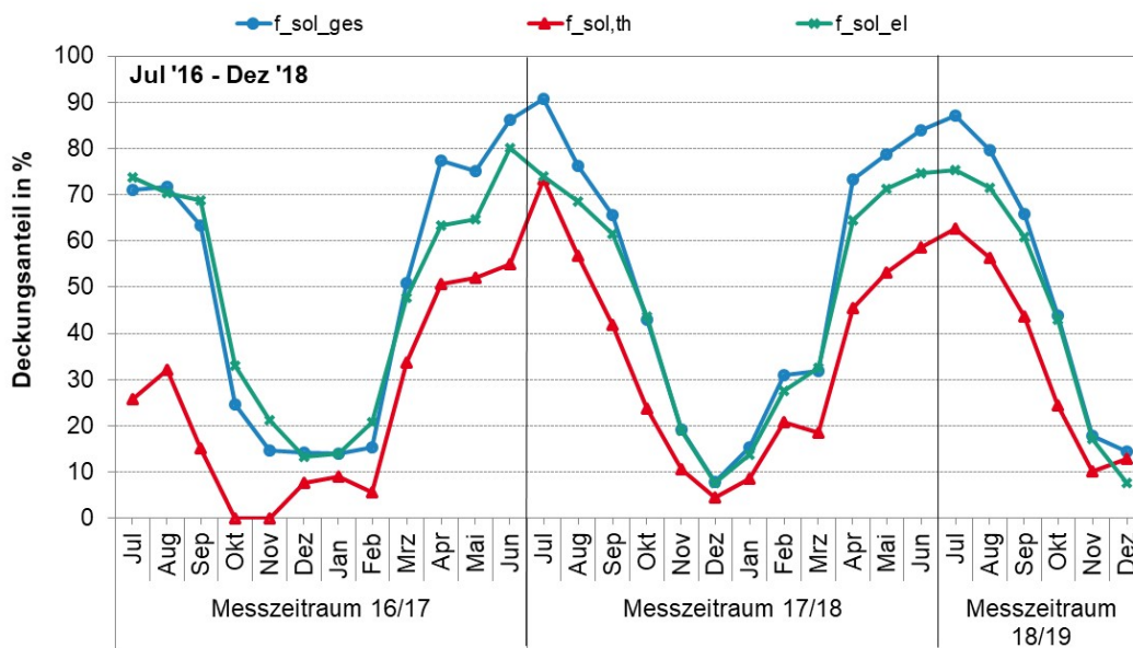
Abbildung 6-23: MFH FFM: Monatliche solare Deckungsanteile
