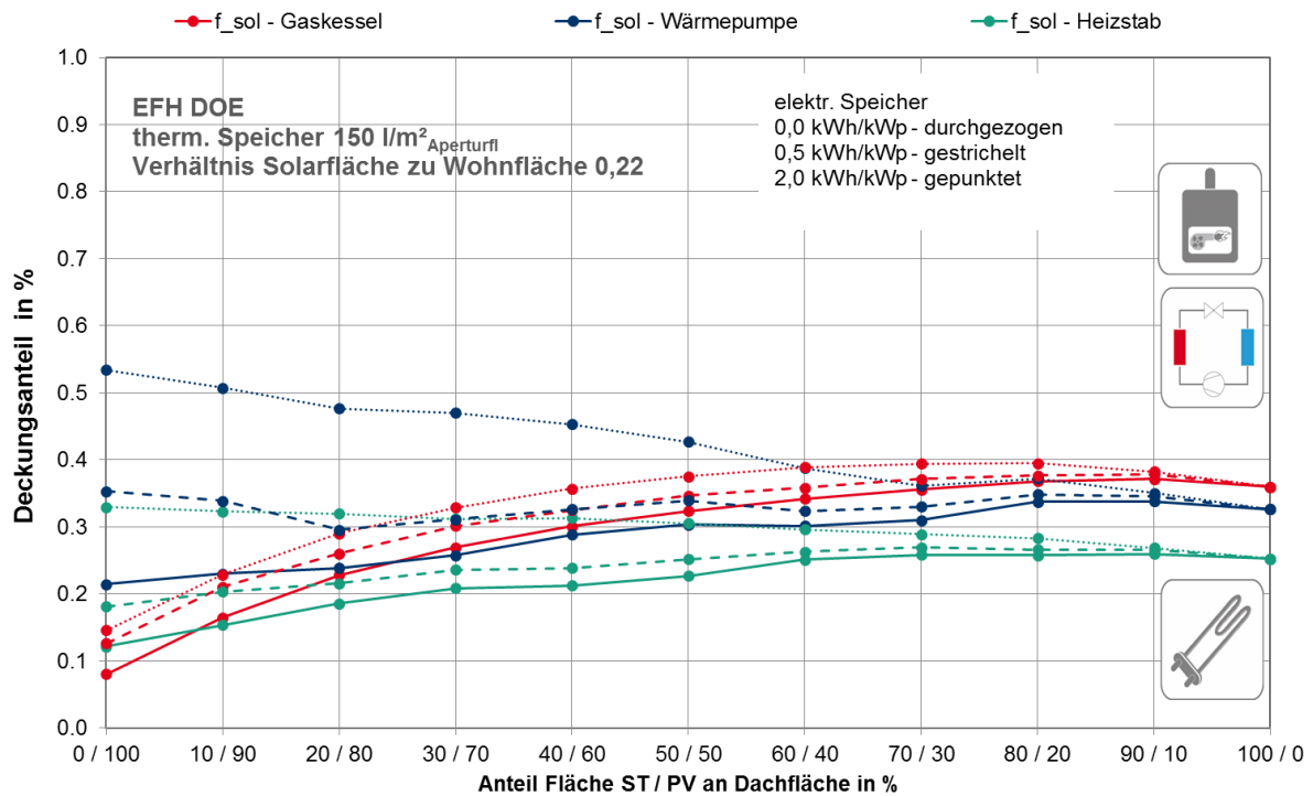
Abbildung G. 15: EFH DOE: Gesamt solarer Deckungsanteile: f_{sol} am jährlichen Energieverbrauch in Abhängigkeit der Konzeptvariante
