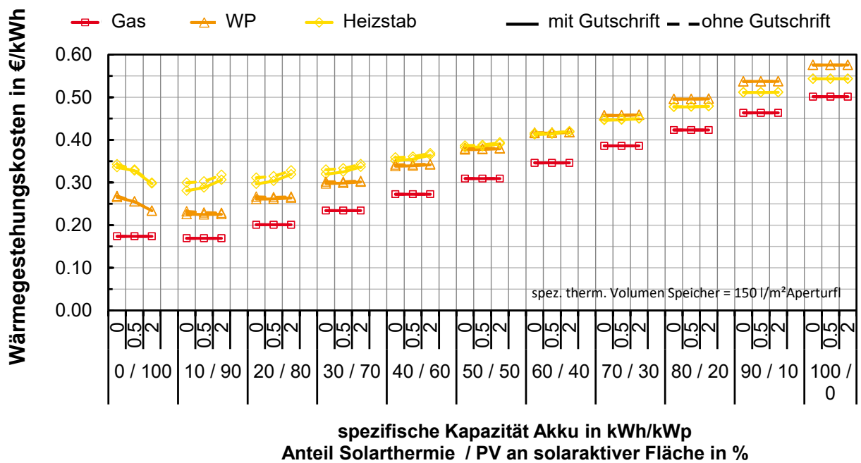
Abbildung G. 60: EFH UMK: Gestehungskosten Wärme Abhängigkeit der Konzeptvariante
