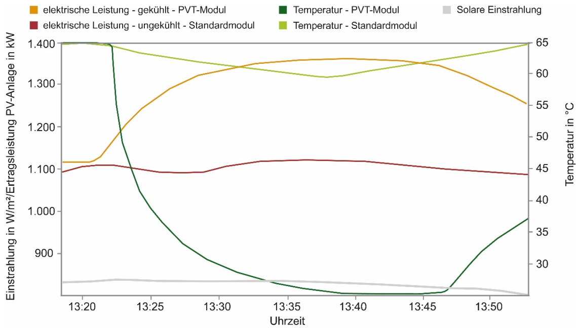
Abbildung A. 5: Schematische Darstellung der elektrischen Leistung der Module in Abhängigkeit von der Modultemperatur
