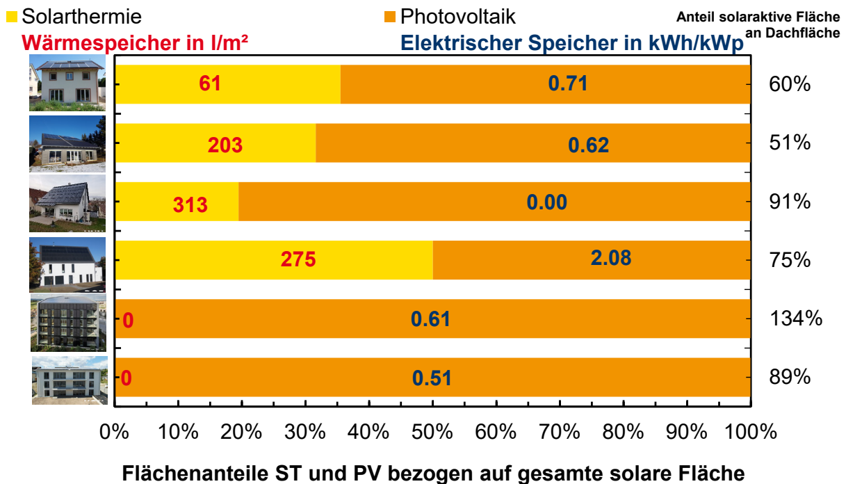
Abbildung 7-1: Dimensionierung der Anlagentechnik in den untersuchten Gebäuden.
