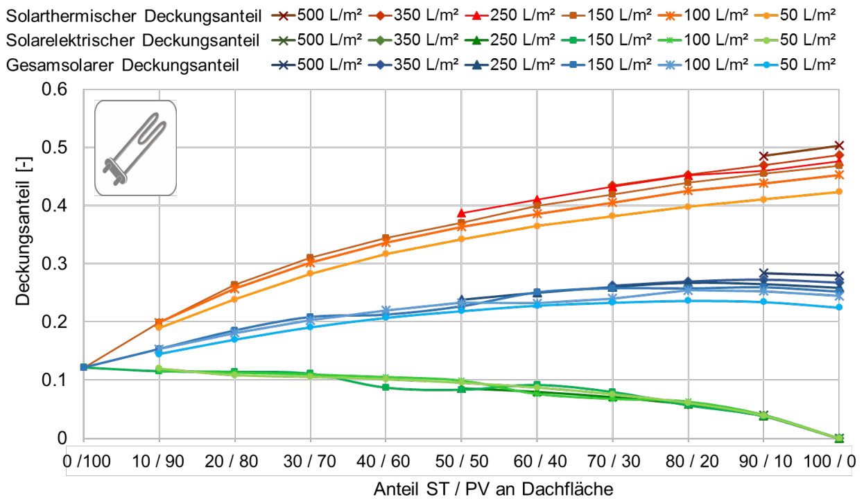
Abbildung G. 2: Solare Deckungsanteile für das EFH in DOE in Abhängigkeit der thermischen Speichergröße, Variante mit Heizstab
