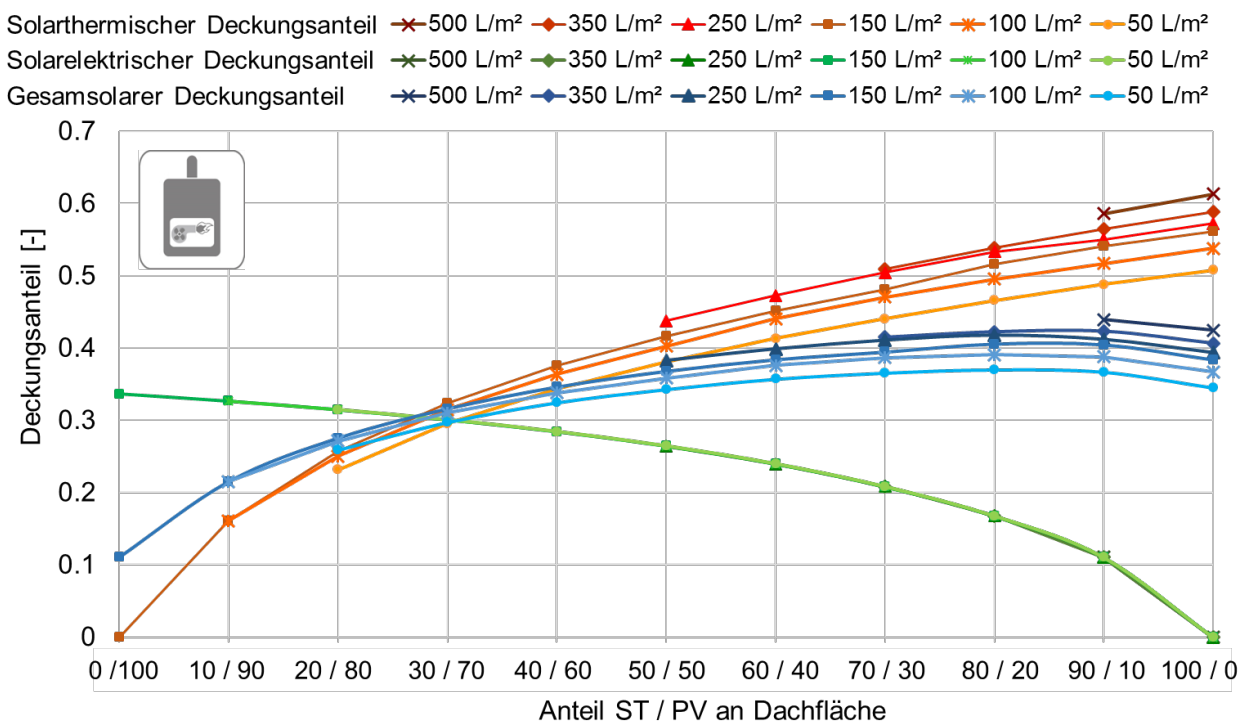
Abbildung G. 3: Solare Deckungsanteile für das EFH in DOE in Abhängigkeit der thermischen Speichergröße, Variante mit Gaskessel
