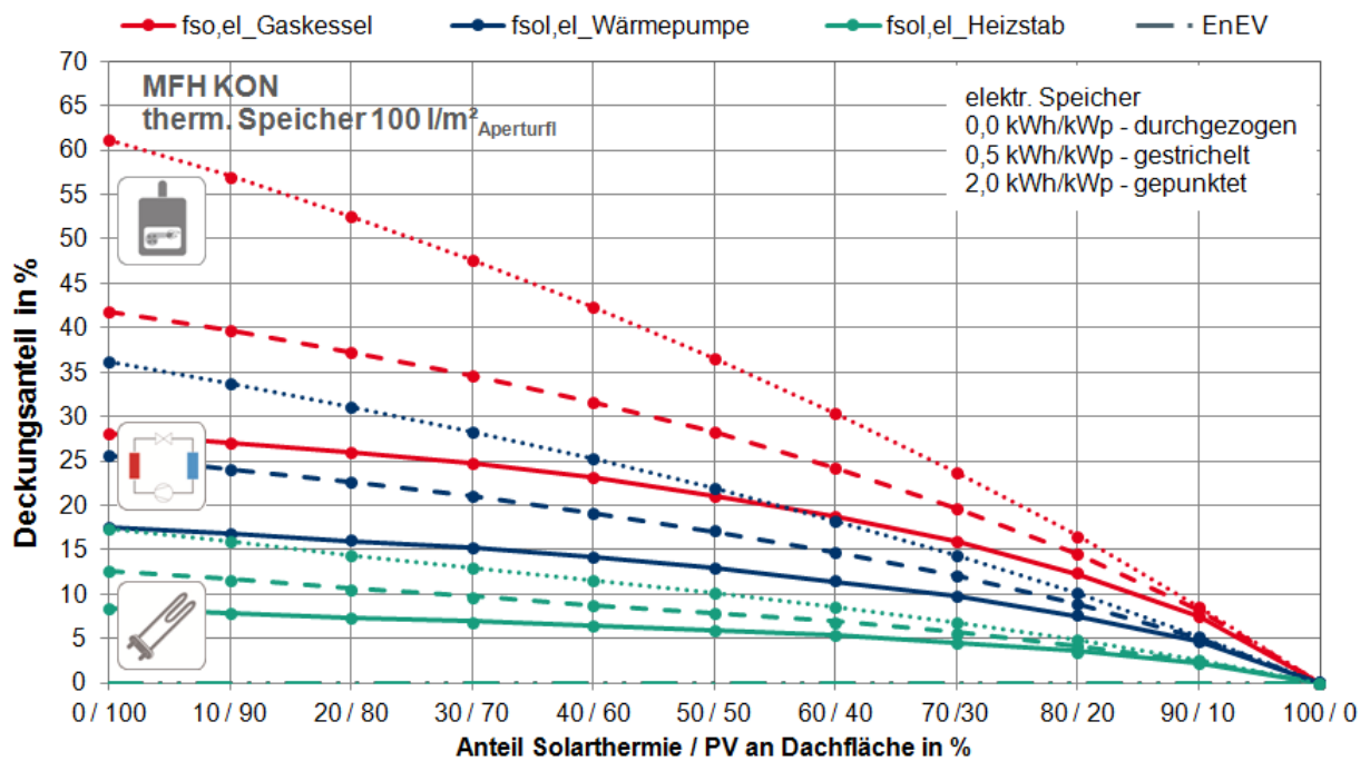
Abbildung G. 8: MFH KON: Solar elektrische Deckungsanteile f_{sol,el} am jährlichen Stromverbrauch in Abhängigkeit der Konzeptvariante
