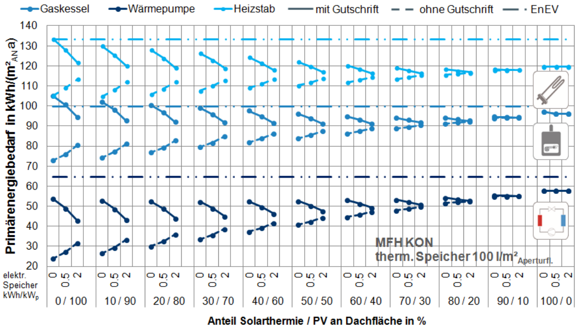
Abbildung G. 32: MFH KON: spez. Primärenergiebedarf in Abhängigkeit der Konzeptvariante während des Betriebes
