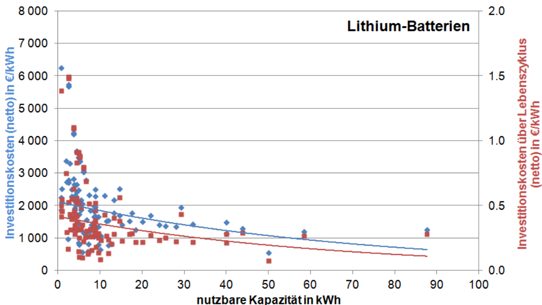
Abbildung A. 20: Investitionskosten für marktübliche Lithium-Ionen-Batterien über deren Nutzkapazität [Herstellerangaben]
