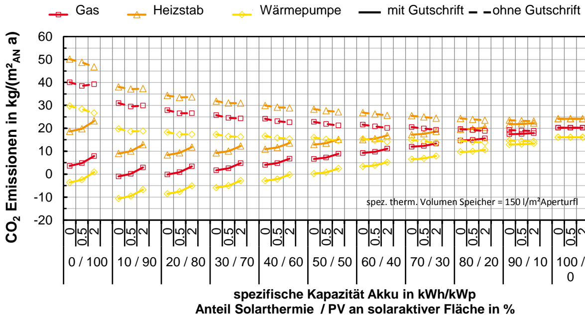
Abbildung 4-10: Arbeitsdiagramm EFH: spez. CO 2 -Emissionen in Abhängigkeit der Konzeptvariante bezogen auf den Lebenszyklus
