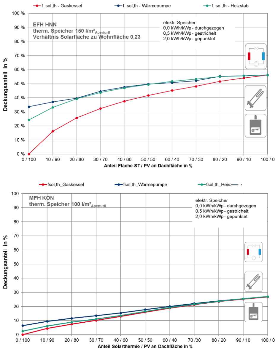
Abbildung 7-26: Vergleich der solarthermischen Deckungsanteile des EFH HNN und des MFH KON ohne elektrischem Energiespeicher
