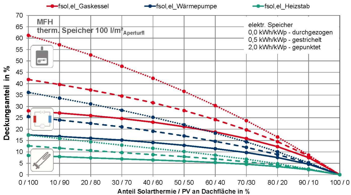
Abbildung 4-9: Arbeitsdiagramm MFH: Solar elektrische Deckungsanteile f_{sol,el} am jährlichen Stromverbrauch in Abhängigkeit der Konzeptvariante
