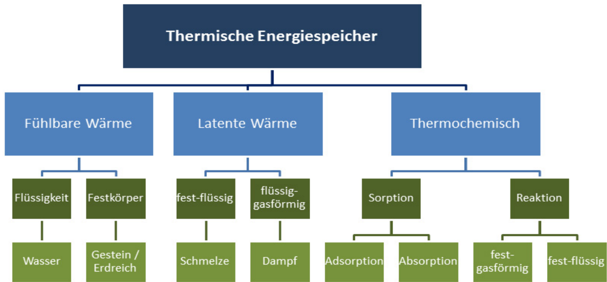
Abbildung B. 4 Einteilung thermischer Energiespeicher (TES)
