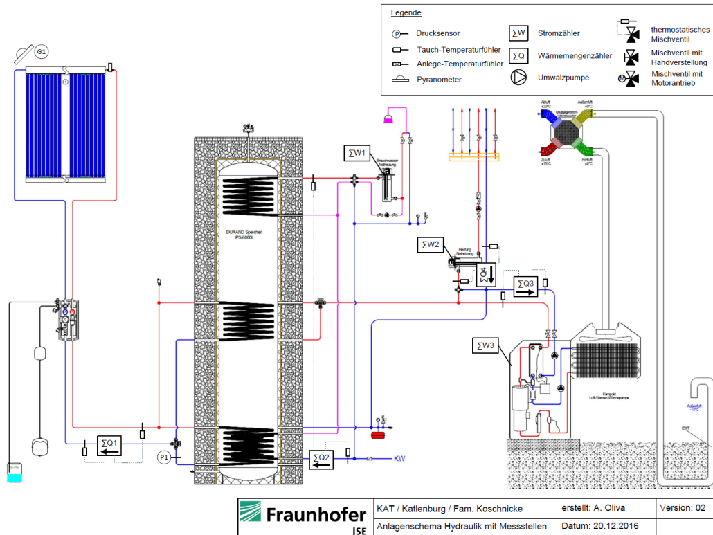
Abbildung 6-43: Energiekonzept der in Katlenburg
