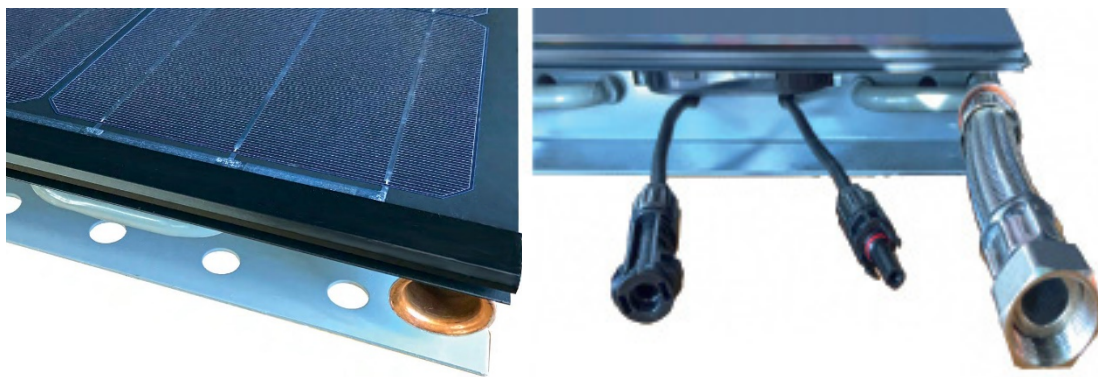
Abbildung B. 3 PVT-Kollektor (links), mit elektrischen und thermischen Anschlüssen (rechts) (Quelle: www.consolar.de )
