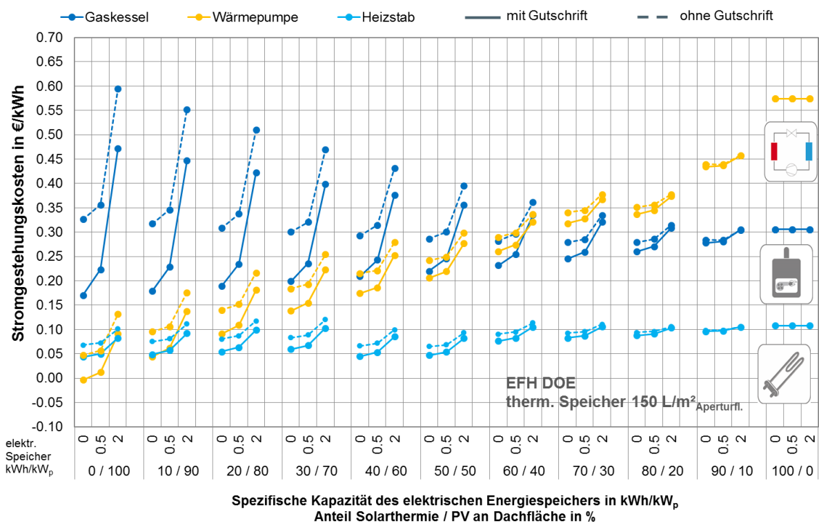
Abbildung G. 54: EFH DOE: Gestehungskosten Strom in Abhängigkeit der Konzeptvariante
