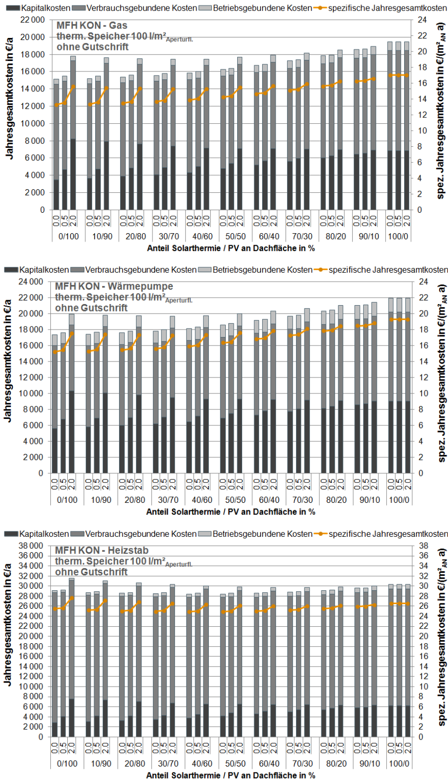
Abbildung G. 40: MFH KON: Jahresgesamtkosten in Abhängigkeit der Konzeptvariante – Gaskessel oben, Wärmepumpe Mitte und Heizstab unten
