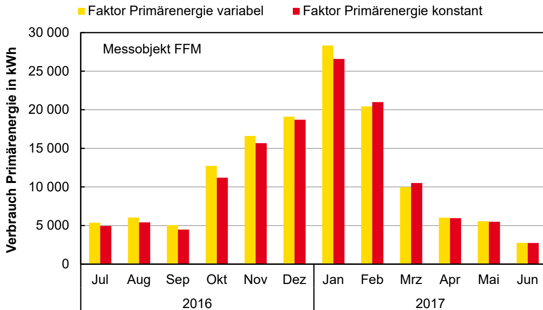
Abbildung 7-19: Verbrauch an Primärenergie für die elektrische Energieversorgung für das MFH FFM in dem Zeitraum 01.07.2016 – 30.06.2017 basierend auf stündlich aufgelösten Daten
