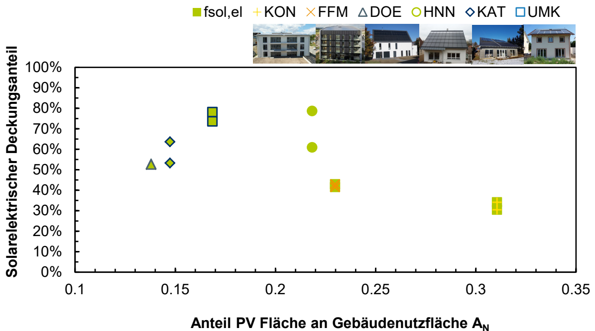
Abbildung 7-6: Solarelekttrischer Deckungsanteil in den messtechnisch untersuchten Gebäuden, Messzeitraum 16/17 und 17/18
