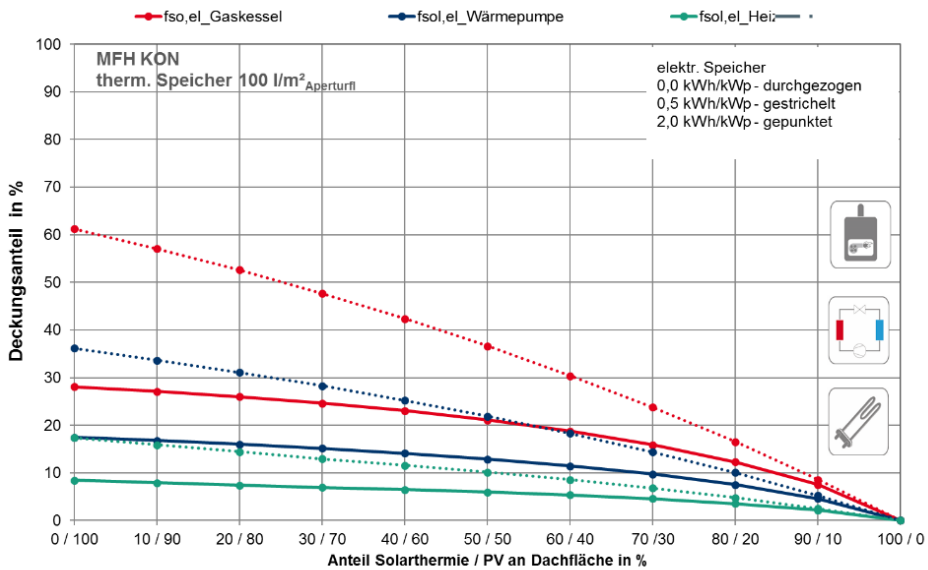
Abbildung 7-29: Vergleich der solarelektrischen Deckungsanteile des EFH UMK und des MFH KON ohne und mit elektrischem Energiespeicher mit 2.0 kWh/kW p
