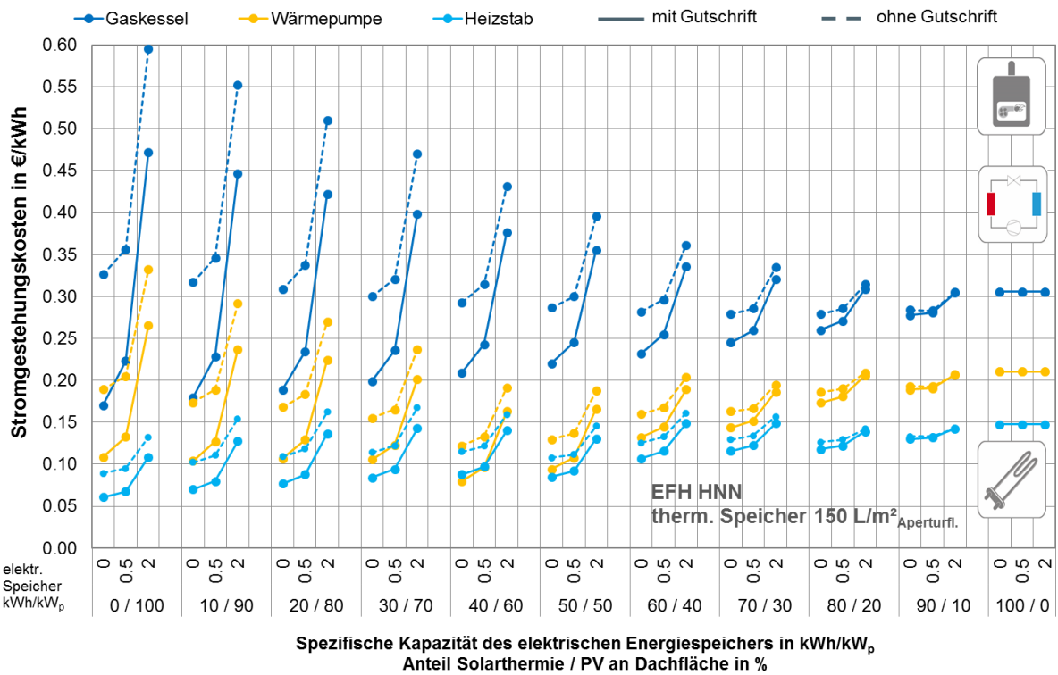
Abbildung G. 56: EFH HNN: Gestehungskosten Strom in Abhängigkeit der Konzeptvariante
