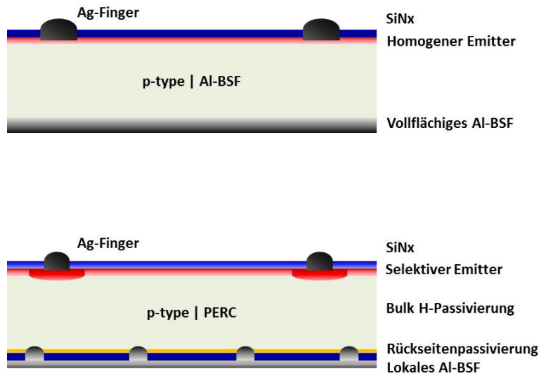
Abbildung A. 25: Derzeit gefertigte Siliziumsolarzellen nach dem Al-BSF-Konzept (oben), Aufbau der PERC-Solarzelle (unten) © Solarworld AG [37]
