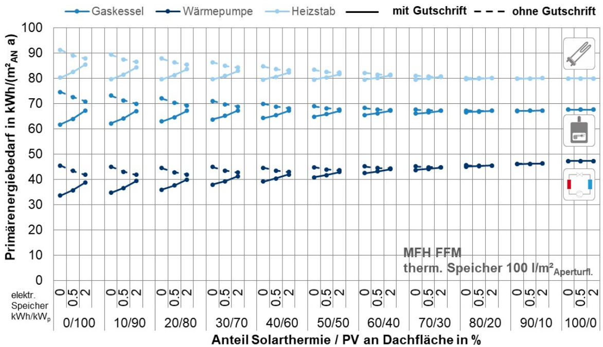
Abbildung G. 35: MFH FFM: spez. Primärenergiebedarf in Abhängigkeit der Konzeptvariante bezogen auf den Lebenszyklus
