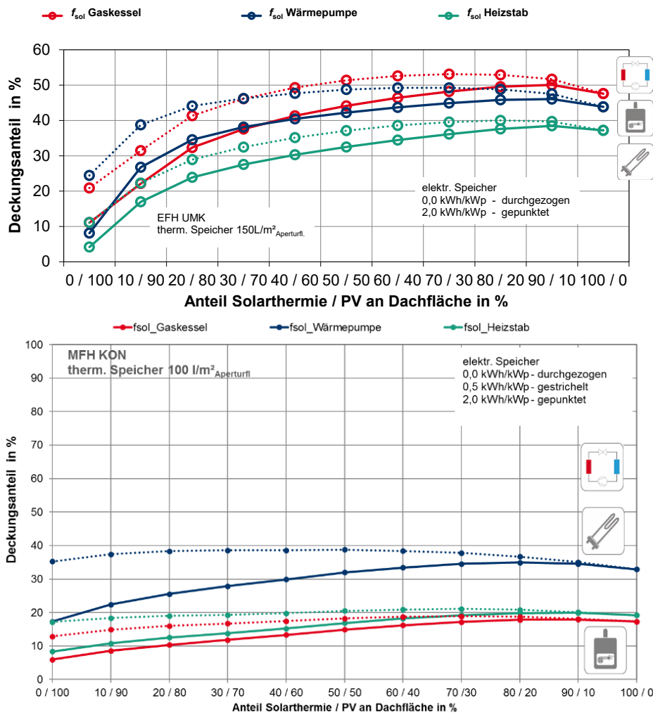
Abbildung 7-25: Vergleich der gesamtsolaren Deckungsanteile des EFH UMK und des MFH KON ohne und mit elektrischem Energiespeicher mit 2.0 kWh/kW p
