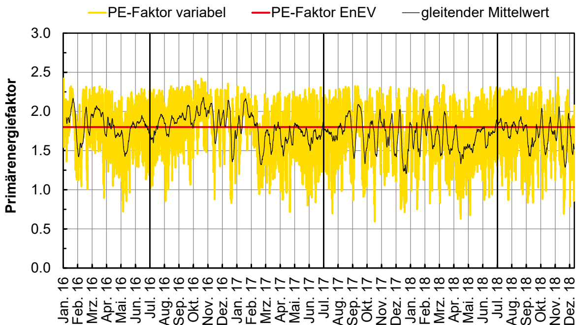
Abbildung 7-16: Vergleich der variablen Primärenergiefaktoren, basierend auf aufbereiteten Daten aus den EnergyCharts [21] im Vergleich mit dem konstanten Primärenergiefaktor nach EnEV 2016 für die Jahre 2016 – 2018
