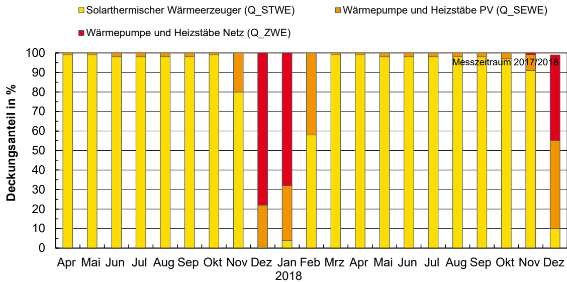
Abbildung 6-45: Anteile der installierten Wärmeerzeuger an der Versorgung des Gebäudes über die gesamte Messperiode
