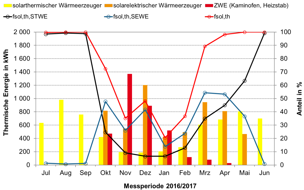
Abbildung 6-37: Monatliche Wärmeerzeugung nach Wärmequellen sowie die solarthermischen Deckungsanteile für den Messzeitraum 2016/2017 des Gebäudes in Heilbronn-Neckargartach
