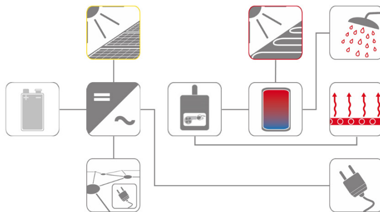
Abbildung 3-6: Schema für ein auf fossilen Energieträgern basierendes, solares Energieversorgungskonzept, optional auch mit elektrischem Energiespeicher möglich
