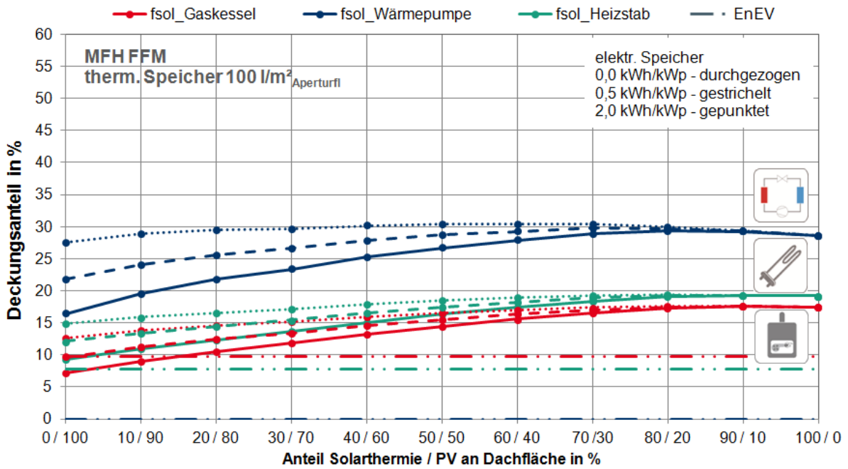
Abbildung G. 9: MFH FFM: Gesamt solarer Deckungsanteile: f_{sol} am jährlichen Energieverbrauch in Abhängigkeit der Konzeptvariante
