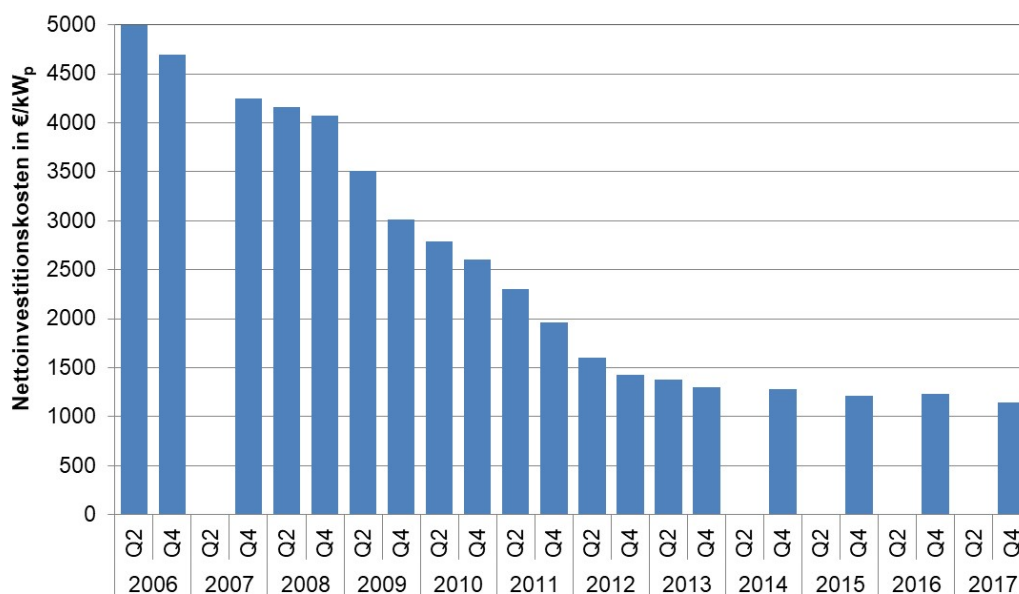
Abbildung A. 3: Nettoinvestitionskosten von fertig installierten PV-Aufdachanlagen €/kWp, gültig für Anlagengrößen von 10 bis 100 kWp (Stand Q4 2017) (in Anlehnung an [9] und [10])
