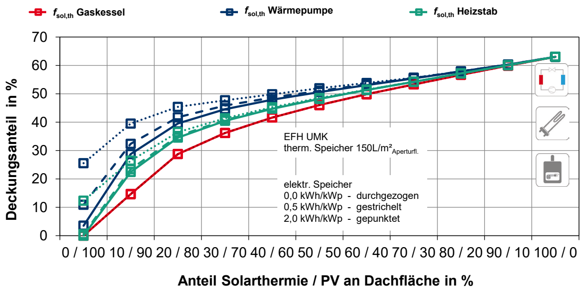
Abbildung G. 22: EFH UMK: Solar thermische Deckungsanteile f_{sol,th} an der Wärmebereitstellung in Abhängigkeit der Konzeptvariante
