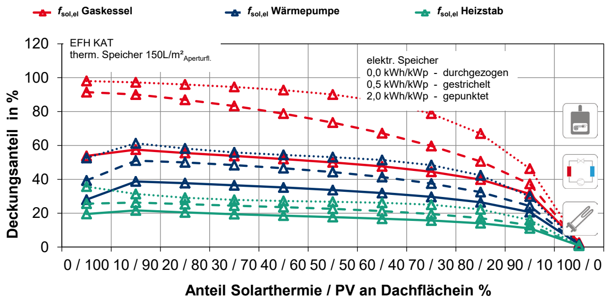
Abbildung G. 20: EFH KAT: Solar elektrische Deckungsanteile f_{sol,el} am jährlichen Stromverbrauch in Abhängigkeit der Konzeptvariante
