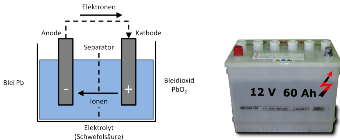
Abbildung A. 17: Schematischer Aufbau einer Blei-Säure-Batterie [eigene Darstellung] (links) und Blei-Säure-Batterie [28] (rechts)
