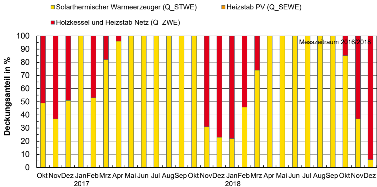
Abbildung 6-56: Anteile der installierten Wärmeerzeuger an der Versorgung des Gebäudes über die gesamte Messperiode
