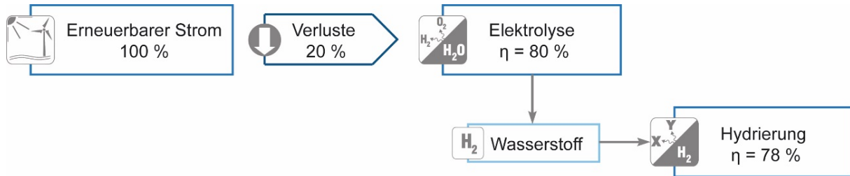
Abbildung A. 26: Erzeugung von Liquid Organic Hydrogen Carriers (LOHC) durch die Aufnahme von Wasserstoff
