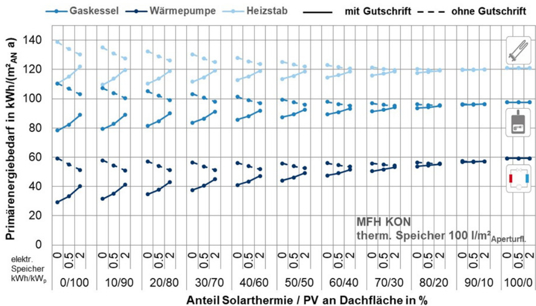
Abbildung 7-32: Vergleich des Primärenergiebedarfs des EFH HNN und des MFH KON ohne und mit Gutschrift für eingespeisten Strom
