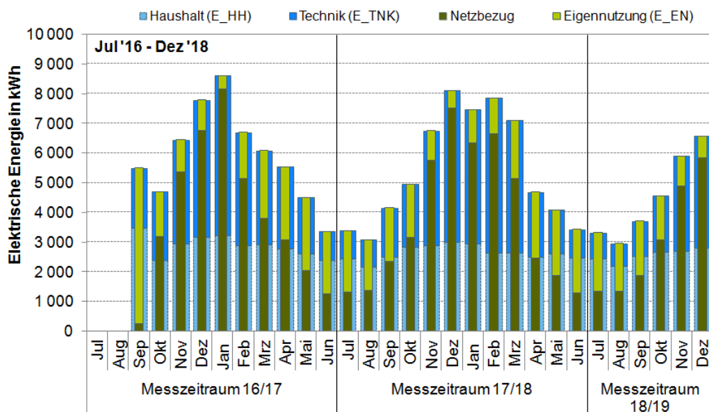
Abbildung 6-9: MFH KON: Monatlicher Stromverbrauch
