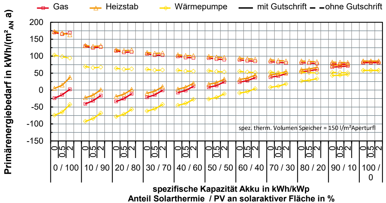
Abbildung G. 39: EFH UMK: spez. Primärenergiebedarf in Abhängigkeit der Konzeptvariante bezogen auf den Lebenszyklus
