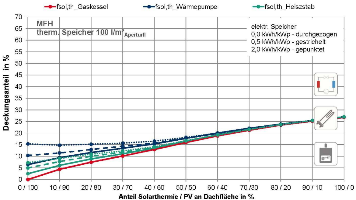
Abbildung 4-7: Arbeitsdiagramm MFH: Solar thermische Deckungsanteile f_{sol,th} an der Wärmebereitstellung in Abhängigkeit der Konzeptvariante
