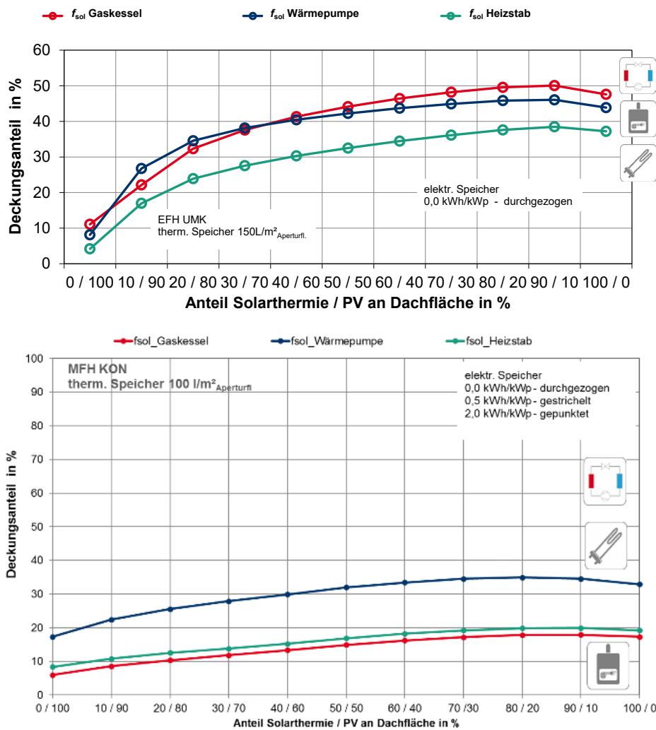
Abbildung 7-24: Vergleich der gesamtsolaren Deckungsanteile der EFH HNN und des MFH KON ohne elektrischem Energiespeicher
