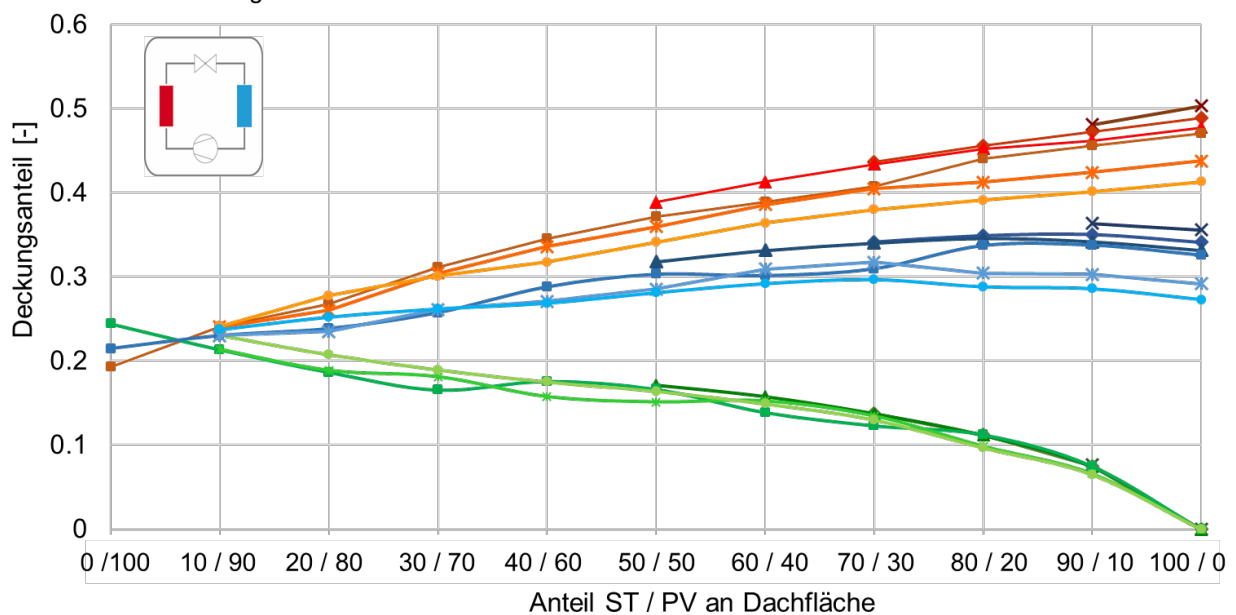
Abbildung G. 1: Solare Deckungsanteile für das EFH in DOE in Abhängigkeit der thermischen Speichergröße, Variante mit Wärmepumpe
