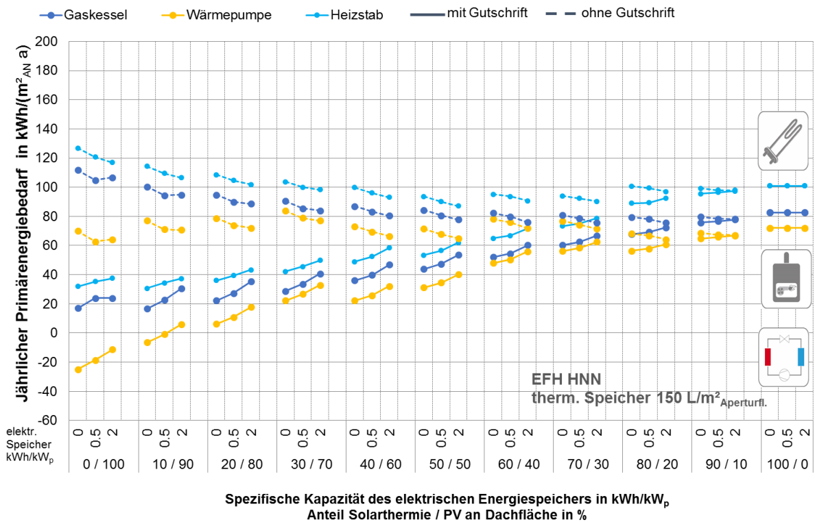
Abbildung G. 36: EFH HNN: spez. Primärenergiebedarf in Abhängigkeit der Konzeptvariante bezogen auf den Lebenszyklus
