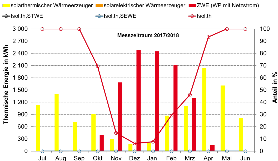
Abbildung 6-29: Monatliche Wärmeerzeugung nach Wärmequellen sowie die solarthermischen Deckungsanteile für den Messzeitraum 2017/2018 des Gebäudes in Döhlau
