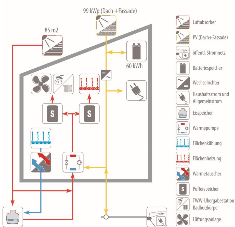
Abbildung 6-15: MFH FFM Energiekonzept
