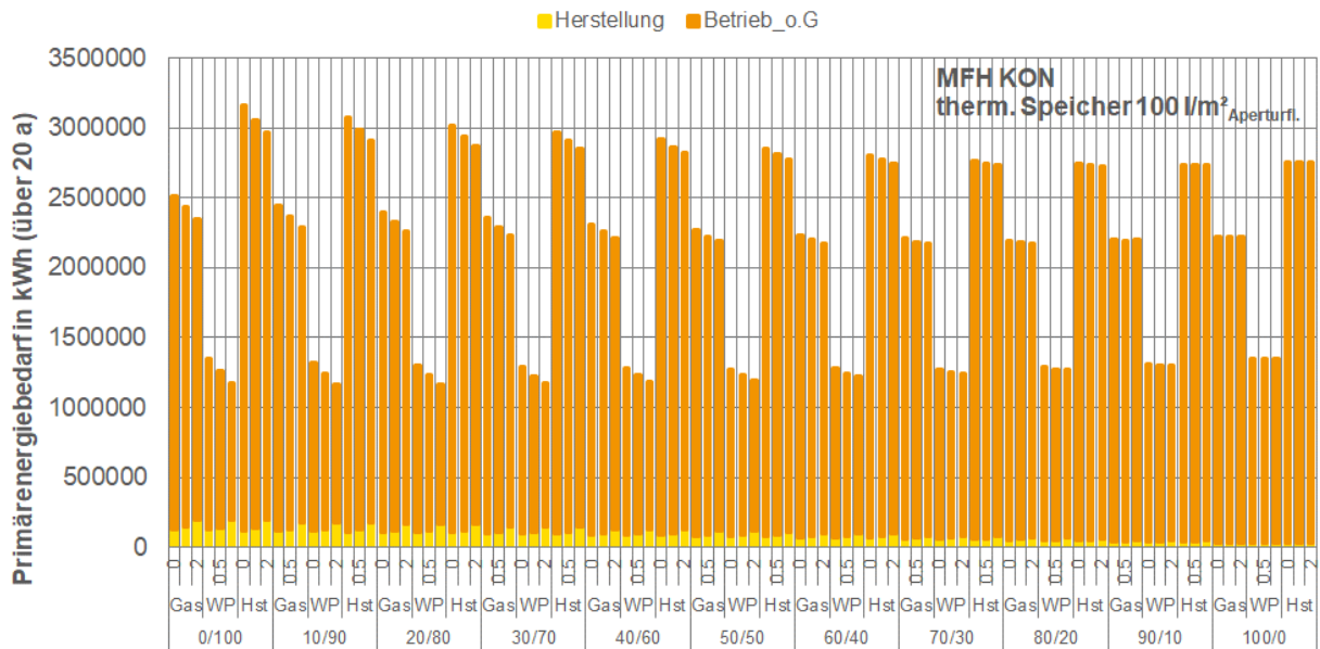
Abbildung G. 33: MFH KON: Primärenergiebedarf in Abhängigkeit der Konzeptvariante bezogen auf den Lebenszyklus, Einfluss / Anteile aus Herstellung und Betrieb
