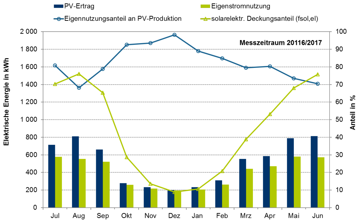
Abbildung 6-31: Monatlicher PV-Ertrag und sowie der Eigennutzungsanteil und der solarelektrische Deckungsanteil für den Messzeitraum 2016/2017 des Gebäudes in Döhlau
