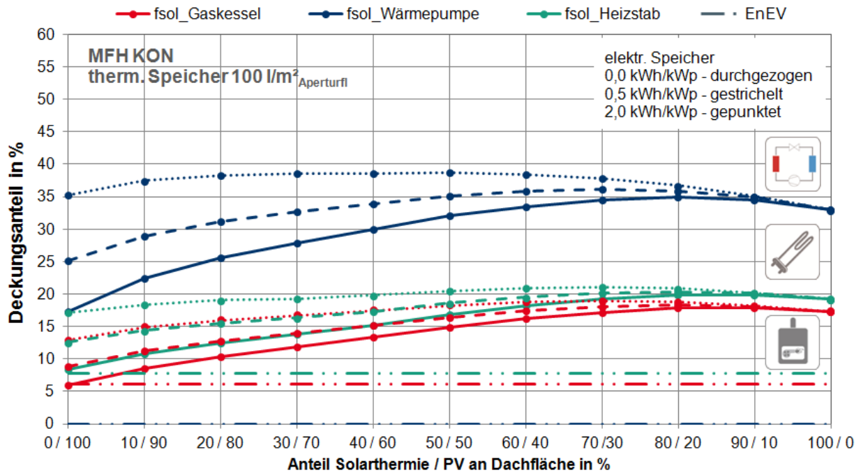
Abbildung G. 6: MFH KON: Gesamt solarer Deckungsanteile: f_{sol} am jährlichen Energieverbrauch in Abhängigkeit der Konzeptvariante
