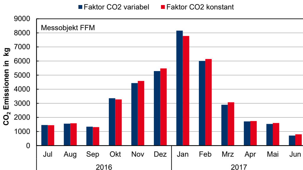
Abbildung 7-23: An den Bezug von elektrischer Energie gebundene CO 2 Emissionen für das MFH FFM in dem Zeitraum 01.07.2016 – 30.06.2017 basierend auf stündlich aufgelösten Daten
