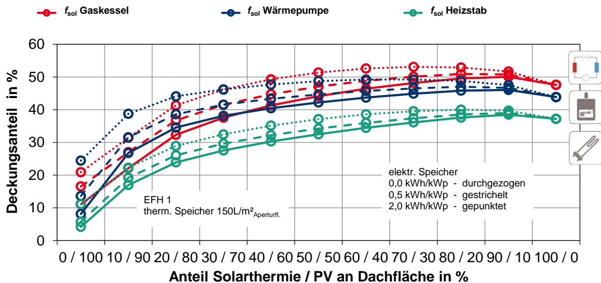
Abbildung 4-4: Arbeitsdiagramm EFH: Gesamt solarer Deckungsanteile: f_{\text{sol}} am jährlichen Energieverbrauch in Abhängigkeit der Konzeptvariante
