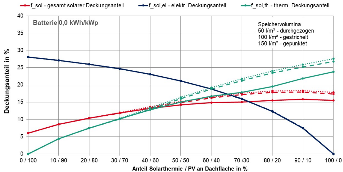
Abbildung 5-6: Einfluss des Verhältnisses von thermischer Speichergröße zur Aperturfläche auf den solaren Deckungsanteil beim Mehrfamilienhaus
