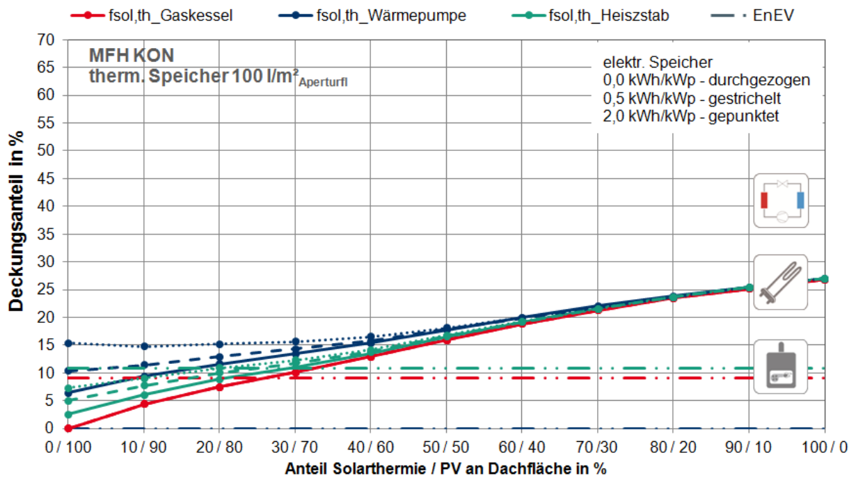
Abbildung G. 7: MFH KON: Solar thermische Deckungsanteile f_{sol,th} an der Wärmebereitstellung in Abhängigkeit der Konzeptvariante
