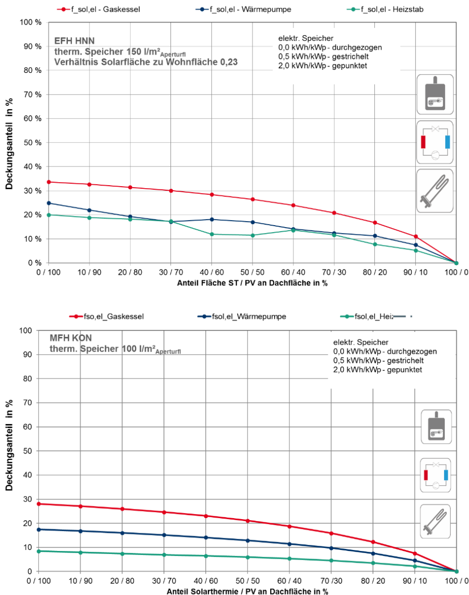
Abbildung 7-28: Vergleich der solarelektrischen Deckungsanteile des EFH HNN und des MFH KON ohne elektrischem Energiespeicher
