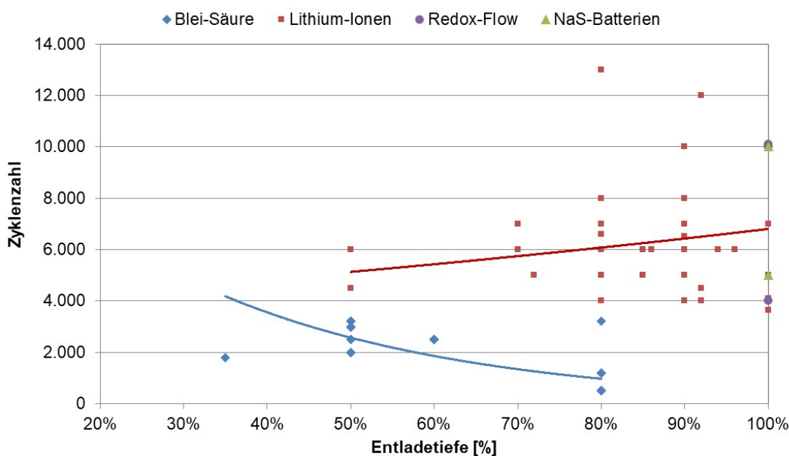
Abbildung A. 16: Zyklenzahl für Batterien in Abhängigkeit der Entladetiefe
