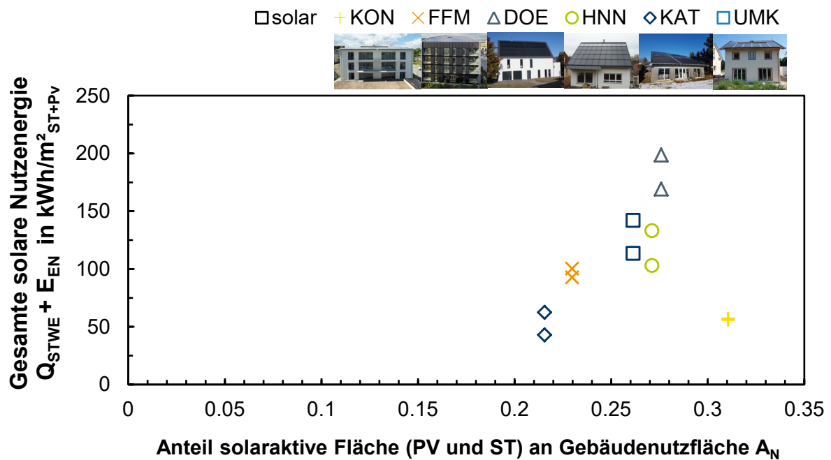
Abbildung 7-13: Gesamtsolare Nutzenergie aus dem solarthermischen Wärmeerzeuger Q_{STWE} sowie der eigengenutzten elektrischen Energie aus der PV Anlage über dem Anteil der gesamtsolaren Flächen an der Gebäudenutzfläche A_N , Messzeitraum 16/17 und 17/18
