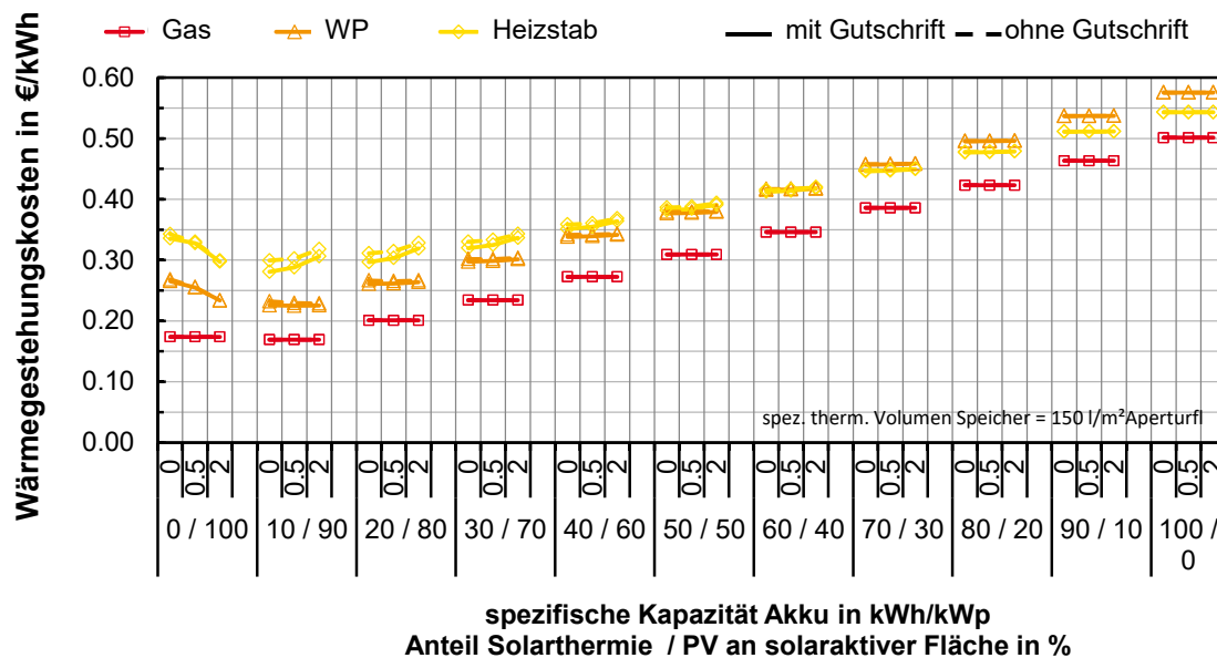
Abbildung 7-36: EFH UMK: Gestehungskosten Wärme in Abhängigkeit der Konzeptvariante
