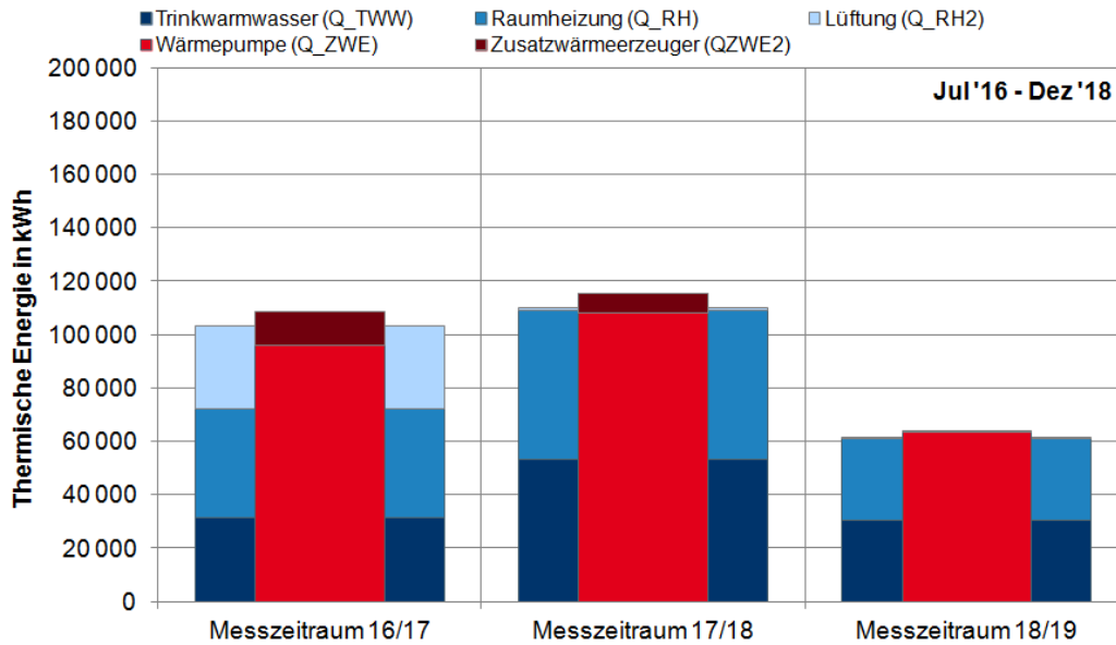
Abbildung 6-17: MFH FFM: Jahreswärmeverbrauch Heizung und Trinkwarmwasser und Wärmebereitstellung der Wärmepumpen
