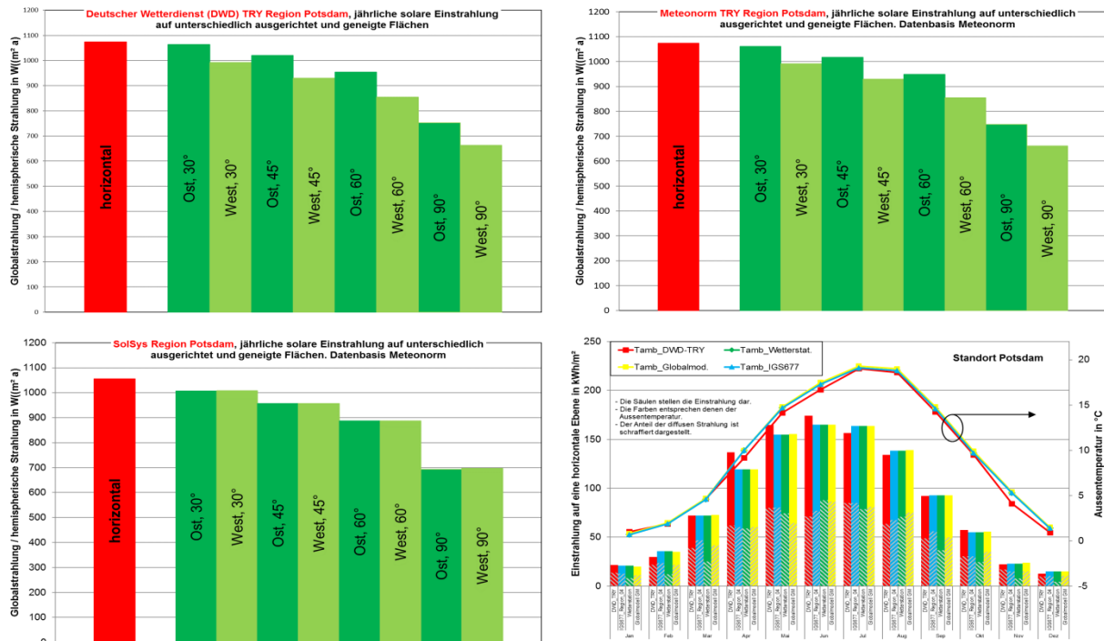
Abbildung 5-3: Globalstrahlung der Testreferenzjahre für Potsdam a) des Deutschen Wetterdienstes (oben, links) und b) mittels Meteonorm® für dieselben Klimaregionen generiert (oben, rechts) sowie mittels Meteonorm® als Referenzwetterdaten für SolSys generierte Wetterdaten (unten, links) und Monatssummen der solaren Einstrahlung auf eine horizontale Ebene und Mittelwerte der Außentemperaturen diverser mittels Meteonorm® generierten Wetterdaten (unten, rechts)
