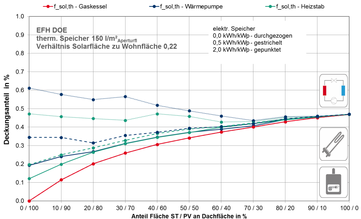
Abbildung G. 16: EFH DOE: Solar thermische Deckungsanteile f_{sol,th} an der Wärmebereitstellung in Abhängigkeit der Konzeptvariante
