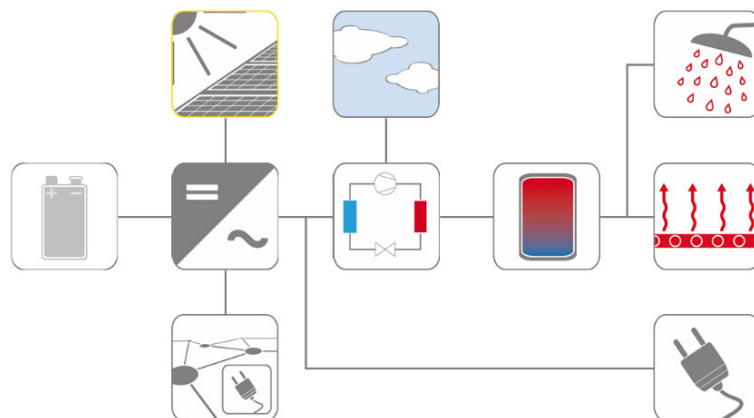
Abbildung 3-4: Schema für ein strombasiertes Energieversorgungskonzept mit optionalem elektrischem Energiespeicher
