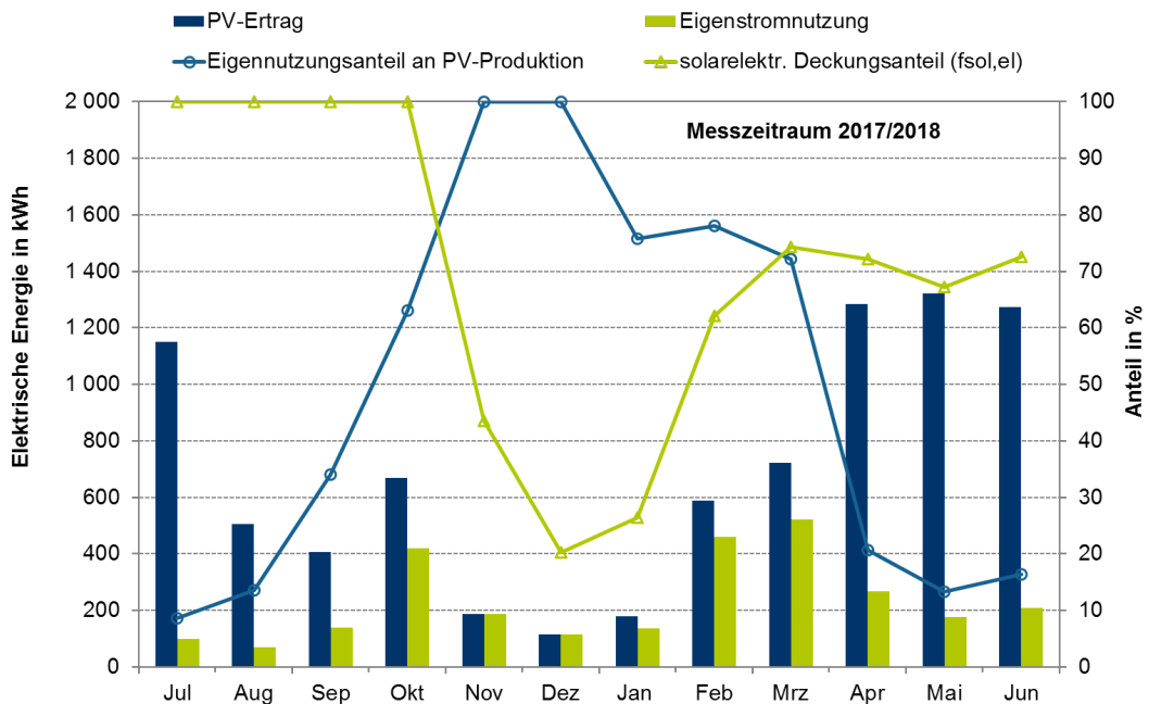
Abbildung 6-41: Monatlicher PV-Ertrag und sowie der Eigennutzungsanteil und der solarelektrische Deckungsanteil für den Messzeitraum 2017/2018 des Gebäudes HNN
