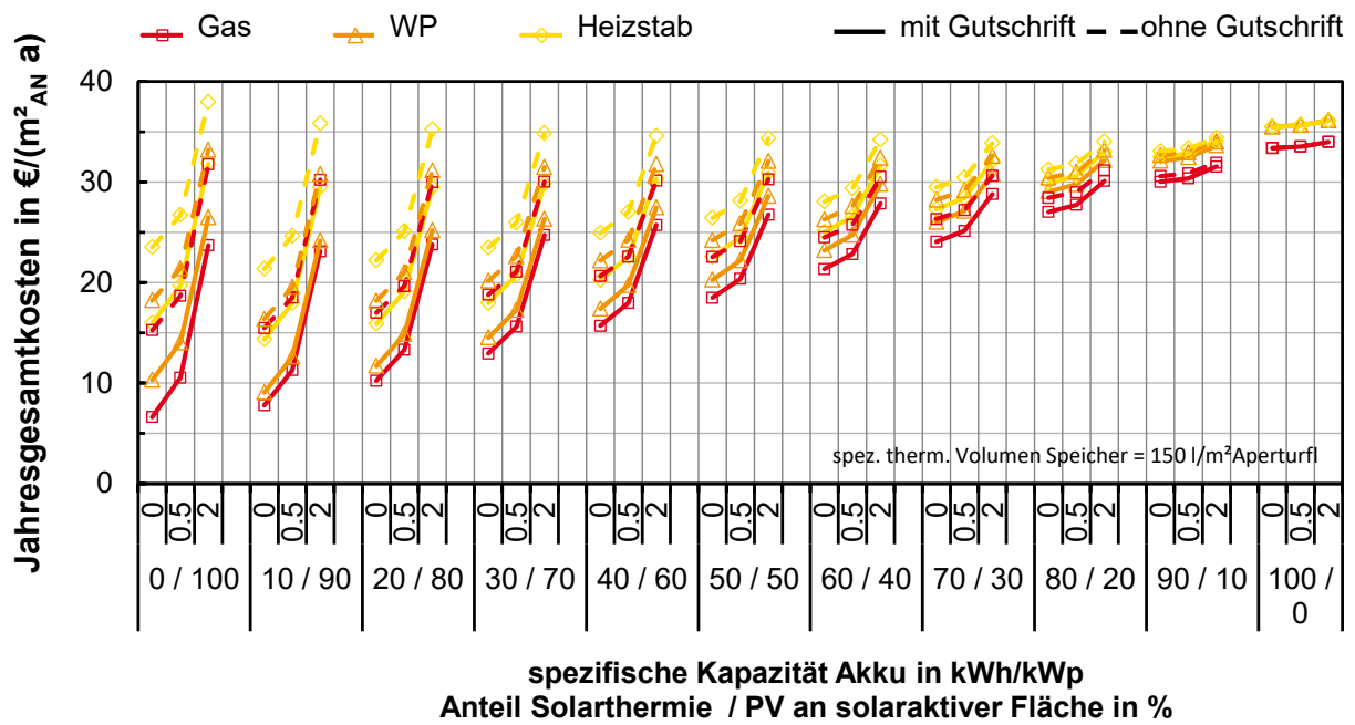
Abbildung G. 47: EFH KAT: spez. Jahresgesamtkosten in Abhängigkeit der Konzeptvariante
