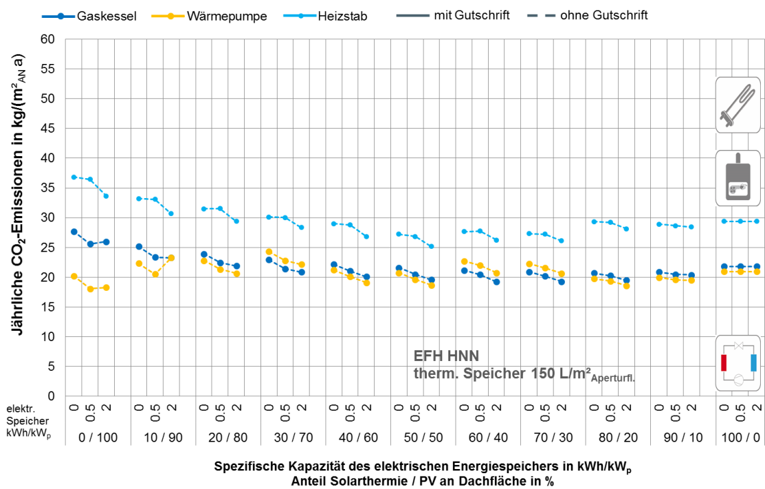
Abbildung 7-30: Vergleich der CO 2 -Emissionen des EFH HNN und des MFH KON ohne Gutschrift für eingespeisten Strom
