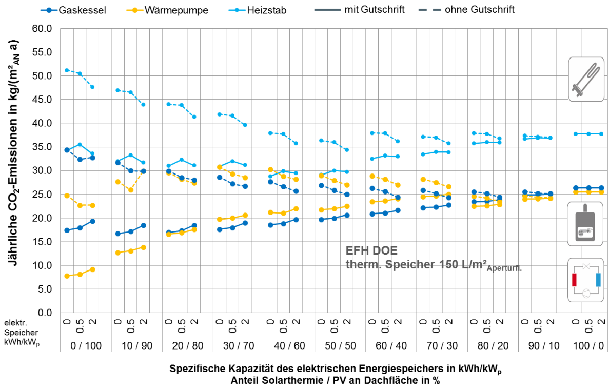
Abbildung G. 29: EFH DOE spez. CO 2 -Emissionen in Abhängigkeit der Konzeptvariante bezogen auf ein Jahr über den gesamten Lebenszyklus von 20 Jahren
