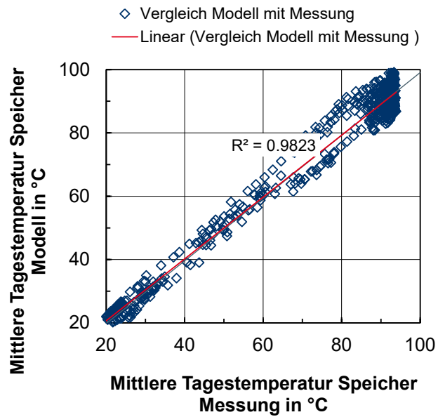
Abbildung 6-64: Vergleich der auf Messdaten basierenden mittleren Speichertemperaturen mit den modellierten Werten
