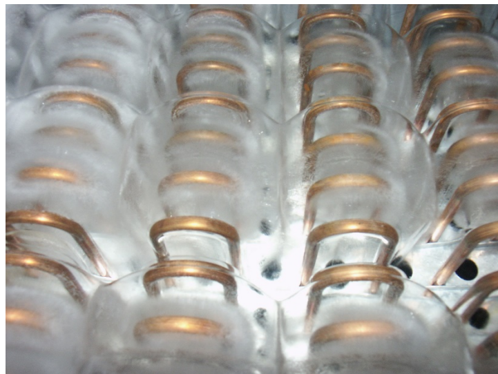
Abbildung B. 7 Eisspeicher, Sicht auf die Wärmeübertragerrohre während des Kristallisationsprozesses
