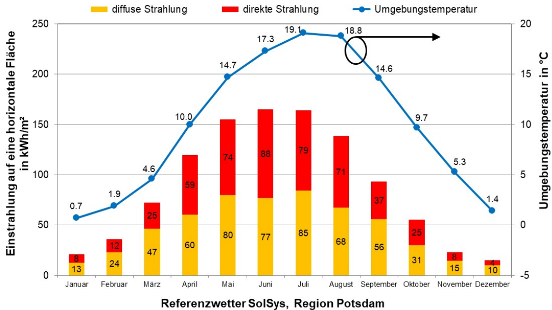
Abbildung 5-4: Monatssummen der Einstrahlung auf eine horizontale Fläche und Mittelwerte der Umgebungstemperatur, Referenzwetter Region Potsdam
