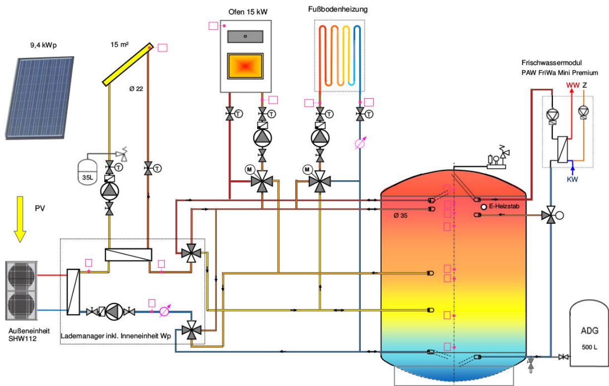
Abbildung 6-34: Energiekonzept des Gebäudes in Heilbronn-Neckargartach
