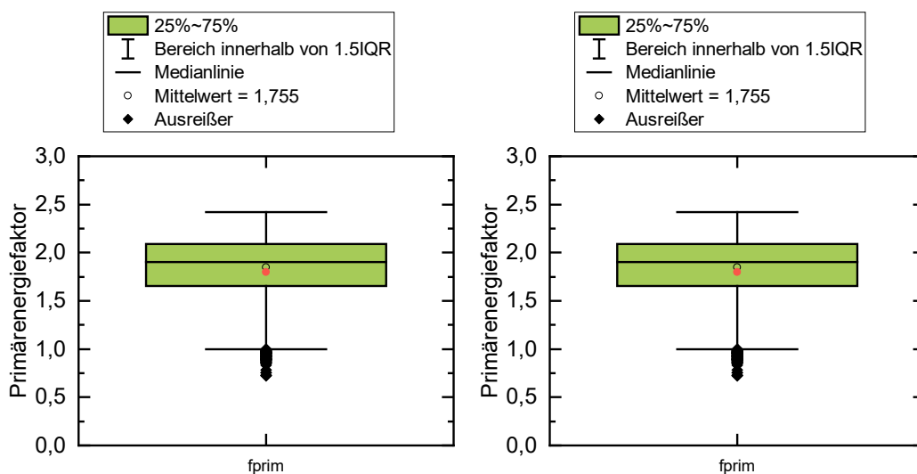
Abbildung 7-17: Boxplot über die variablen Primärenergiefaktoren für den Zeitraum 01.07.2016 – 30.06.2017 (links) und 01.07.2017 – 30.06.2018 (rechts) im Vergleich mit dem konstanten Faktor von 1,8 nach EnEV (roter Punkt)
