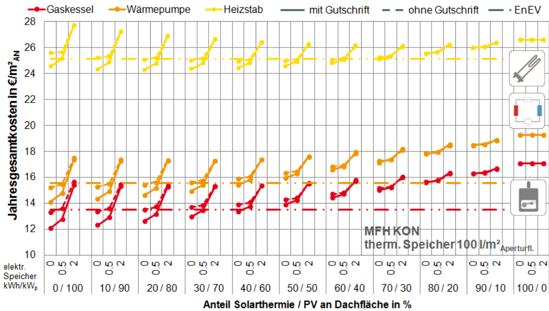
Abbildung 7-33: MFH KON: spez. Jahresgesamtkosten in Abhängigkeit der Konzeptvariante
