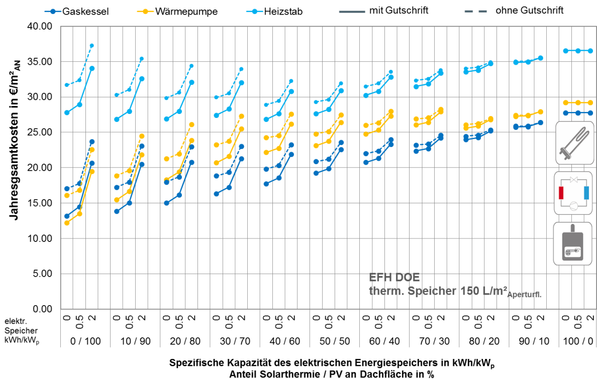
Abbildung G. 45: EFH DOE: spez. Jahresgesamtkosten in Abhängigkeit der Konzeptvariante
