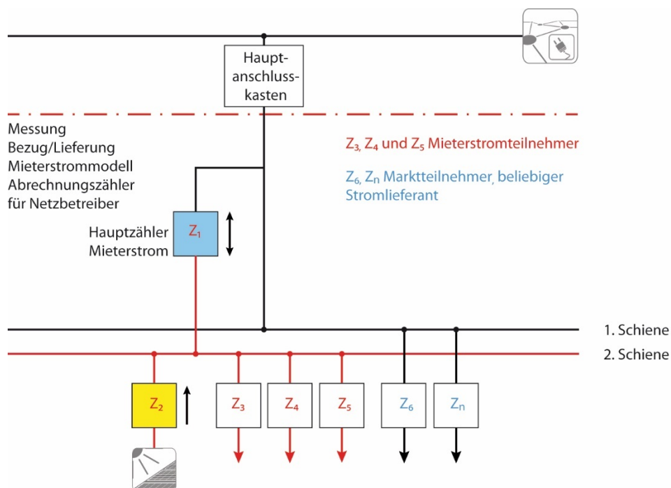
Abbildung 9-2: Messprinzip Doppelte Sammelschiene (nach [48])
