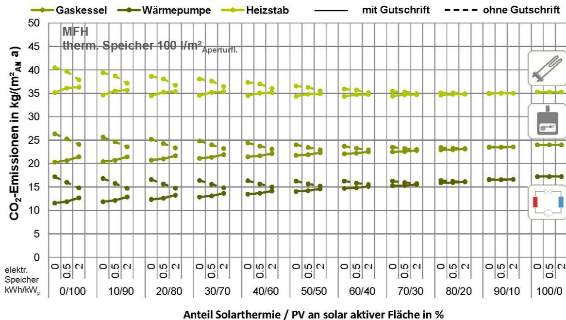
Abbildung 4-12: Arbeitsdiagramm MFH: spez. CO 2 -Emissionen in Abhängigkeit der Konzeptvariante bezogen auf den Lebenszyklus
