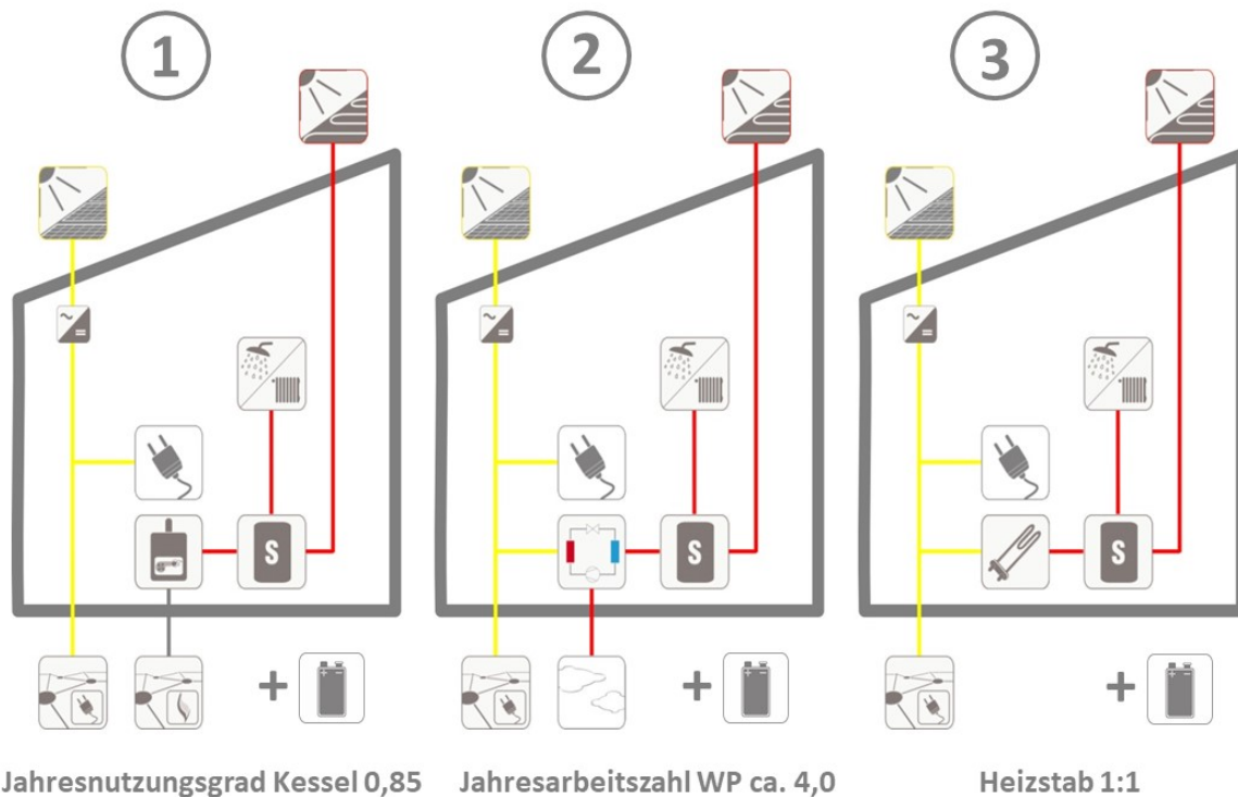
Abbildung 3-18: Varianten der Energieversorgungskonzepte mit Solarthermie und Photovoltaik sowie unterschiedlichen Wärmeerzeugersystemen, mit und ohne elektrischem Speicher
