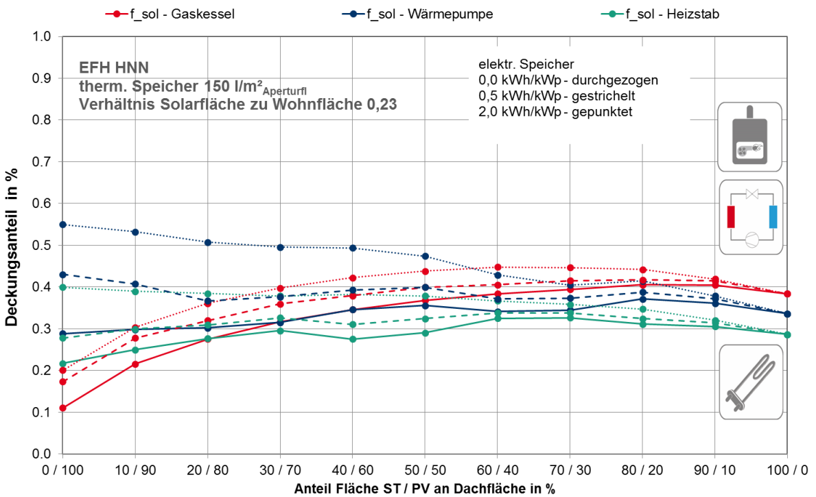
Abbildung G. 12: EFH HNN: Gesamt solarer Deckungsanteile: f_{sol} am jährlichen Energieverbrauch in Abhängigkeit der Konzeptvariante
