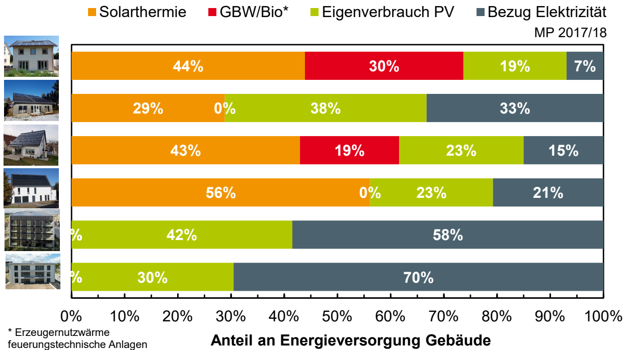
Abbildung 7-15: Detailliertere Aufteilung der Energieversorgung der Gebäude mit elektrischer Energie und Wärme in solar bereitgestellte Energie über den solarthermischen Wärmeerzeuger, dem Eigenverbrauch aus der PV Anlage und extern bezogener Energie zur Beheizung und Versorgung mit elektrischer Energie für den Messzeitraum 2017/18
