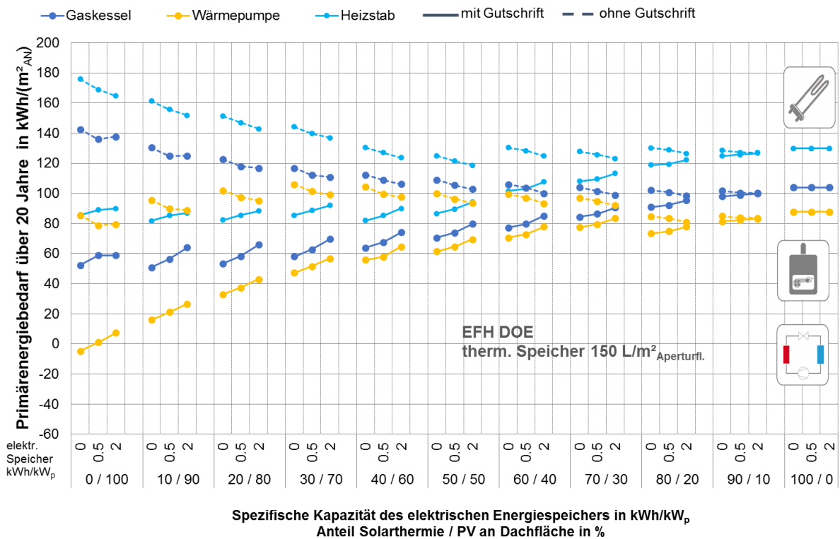
Abbildung G. 37: EFH DOE: spez. Primärenergiebedarf in Abhängigkeit der Konzeptvariante bezogen auf den Lebenszyklus
