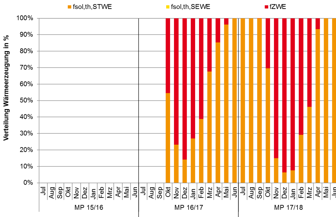
Abbildung 6-30: Anteile der monatlichen Wärmeerzeugung nach Wärmequellen für den Messzeitraum 2016/2017 und 2017/2018 des Gebäudes in Döhlau
