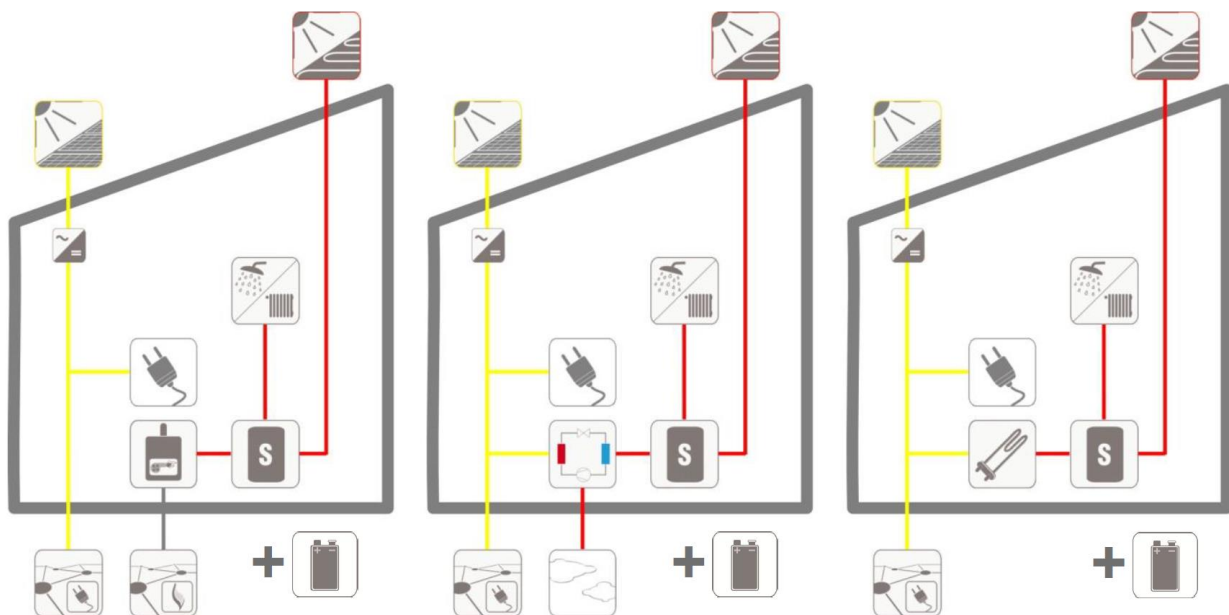
Abbildung 4-1: Systemkonzepte für solarbasierte Versorgungskonzepte
