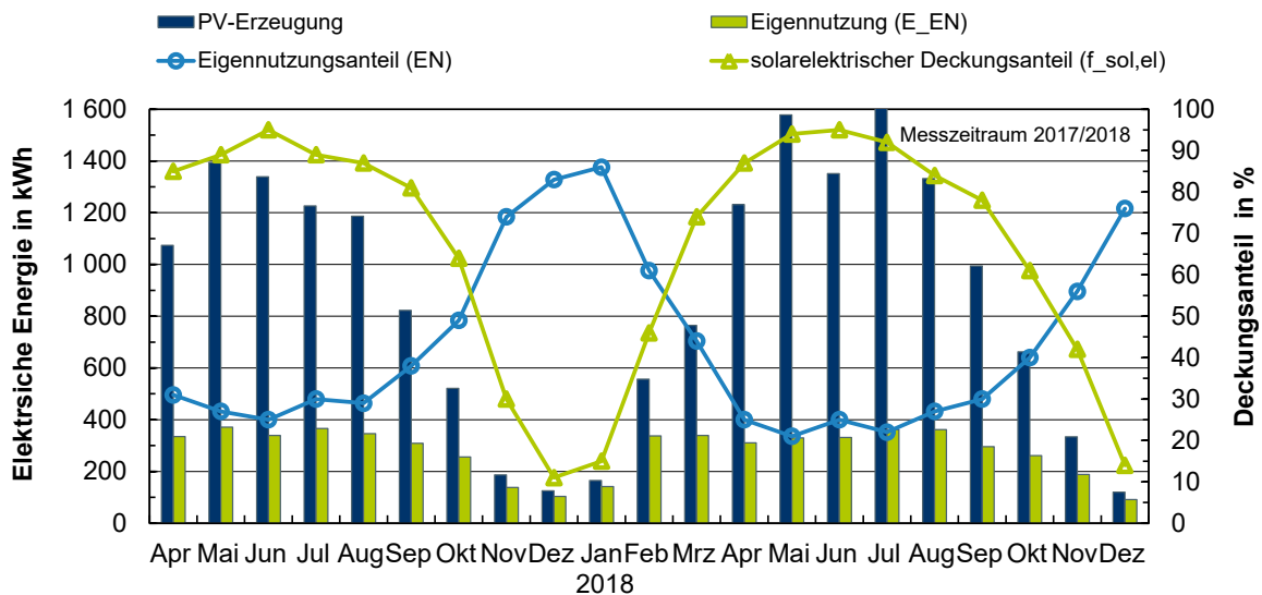
Abbildung 6-49: Monatliche Messdaten für die Elektrizitätsversorgung über den gesamten Messzeitraum
