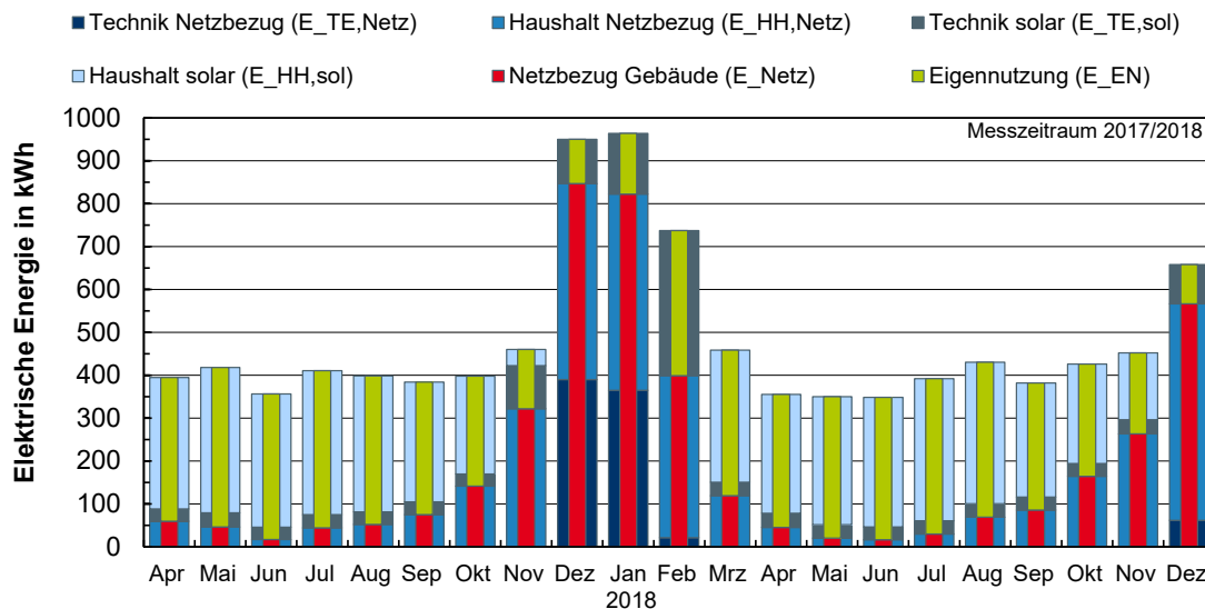
Abbildung 6-50: Monatliche Messdaten für die Elektrizitätsversorgung aus dem gesamten mess-technisch untersuchten Zeitraum
