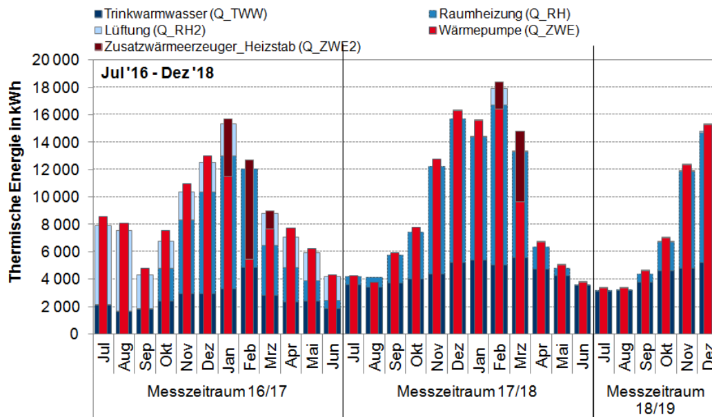
Abbildung 6-16: MFH FFM: Monatlicher Wärmeverbrauch Heizung und Trinkwarmwasser
