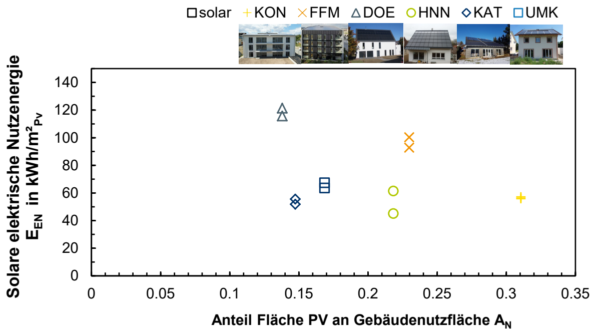
Abbildung 7-12: Spezifische selbstgenutzte elektrische Erträge der PV Anlage E_{EN} über dem Anteil der Bruttomodulfläche an der Gebäudenutzfläche A_N , Messzeitraum 16/17 und 17/18
