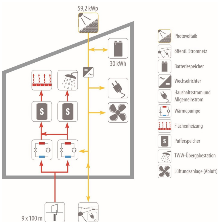
Abbildung 6-4: MFH KON Energiekonzept
