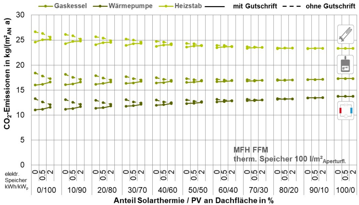
Abbildung G. 27: MFH FFM: spez. CO 2 -Emissionen in Abhängigkeit der Konzeptvariante bezogen auf den Lebenszyklus
