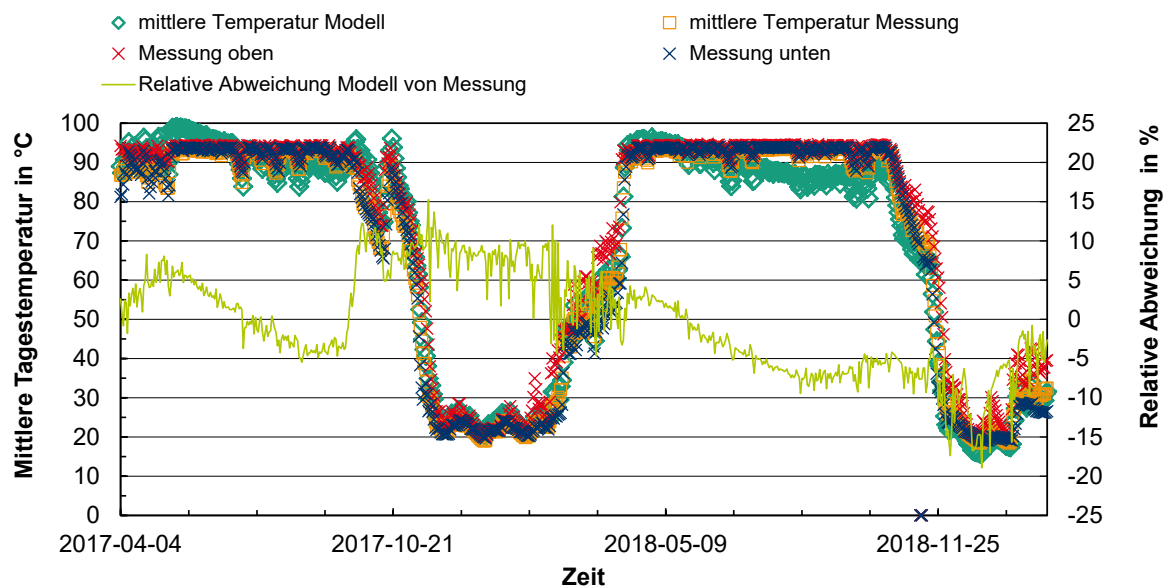
Abbildung 6-63: Temperaturverlauf in der obersten und untersten messtechnisch erfassten Zone des Warmwasserspeichers sowie die auf den Messdaten basierende und modellierte mittlere Tagestemperatur des Warmwasserspeichers im Gebäude Katlenburg
