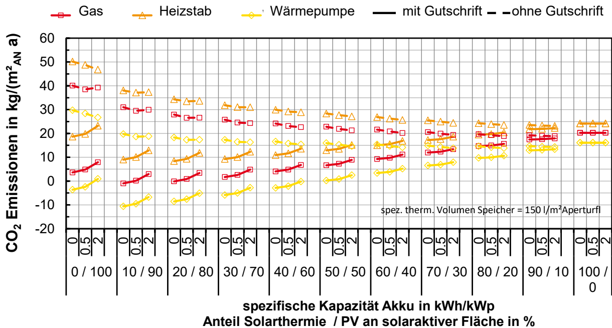
Abbildung G. 31: EFH UMK: spez. CO 2 -Emissionen in Abhängigkeit der Konzeptvariante bezogen auf den Lebenszyklus
