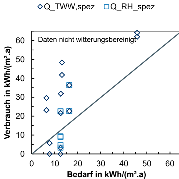
Abbildung 7-2: Gegenüberstellung des Trinkwarmwasserverbrauches sowie des Raumwärmeverbrauches mit den in der Planung hinterlegten Größen, Messzeitraum 16/17 und 17/18
