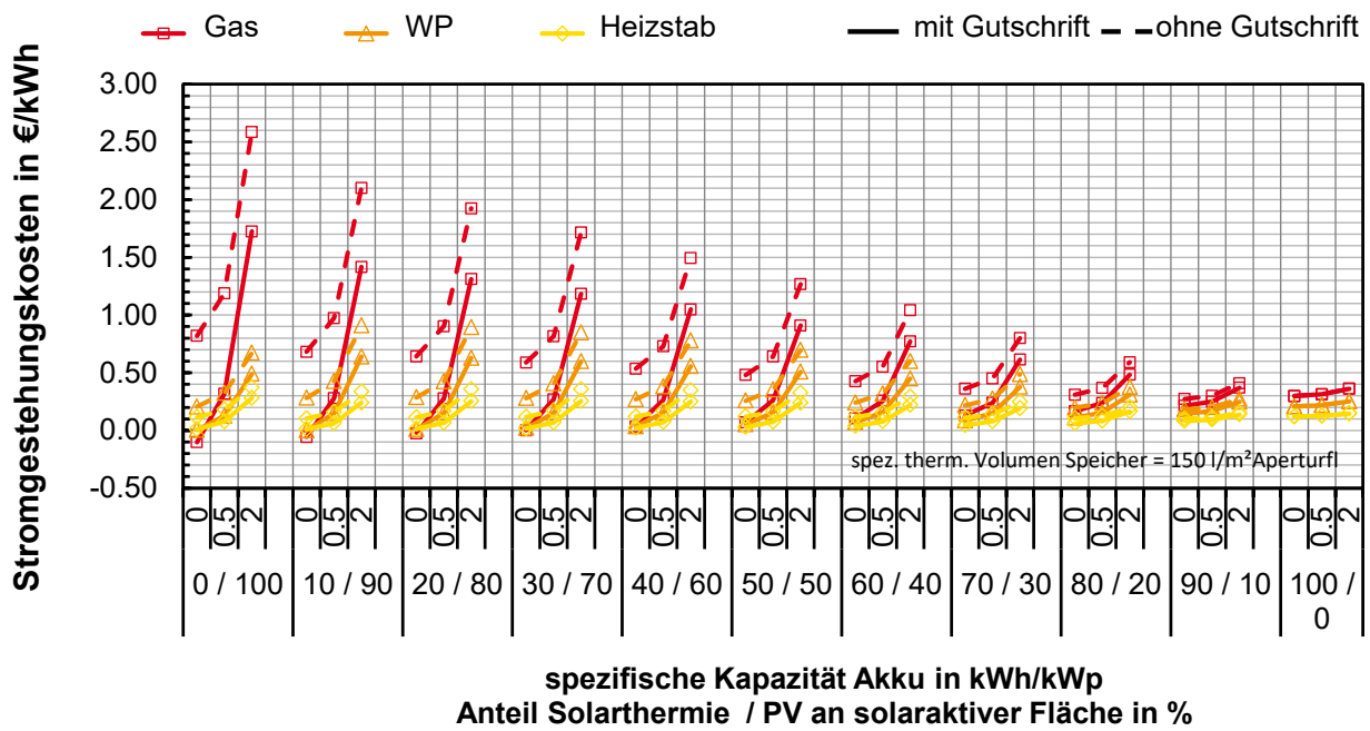
Abbildung G. 57: EFH KAT: Gestehungskosten Strom in Abhängigkeit der Konzeptvariante
