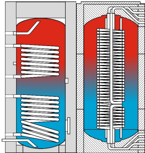
Abbildung B. 5 Schematische Darstellung zweier Warmwasserspeicher; links ein Trinkwasserspeicher mit Wärmeübertragern für Nachheizung (oben) und Solaranlage (unten), rechts ein Kombispeicher mit Wärmeübertragern zur Trinkwassererwärmung (durchgängig von unten nach oben) und Solarenergie (unten), die Nachheizung erfolgt direkt.
