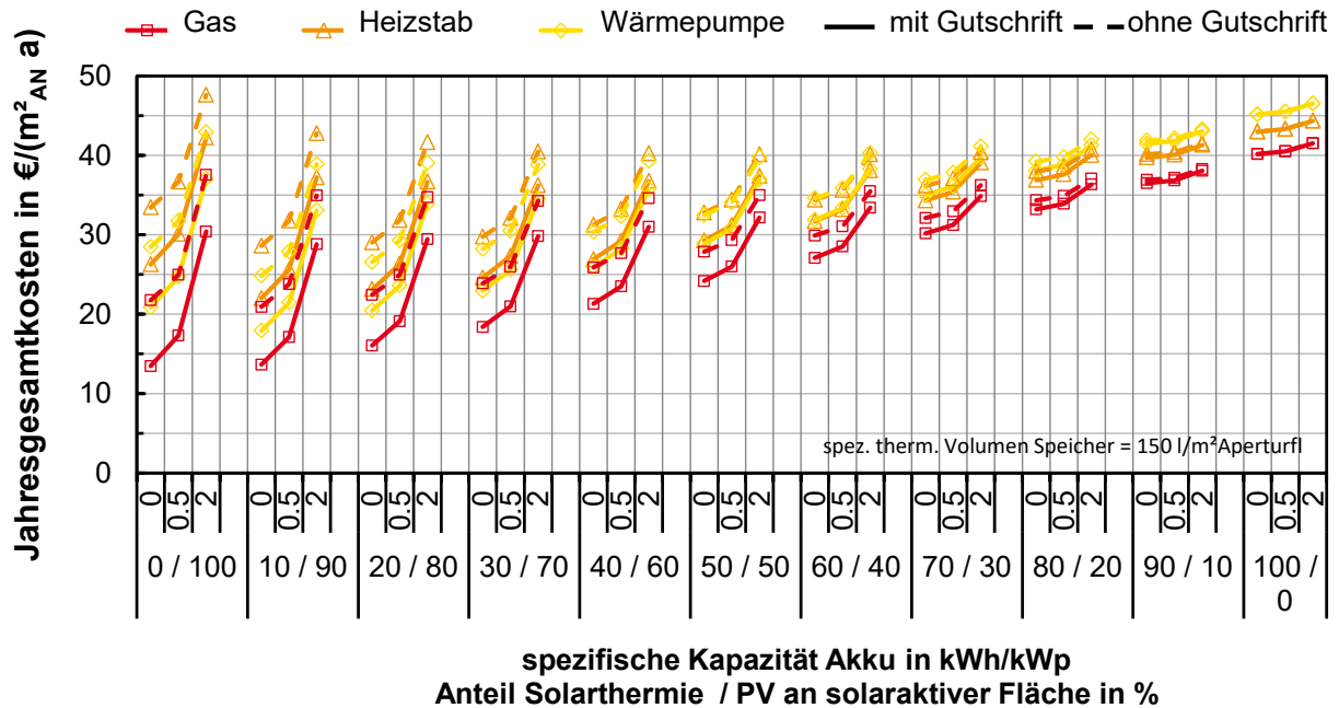
Abbildung G. 48: EFH UMK: spez. Jahresgesamtkosten in Abhängigkeit der Konzeptvariante
