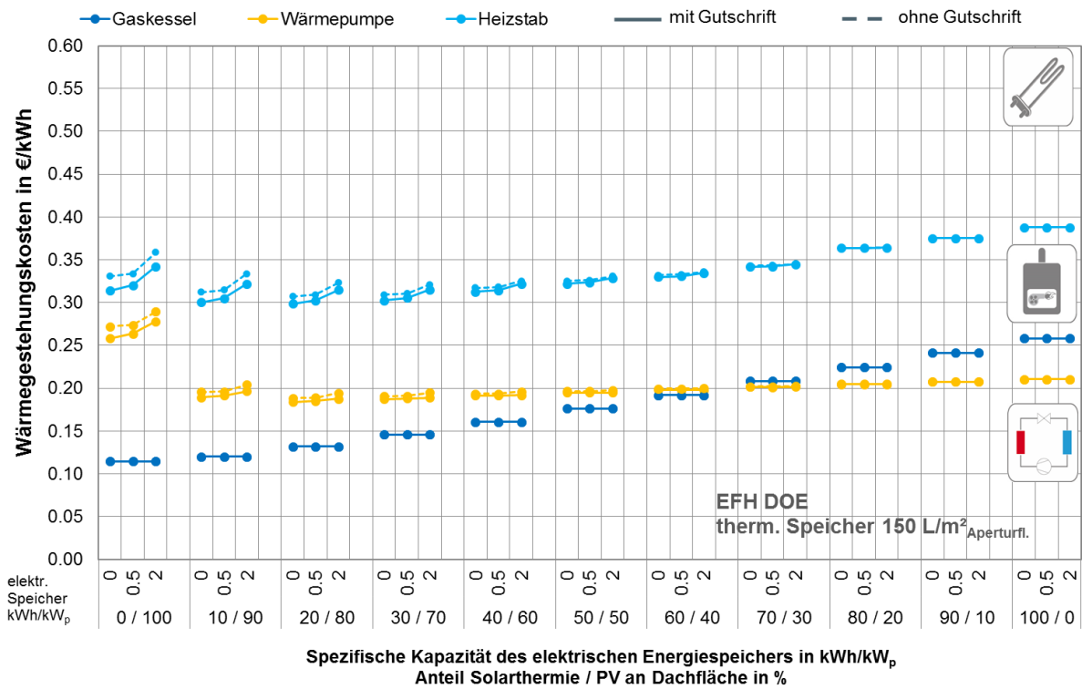
Abbildung G. 53: EFH DOE: Gestehungskosten Wärme in Abhängigkeit der Konzeptvariante
