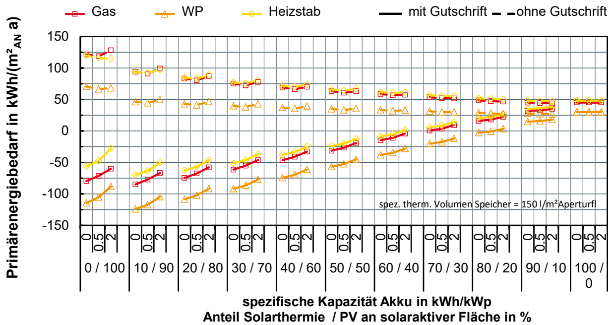
Abbildung G. 38: EFH KAT: spez. Primärenergiebedarf in Abhängigkeit der Konzeptvariante bezogen auf den Lebenszyklus
