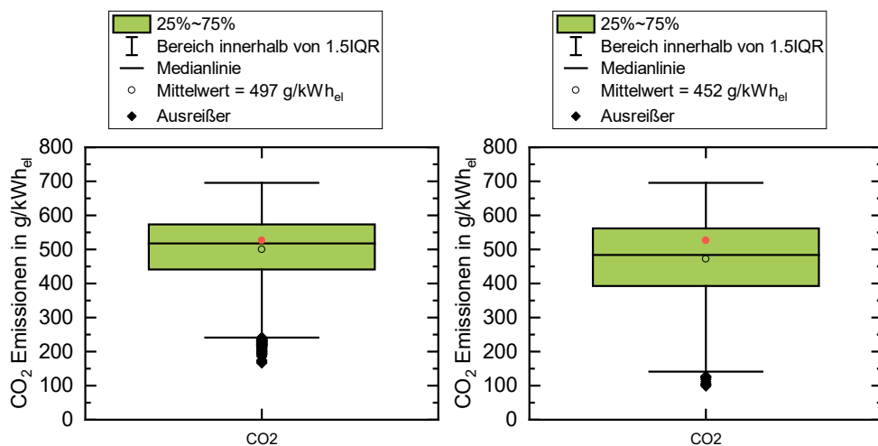
Abbildung 7-21: Boxplot über die variablen CO 2 Faktoren für den Zeitraum 01.07.2016 – 30.06.2017 (links) und 01.07.2017 – 30.06.2018 (rechts) im Vergleich mit dem konstanten Faktor von 527 g/kWh nach GEMIS (roter Punkt)
