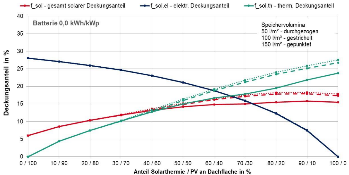
Abbildung 4-3: Einfluss des Verhältnisses von thermischer Speichergöße zur Aperturfläche auf den solaren Deckungsanteil beim MFH
