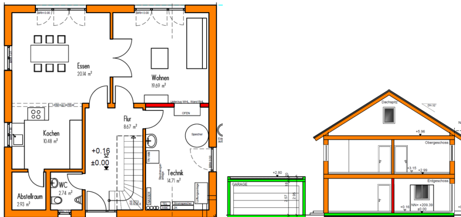
Abbildung 6-53: Grundriss und Längsschnitt des Gebäudes und der daneben befindlichen Garage. (Bauteile aus Beton sind grün, gemauerte Teile in rot und andere Materialien in orange dargestellt).
