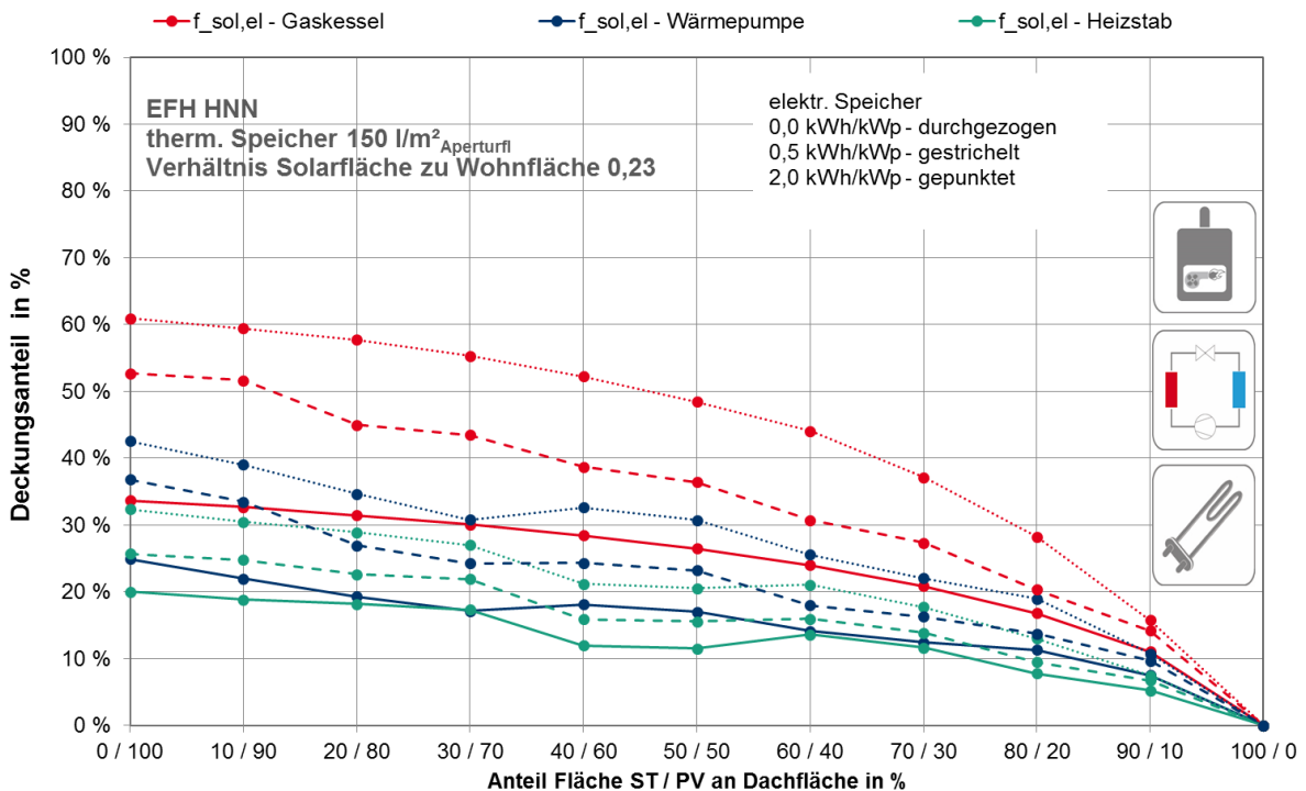
Abbildung G. 14: EFH HNN: Solar elektrische Deckungsanteile f_{sol,el} am jährlichen Stromverbrauch in Abhängigkeit der Konzeptvariante
