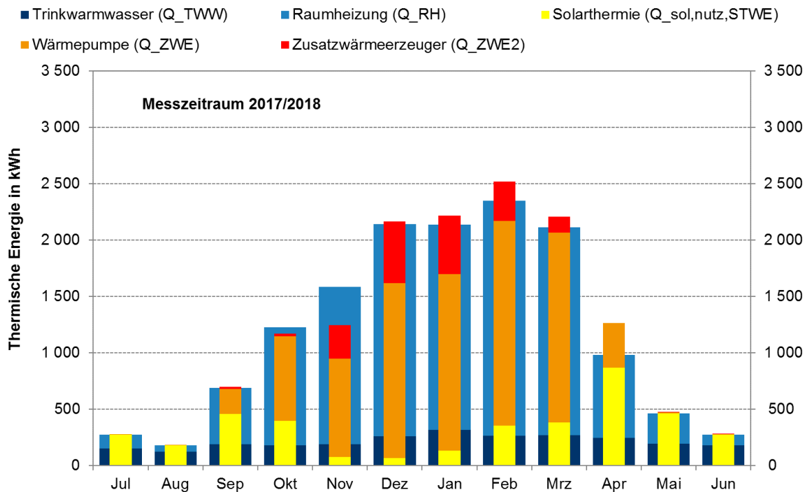
Abbildung 6-36: Monatliche Energiebilanzen für den Messzeitraum 2017/2018 des Gebäudes in Heilbronn-Neckargartach
