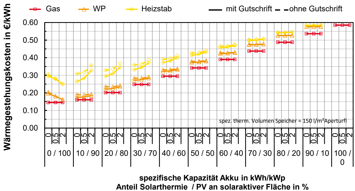
Abbildung G. 58: EFH KAT: Gestehungskosten Wärme in Abhängigkeit der Konzeptvariante
