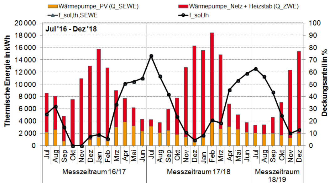
Abbildung 6-18: MFH FFM: Monatliche Wärmebereitstellung über die Wärmepumpe – Anteile regenerative Erzeugung
