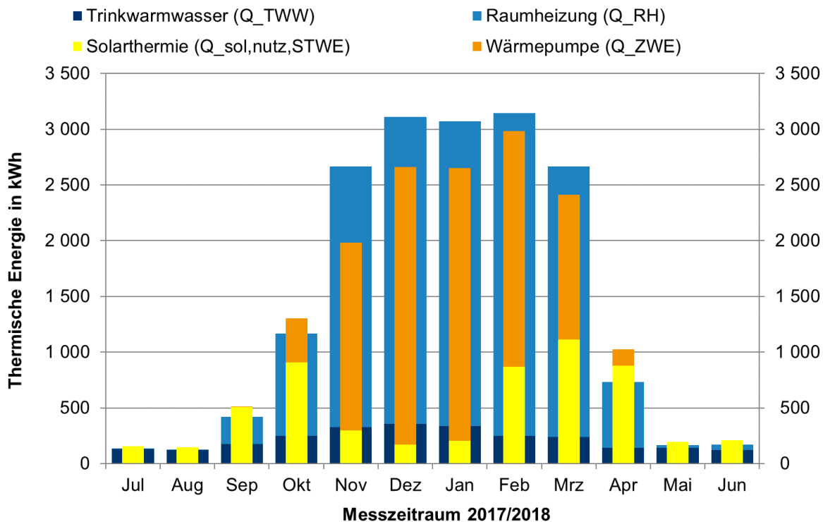
Abbildung 6-27: Monatliche Energiebilanzen für den Messzeitraum 2017/2018 des Gebäudes in Döhlau
