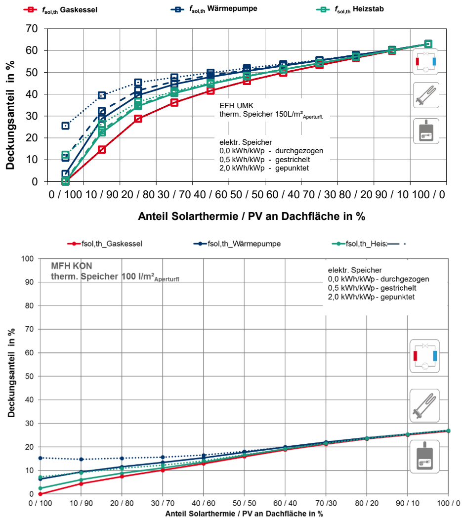
Abbildung 7-27: Vergleich der solarthermischen Deckungsanteile des EFH UMK und des MFH KON ohne und mit elektrischem Energiespeicher mit 2.0 kWh/kW p
