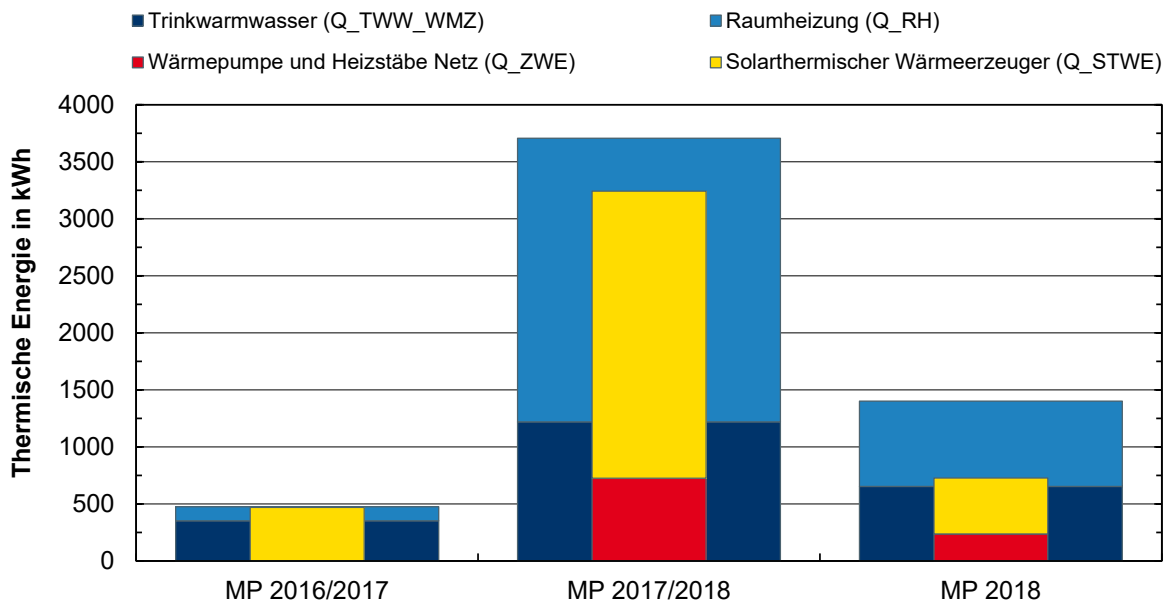
Abbildung 6-48: Jährliche Messdaten für die Wärmeversorgung
