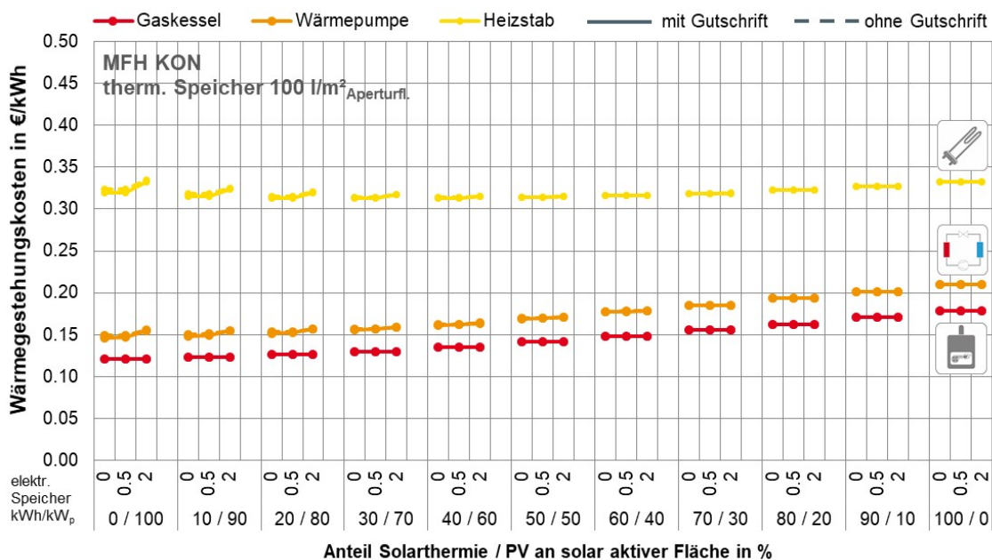
Abbildung 7-35: MFH KON: Gestehungskosten Wärme in Abhängigkeit der Konzeptvariante
