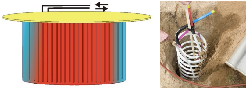
Abbildung B. 6 Schematische Darstellung eines Feststoffspeichers nach dem Prinzip der fühlbaren Wärme in der Ausführung als Erdsondenwärmespeicher (links), Erdsonde in Helix-Ausführung während des Einbringens ins Erdreich (rechts)
