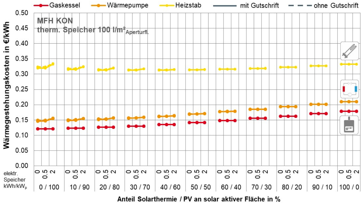
Abbildung G. 49: MFH KON: Gestehungskosten Wärme in Abhängigkeit der Konzeptvariante
