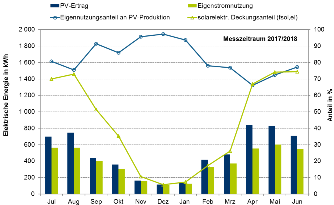
Abbildung 6-32: Monatlicher PV-Ertrag und sowie der Eigennutzungsanteil und der solarelektrische Deckungsanteil für den Messzeitraum 2017/2018 des Gebäudes in Döhlau
