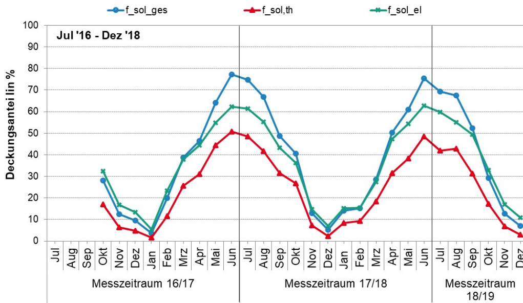
Abbildung 6-12: MFH KON: Monatliche solare Deckungsanteile
