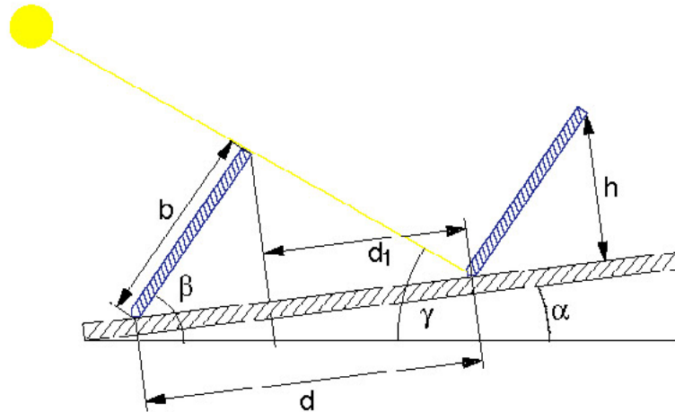
Abbildung 5-7: Schematische Darstellung der Aufstellung der Photovoltaikmodule
