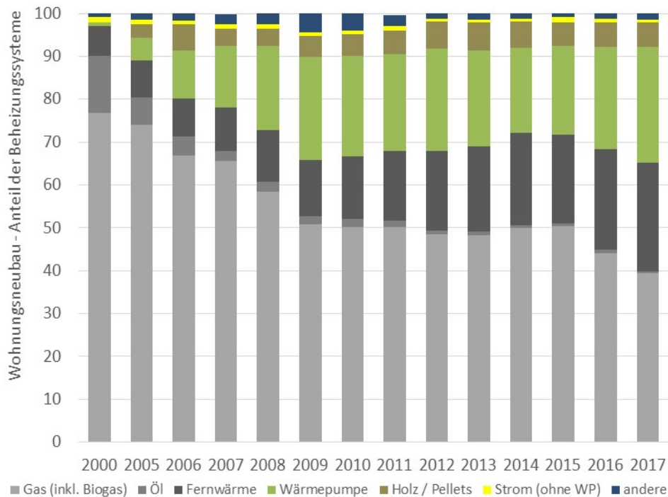
Abbildung 3-1: Beheizungsstruktur im Wohnungsneubau in Deutschland in den Jahren 2000 bis 2017 [BDEW]
