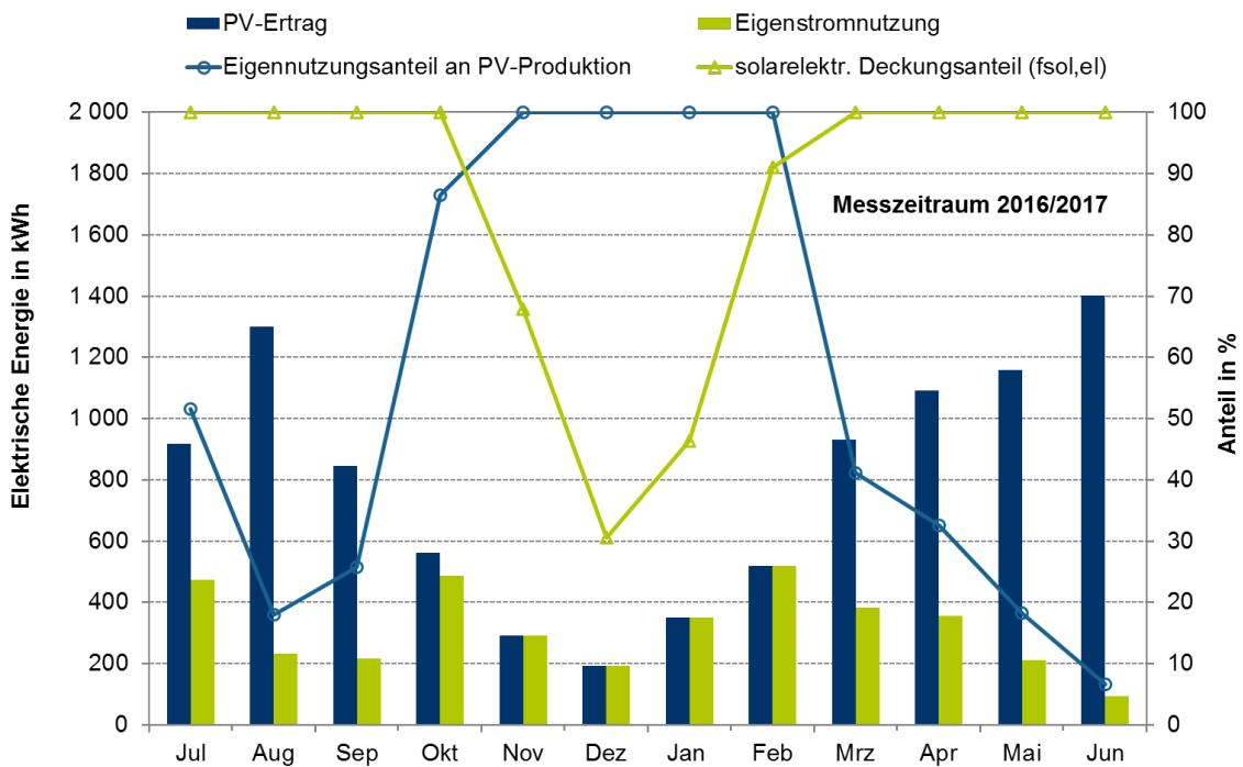
Abbildung 6-40: Monatlicher PV-Ertrag und sowie der Eigennutzungsanteil und der solarelektrische Deckungsanteil für den Messzeitraum 2016/2017 des Gebäudes HNN
