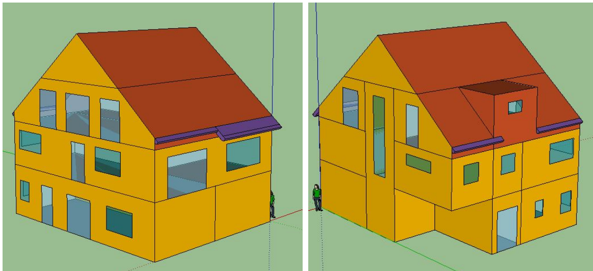
Abbildung 5-1: Zeichnung des Gebäudemodells HNN, Ansichten Süd-West (links) und Nord-Ost (rechts)
