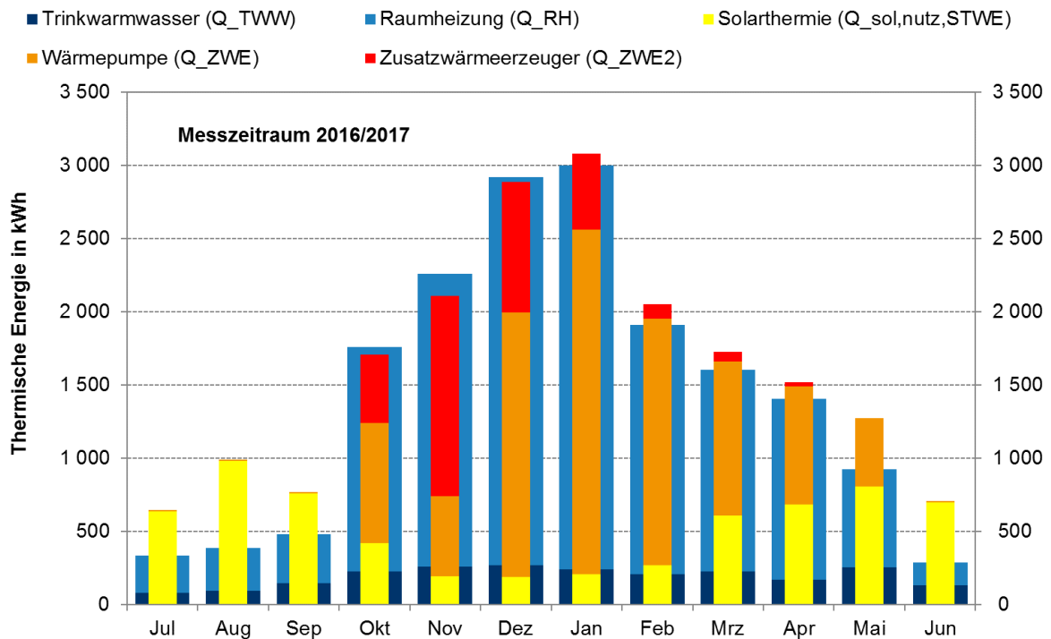
Abbildung 6-35: Monatliche Energiebilanzen für den Messzeitraum 2016/2017 des Gebäudes in Heilbronn-Neckargartach
