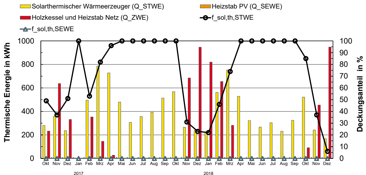
Abbildung 6-57: Erzeugte Wärmemengen der einzelnen Wärmeerzeuger sowie die daraus resultierenden Deckungsbeiträge über die gesamte Messperiode
