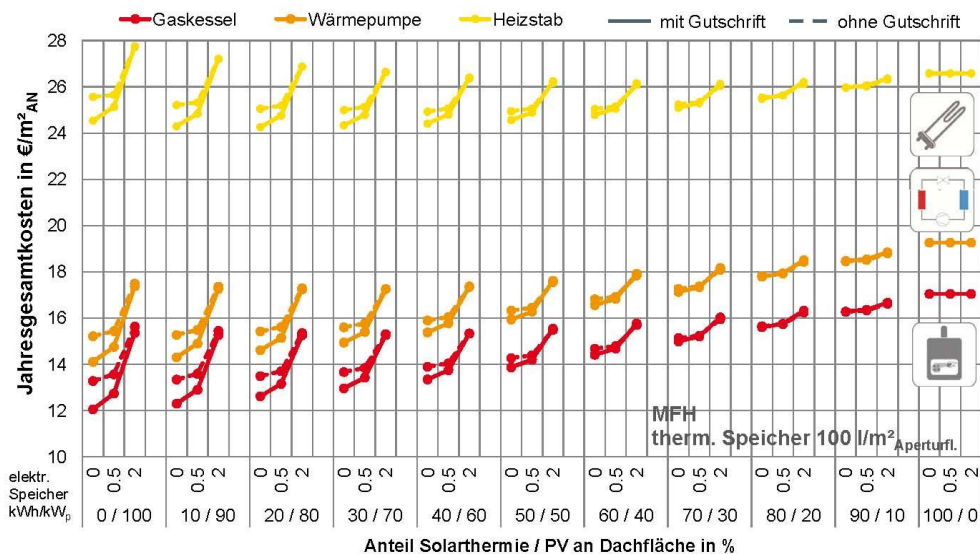
Abbildung 4-15: Arbeitsdiagramm MFH: spez. Jahresgesamtkosten in Abhängigkeit der Konzeptvariante
