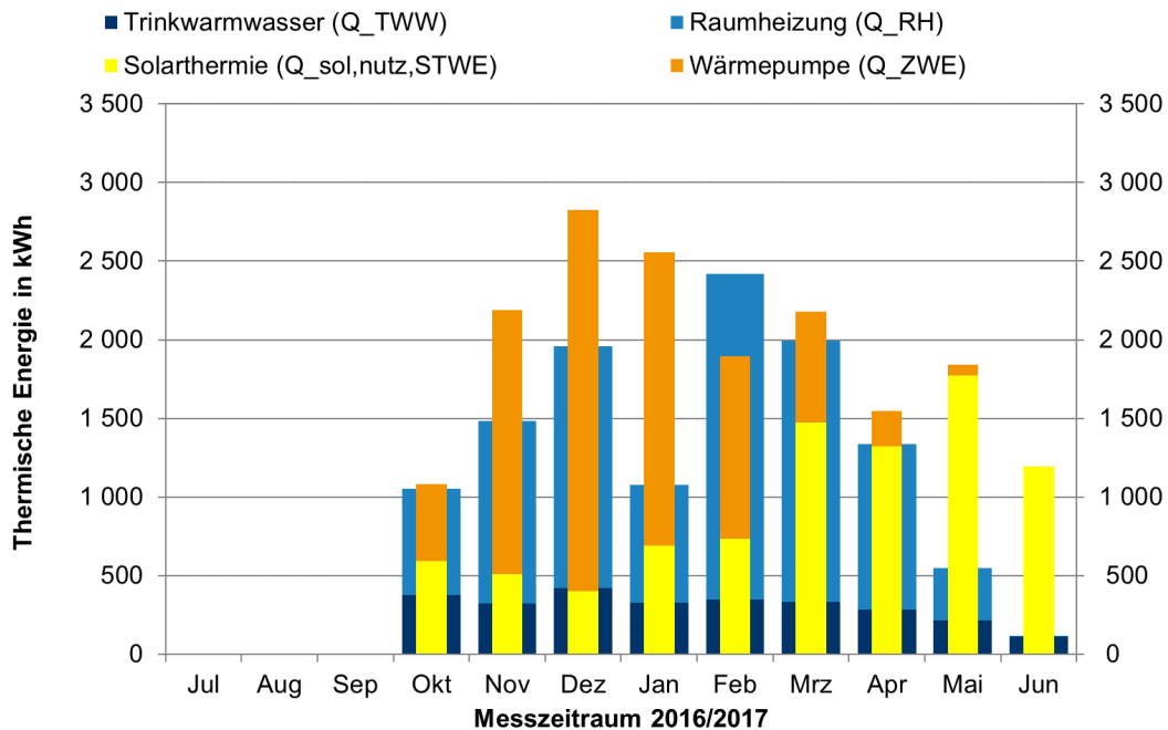
Abbildung 6-26: Monatliche Energiebilanzen für den Messzeitraum 2016/2017 des Gebäudes in Döhlau
