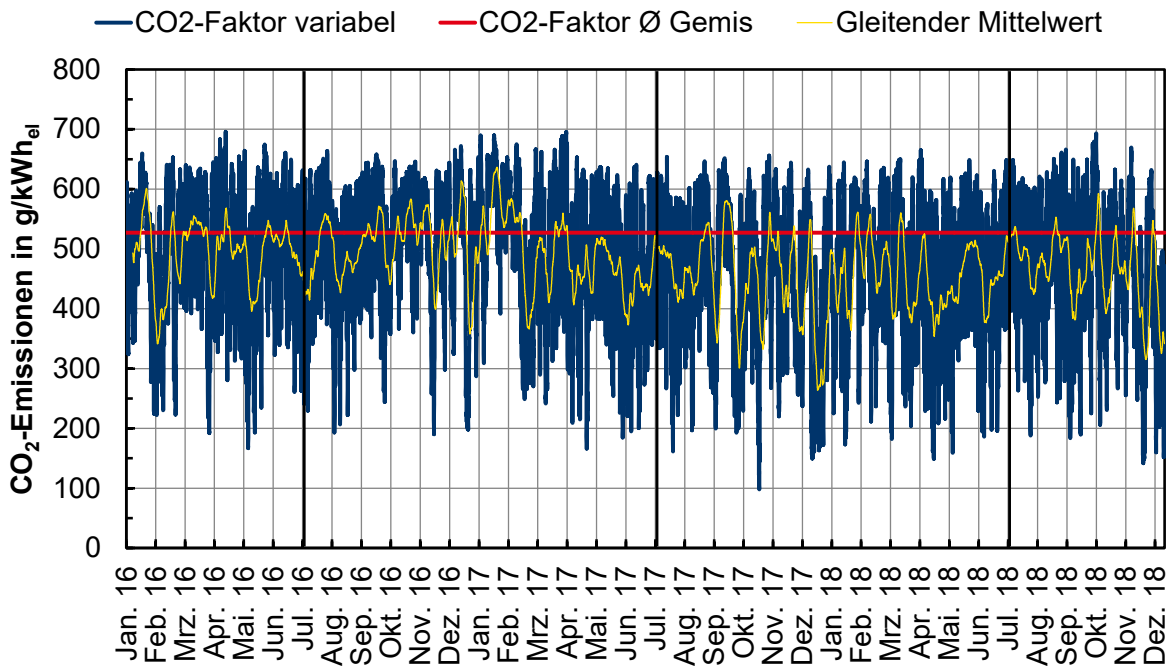
Abbildung 7-20: Vergleich der variablen CO 2 Faktoren, basierend auf aufbereiteten Daten aus den EnergyCharts [21] im Vergleich mit einem konstanten CO 2 Faktoren für die Jahre 2016 – 2018
