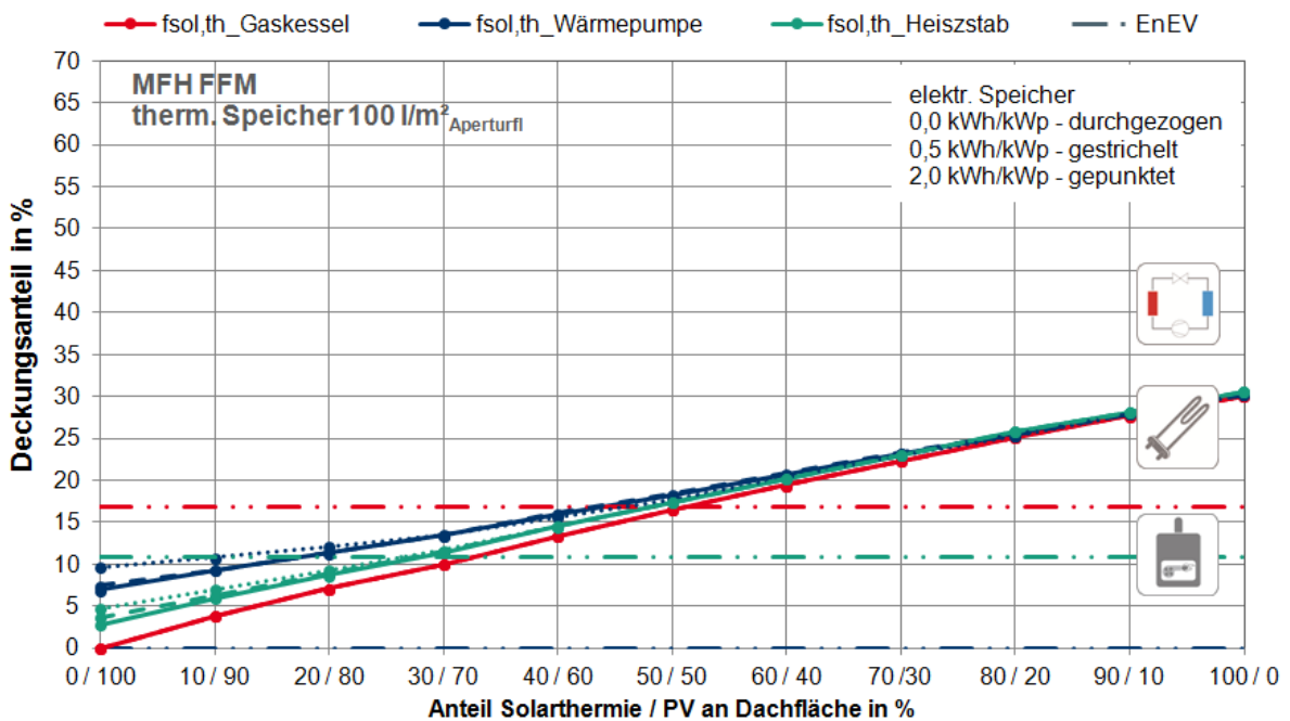
Abbildung G. 10: MFH FFM: Solar thermische Deckungsanteile f_{sol,th} an der Wärmebereitstellung in Abhängigkeit der Konzeptvariante
