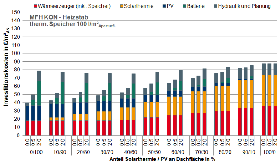
Abbildung G. 41: MFH KON: spez. Investitionskosten in Abhängigkeit der Konzeptvariante – Gaskessel oben, Wärmepumpe Mitte und Heizstab unten
