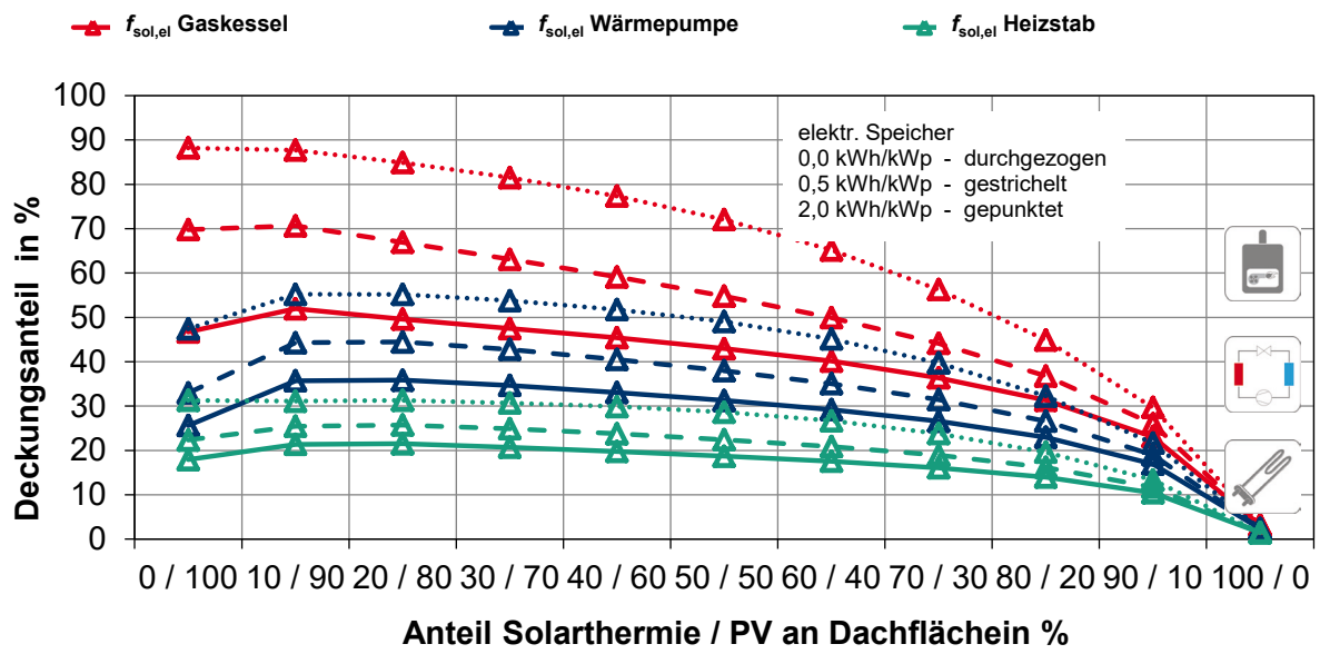
Abbildung G. 23: EFH UMK: Solar elektrische Deckungsanteile f_{sol,el} am jährlichen Stromverbrauch in Abhängigkeit der Konzeptvariante
