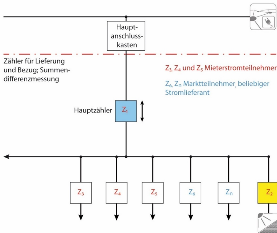
Abbildung 9-3: Messprinzip Summenzählermodell (nach [48])
