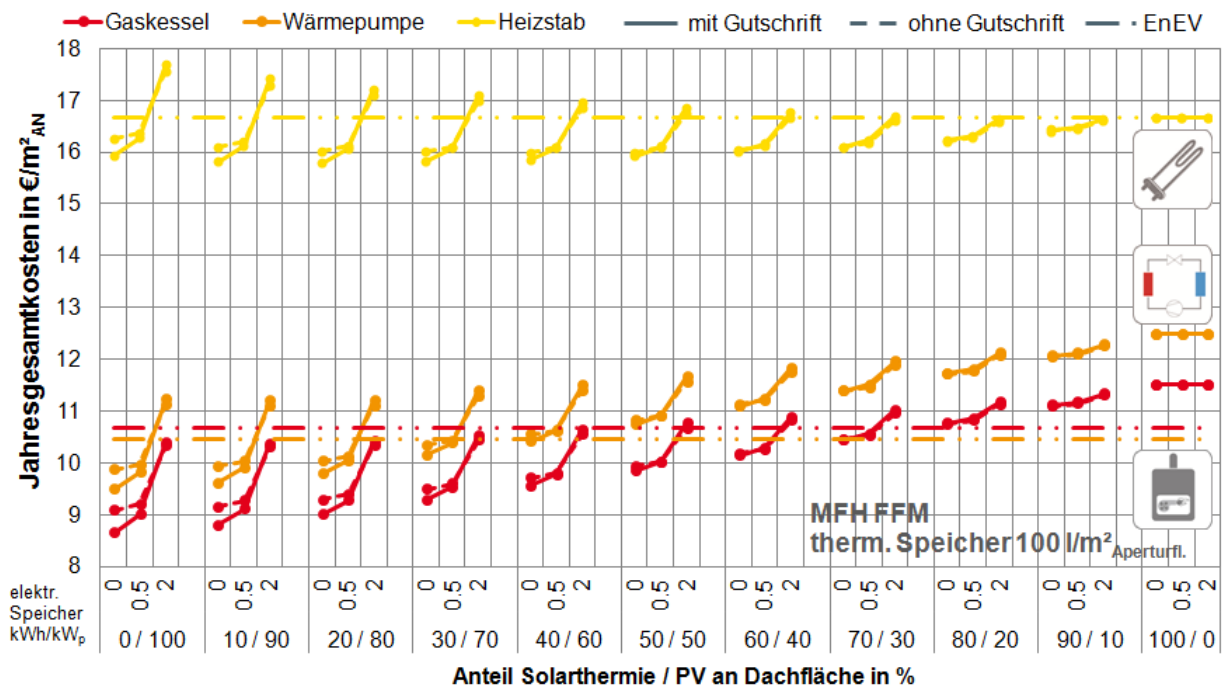
Abbildung G. 42: MFH FFM: spez. Jahresgesamtkosten in Abhängigkeit der Konzeptvariante
