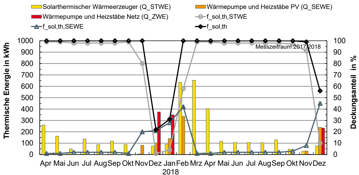
Abbildung 6-46: Erzeugte Wärmemengen der einzelnen Wärmeerzeuger sowie die daraus resultierenden Deckungsbeiträge über die gesamte Messperiode
