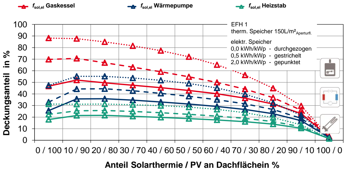
Abbildung 4-8: Arbeitsdiagramm EFH: Solar elektrische Deckungsanteile f_{sol,el} am jährlichen Stromverbrauch in Abhängigkeit der Konzeptvariante
