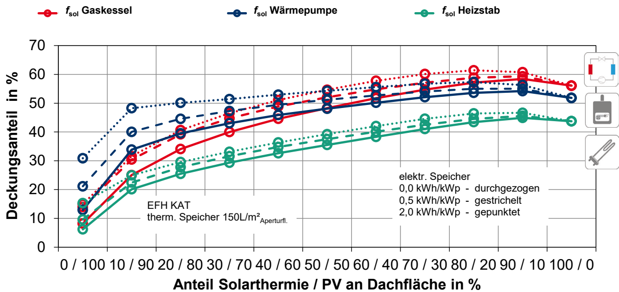
Abbildung G. 18: EFH KAT: Gesamt solarer Deckungsanteile: f_{sol} am jährlichen Energieverbrauch in Abhängigkeit der Konzeptvariante
