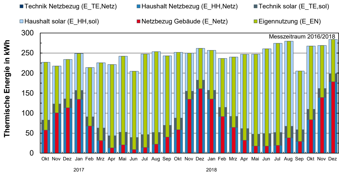
Abbildung 6-61: Monatliche Messdaten für die Elektrizitätsversorgung aus dem gesamten messtechnisch untersuchten Zeitraum
