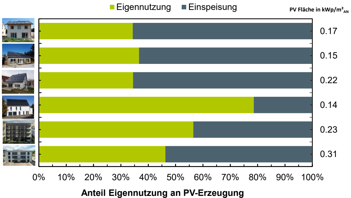
Abbildung 7-8: Gegenüberstellung der Messdaten aus dem Messzeitraum 2016/2017 von eigen genutzter Energie aus der PV Anlage E_{EN} sowie dem eingespeisten Anteil. Weiterhin ist die installierte Leistung der PV Anlagen in kW p über die Gebäudenutzfläche A_N dargestellt.
