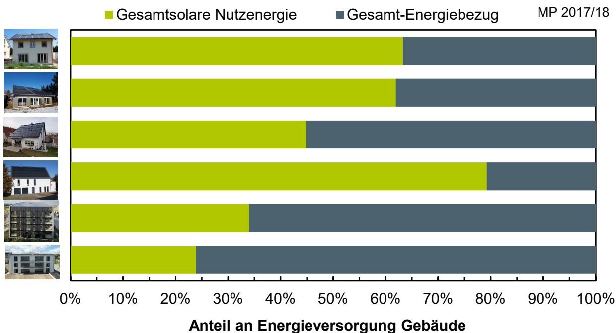
Abbildung 7-14: Aufteilung der Energieversorgung der Gebäude mit elektrischer Energie und Wärme in solar bereitgestellte Energie und extern bezogene Energie für den Messzeitraum 2017/2018.
