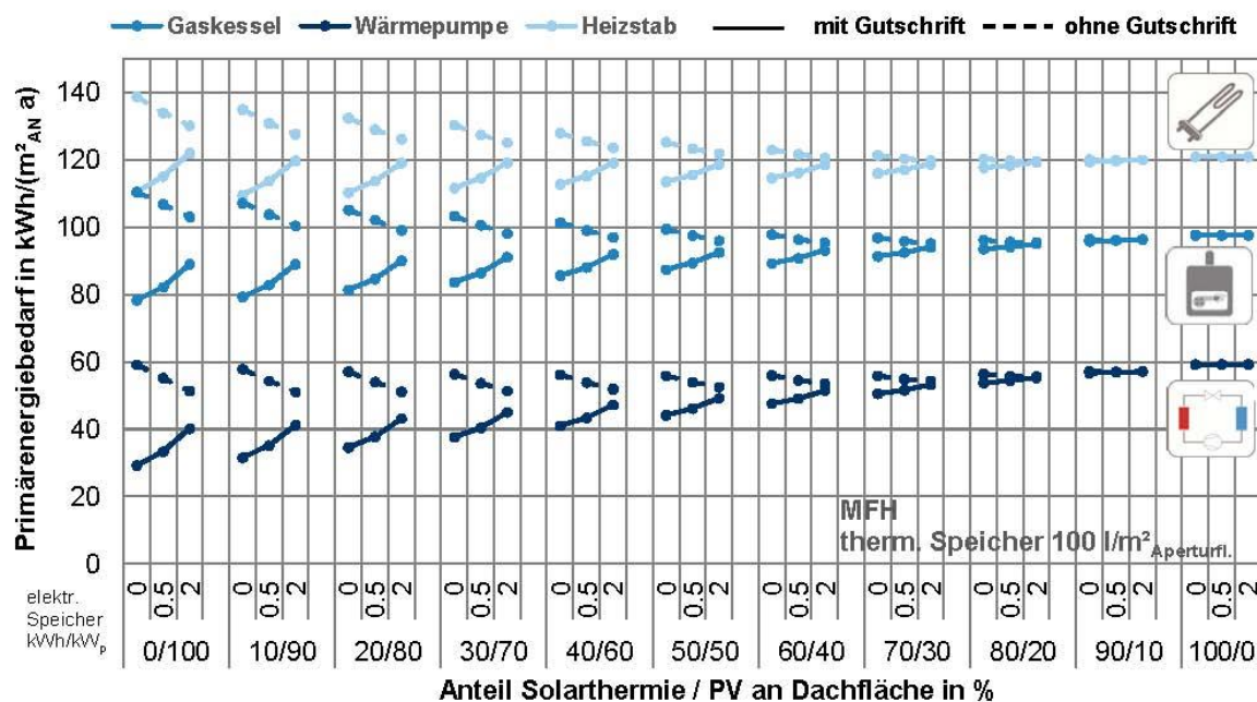
Abbildung 4-13: Arbeitsdiagramm MFH: Primärenergiebedarf in Abhängigkeit der Konzeptvariante bezogen auf den Lebenszyklus mit einem
