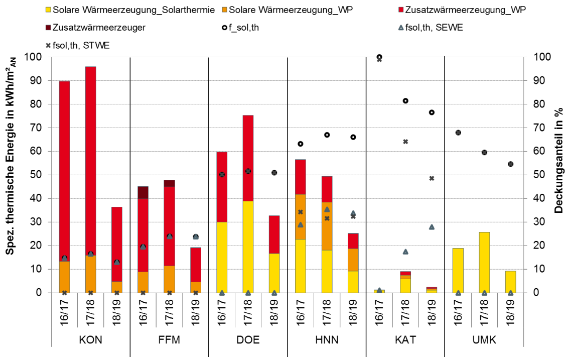
Abbildung 7-3: Anteile der solaren und konventionell bereit gestellten Wärmeversorgung sowie die Deckungsanteile des solarthermischen Wärmeerzeugers f_{\text{sol,th,STWE}} und des solarelektrischen Wärmeerzeugers f_{\text{sol,th,SEWE}} sowie der solarthermische Deckungsanteil f_{\text{sol,th}} als Summe dieser beiden Anteile
