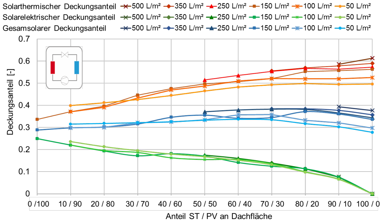
Abbildung G. 4: Solare Deckungsanteile für das EFH in HNN in Abhängigkeit der thermischen Speichergröße, Variante mit Wärmepumpe
