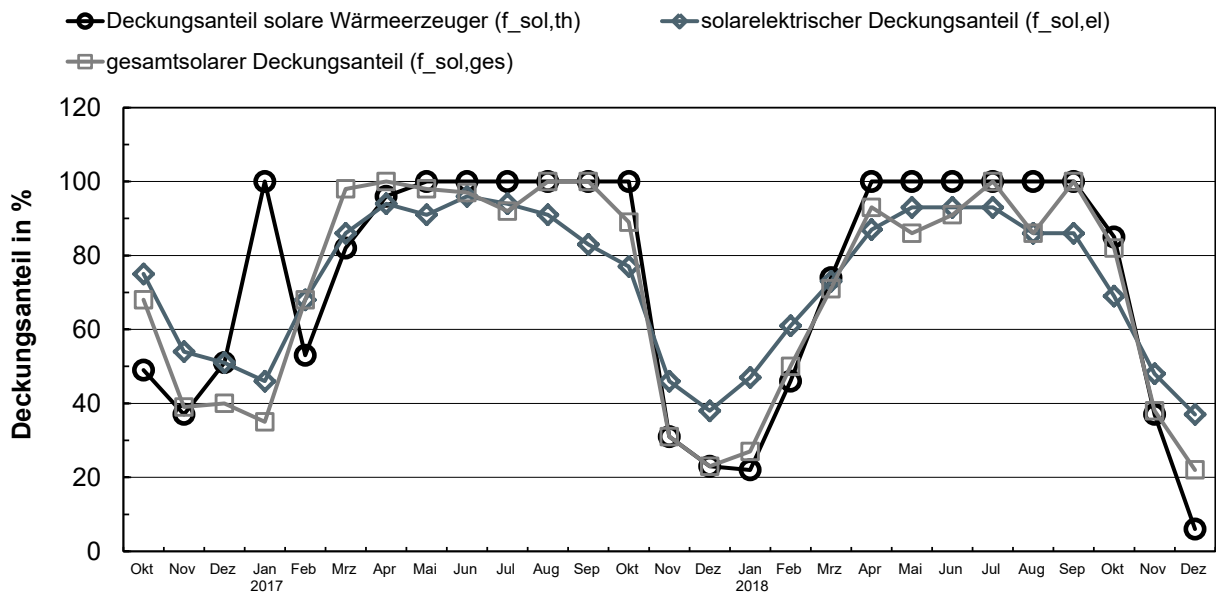
Abbildung 6-62: EFH UNK: Monatliche solare Deckungsanteile
