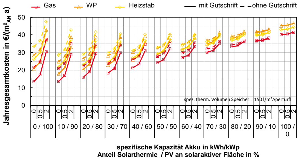
Abbildung 4-14: Arbeitsdiagramm EFH: spez. Jahresgesamtkosten in Abhängigkeit der Konzeptvariante
