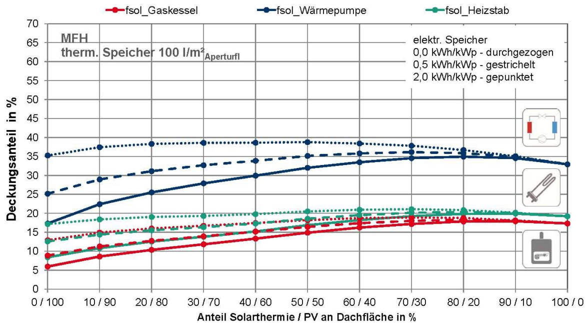
Abbildung 4-5: Arbeitsdiagramm MFH: Gesamt solarer Deckungsanteile: f_{sol} am jährlichen Energieverbrauch in Abhängigkeit der Konzeptvariante
