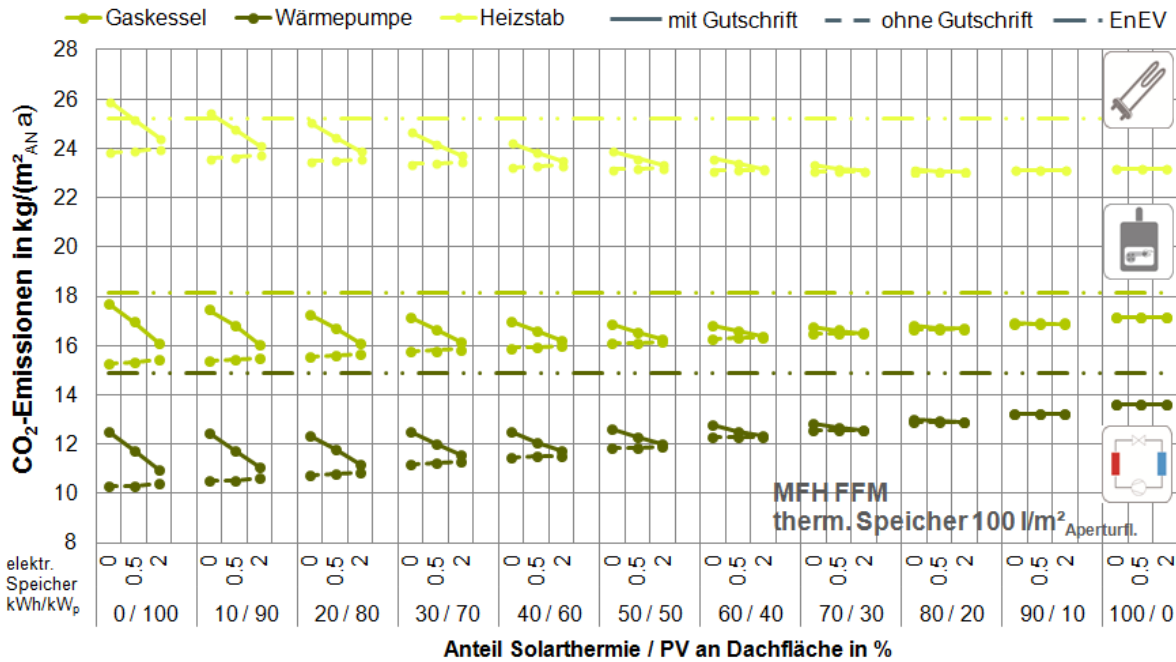
Abbildung G. 26: MFH FFM: spez. CO 2 -Emissionen in Abhängigkeit der Konzeptvariante während des Betriebes
