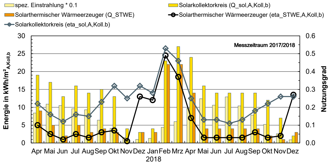
Abbildung 6-44: Aperturflächenspezifische Einstrahlung sowie die im Kollektorkreis erzeugte Wärme bezüglich dem tatsächlich nutzbaren solarthermischen Ertrag und den daraus resultierenden Nutzungsgraden für den Kollektorkreis und den solarthermischen Wärmereizger.
