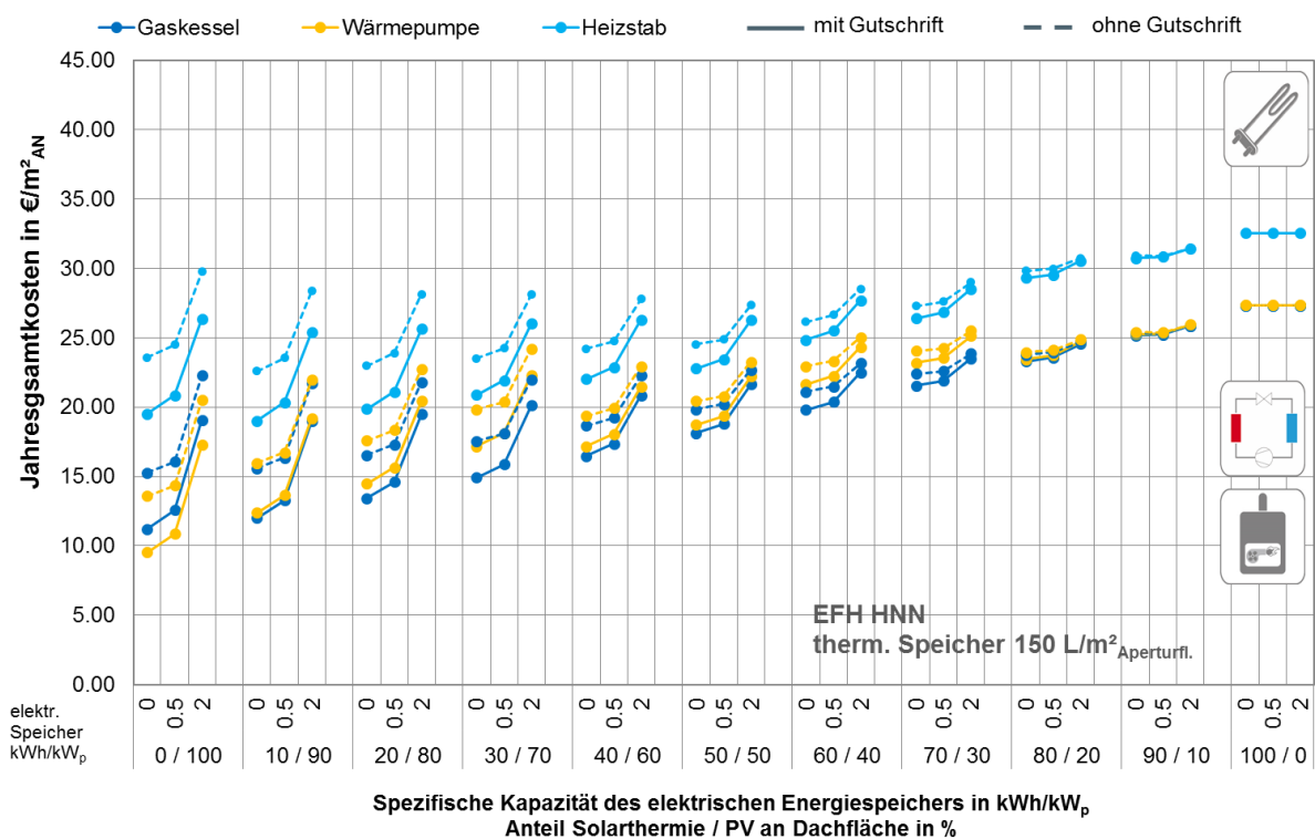
Abbildung G. 46: EFH HNN: spez. Jahresgesamtkosten in Abhängigkeit der Konzeptvariante
