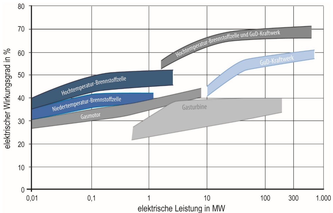
Abbildung A. 27: Elektrische Wirkungsgrade unterschiedlicher Technologien zur Stromerzeugung
