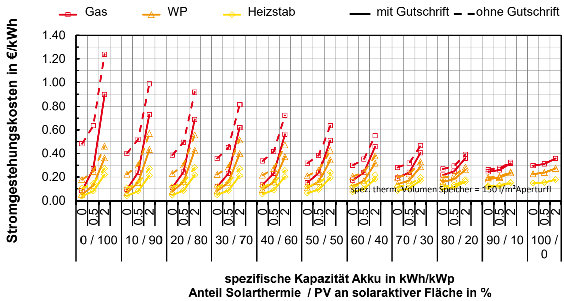
Abbildung 7-38: EFH UMK: Gestehungskosten Strom in Abhängigkeit der Konzeptvariante
