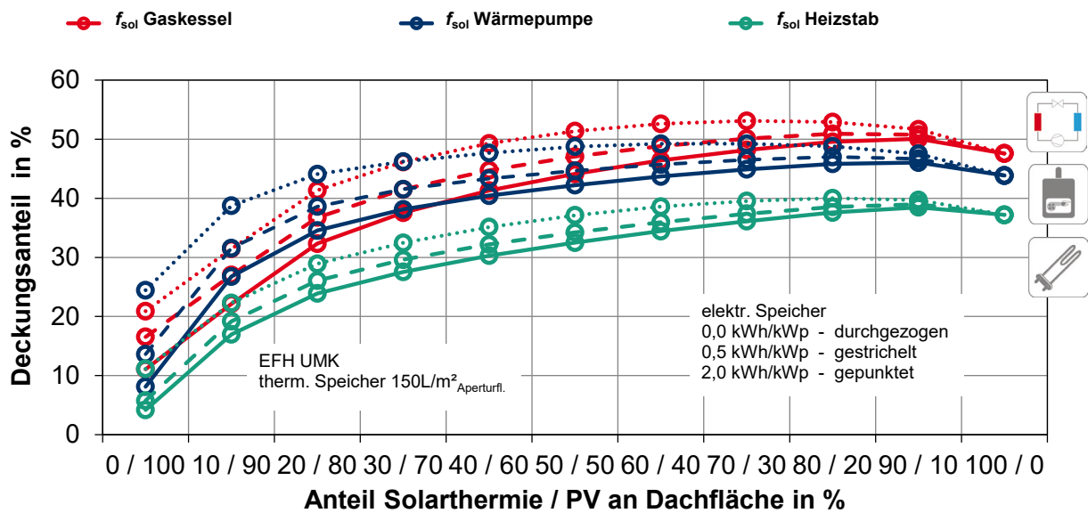
Abbildung G. 21: EFH UMK: Gesamt solarer Deckungsanteile: f_{sol} am jährlichen Energieverbrauch in Abhängigkeit der Konzeptvariante
