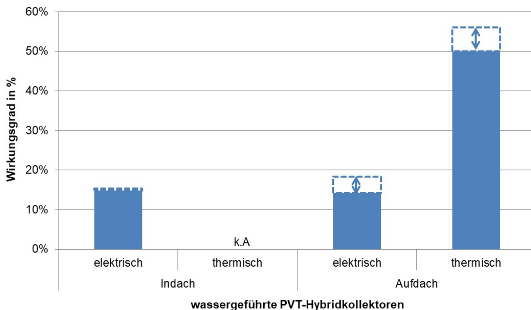
Abbildung A. 7: Elektrische und thermische Modulwirkungsgrade von wassergeführten PVT-Kollektoren
