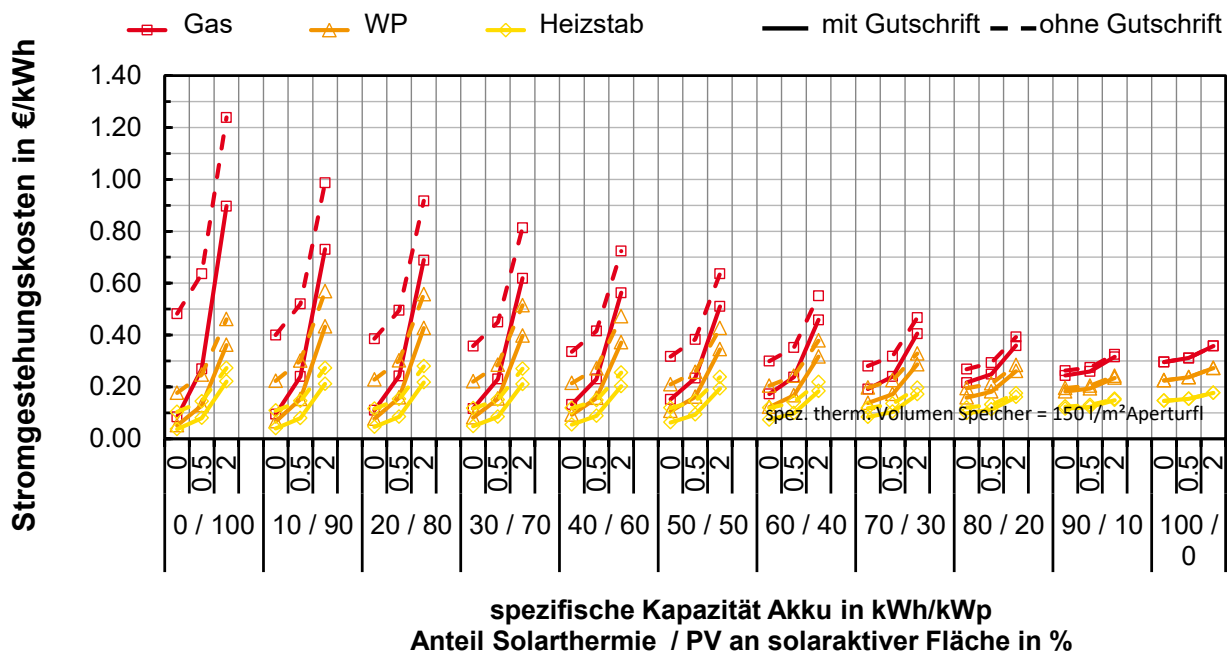
Abbildung G. 59: EFH UMK: Gestehungskosten Strom Abhängigkeit der Konzeptvariante
