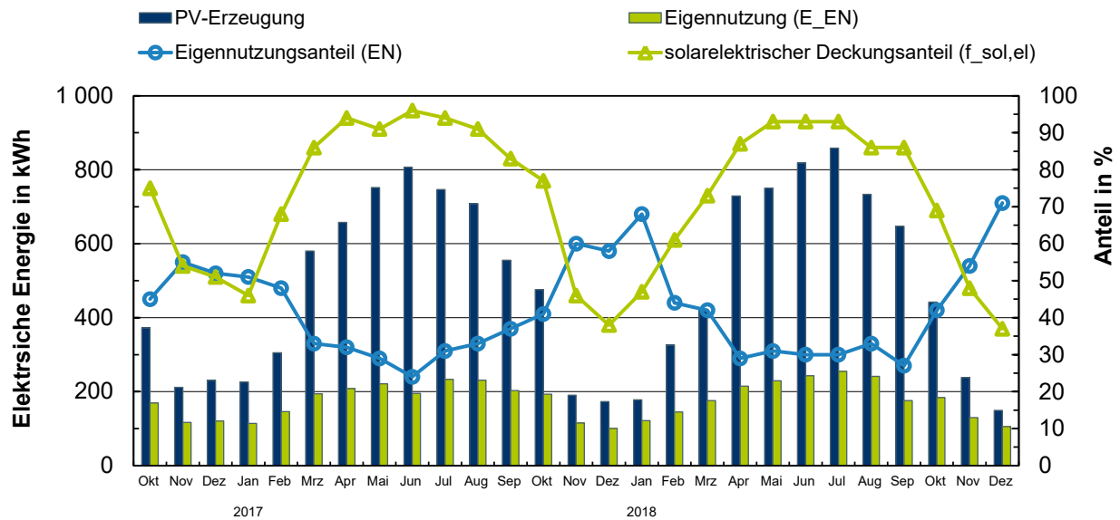
Abbildung 6-60: Monatliche Messdaten für die Elektrizitätsversorgung über den gesamten Messzeitraum
