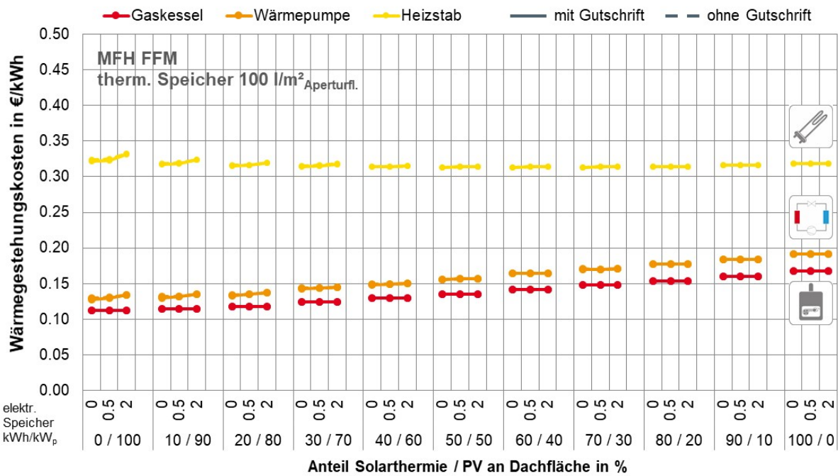
Abbildung G. 51: MFH FFM: Gestehungskosten Wärme in Abhängigkeit der Konzeptvariante
