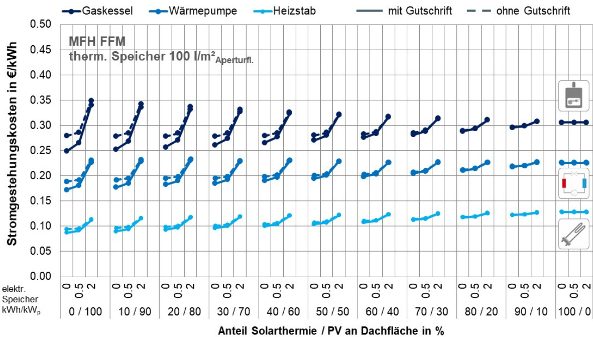
Abbildung G. 52: MFH FFM: Gestehungskosten Strom in Abhängigkeit der Konzeptvariante
