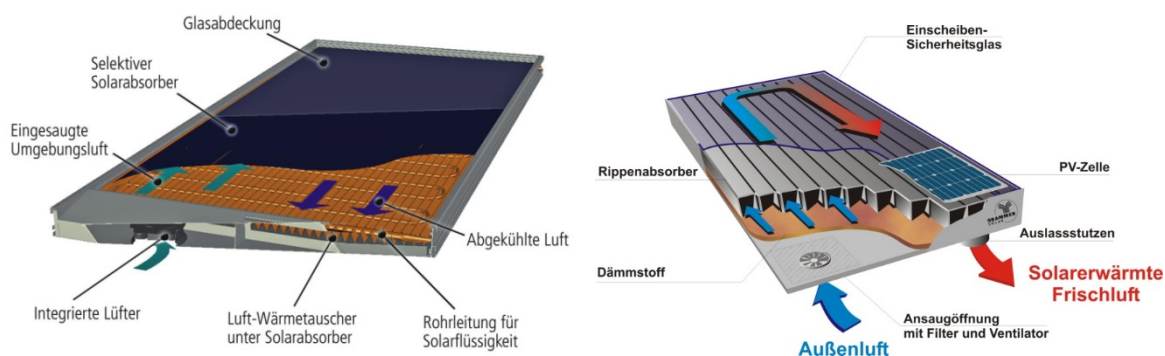
Abbildung A. 4: Beispiele für den schematischen Aufbau eines PVT-Kollektors ([Consolar Solare Energiesysteme GmbH], [GRAMMER Solar GmbH])
