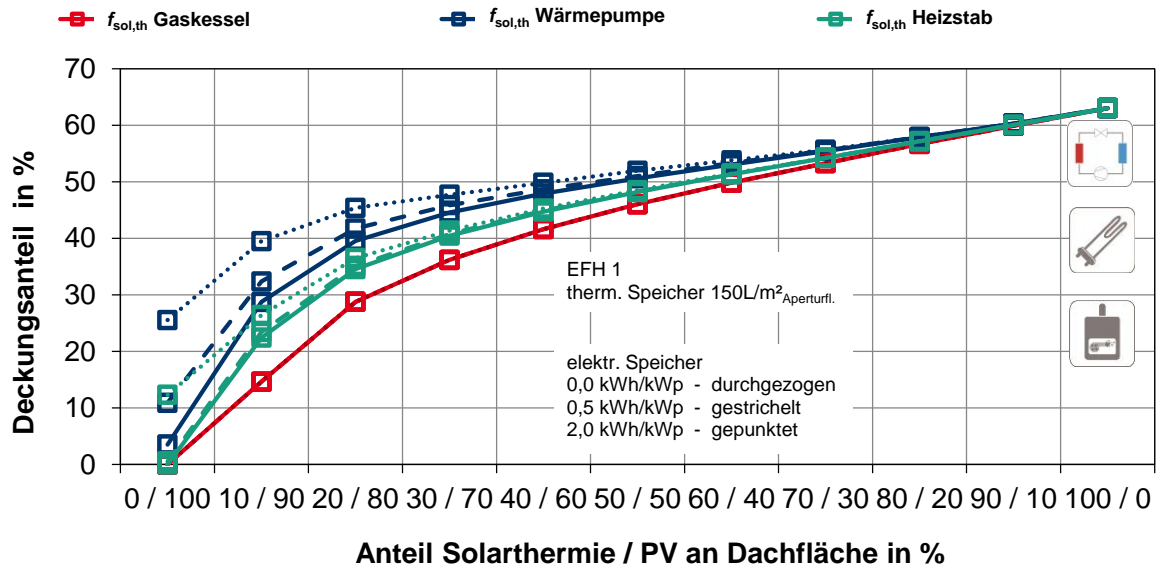
Abbildung 4-6: Arbeitsdiagramm EFH: Solar thermische Deckungsanteile f_{sol,th} an der Wärmebereitstellung in Abhängigkeit der Konzeptvariante
