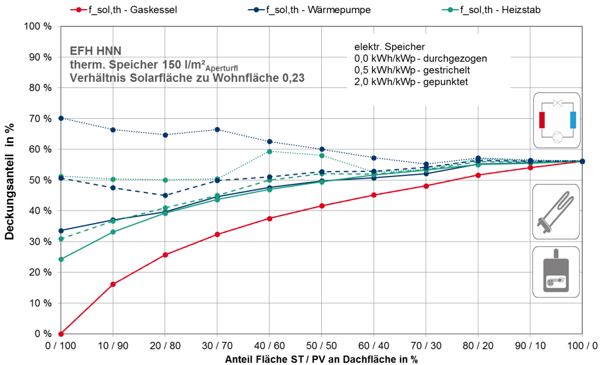
Abbildung G. 13: EFH HNN: Solar thermische Deckungsanteile f_{sol,th} an der Wärmebereitstellung in Abhängigkeit der Konzeptvariante
